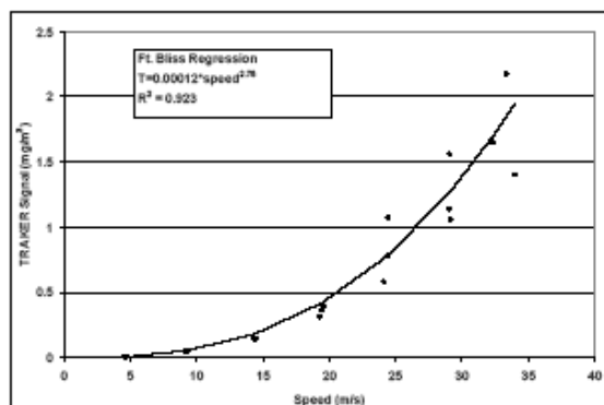
Obr. 5.8.: Vztah mezi rychlostí jízdy a množstvím zvířeného prachu [64]
