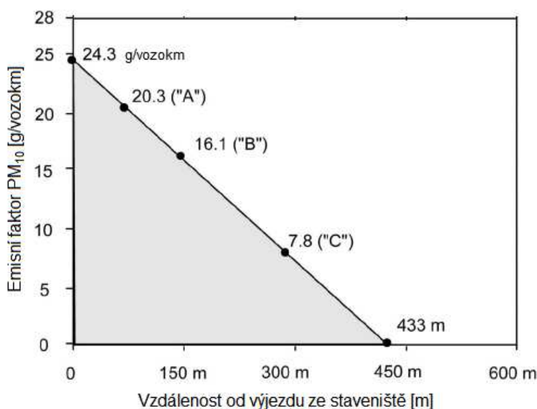
Obr. 7.1.: Emisní faktory s narůstající vzdáleností od výjezdu ze staveniště
