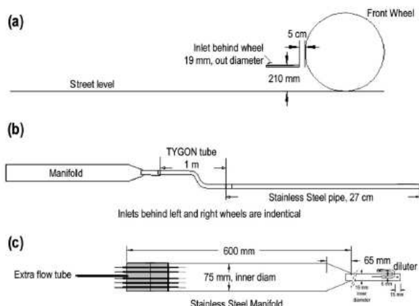
Obr. 5.5.: Vzorkovací vůz EMMA a schéma sběrného zařízení
