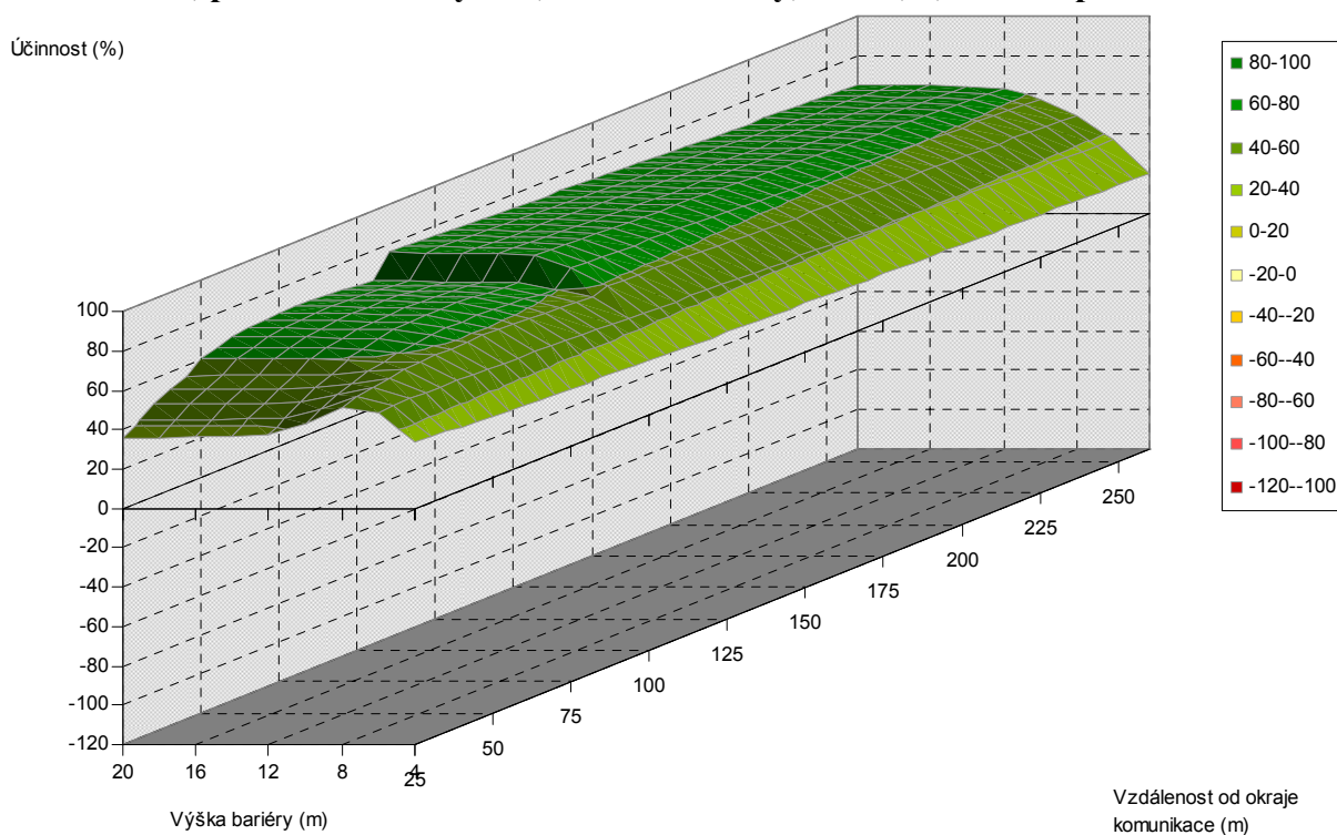
Obr. 5.68. Závislost účinnosti vegetační bariéry na výšce bariéry a vzdálenosti od komunikace, pro šířku bariéry 8 m, listnaté dřeviny, PM75, 1,5 m nad povrchem
