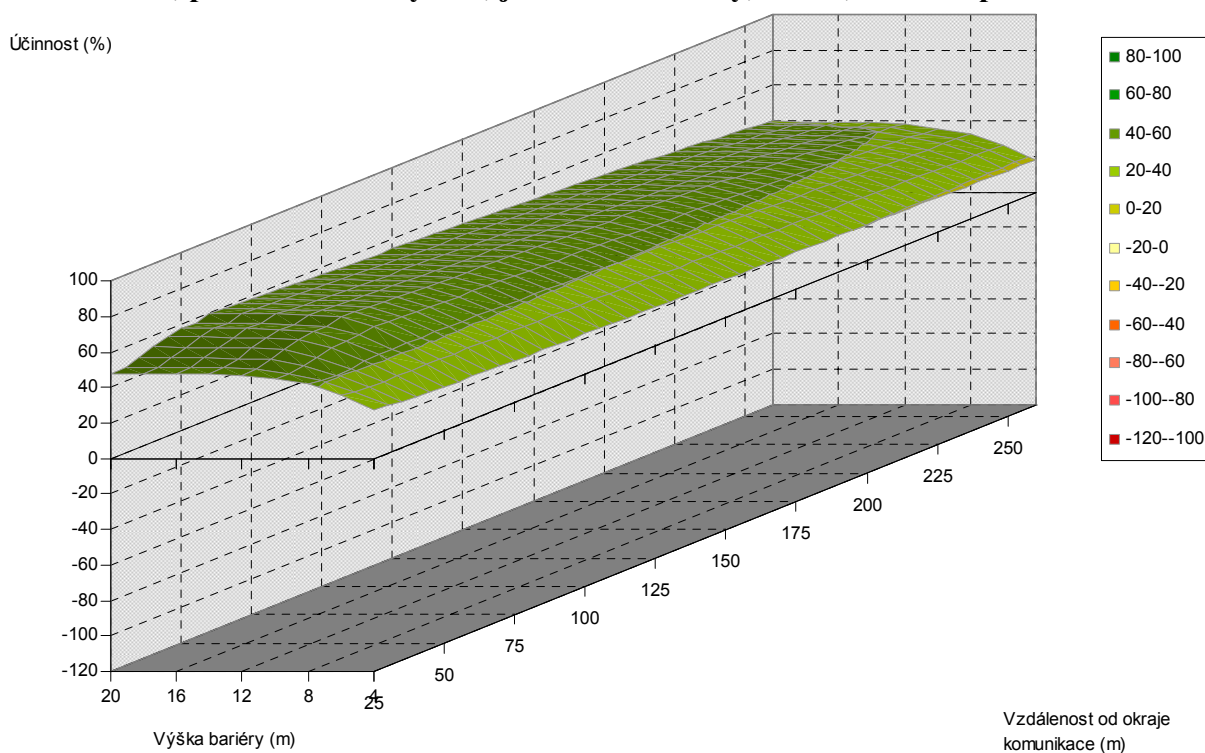
Obr. 5.100. Závislost účinnosti vegetační bariéry na výšce bariéry a vzdálenosti od komunikace, pro šířku bariéry 4 m, jehličnaté dřeviny, PM75, 3 m nad povrchem
