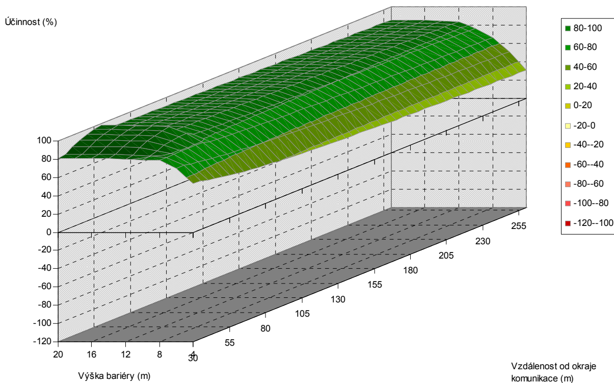
Obr. 5.72. Závislost účinnosti vegetační bariéry na výšce bariéry a vzdálenosti od komunikace, pro šířku bariéry 30 m, listnaté dřeviny, PM75, 1,5 m nad povrchem
