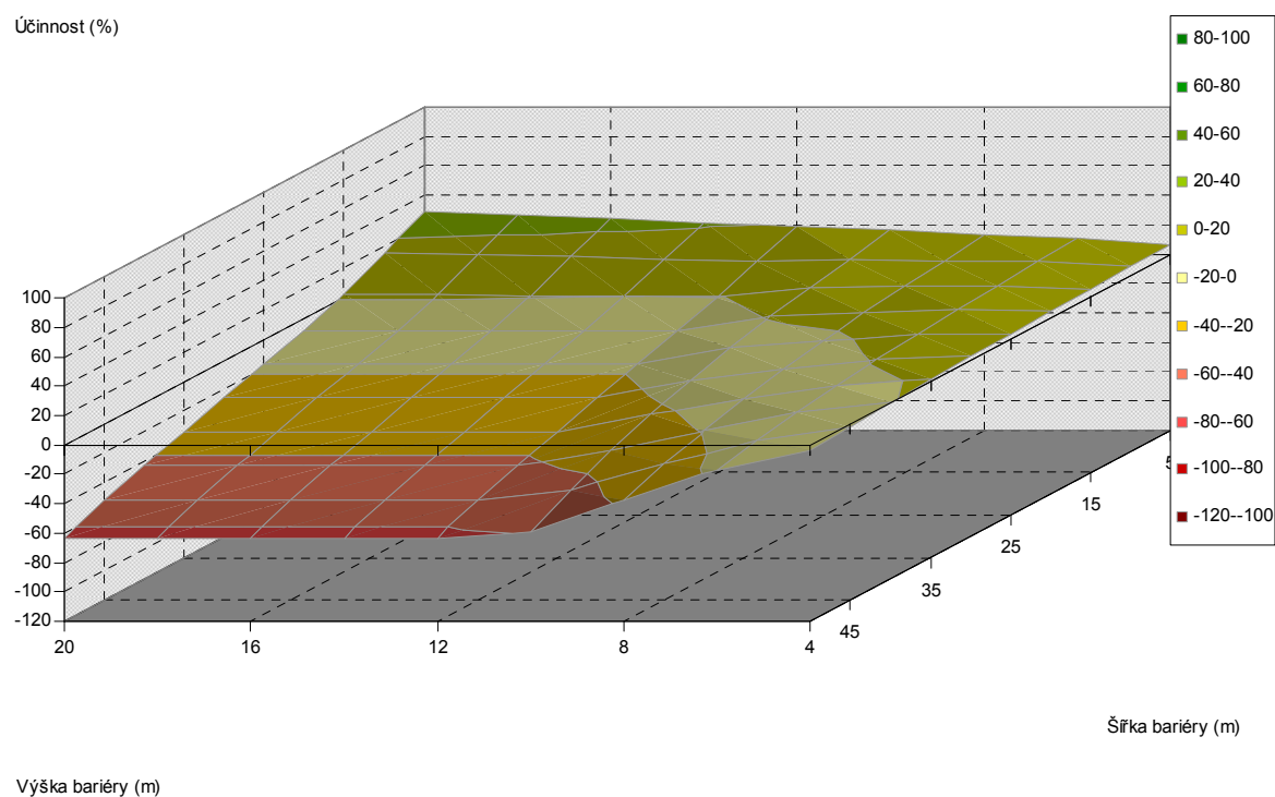
Obr. 5.282. Závislost účinnosti vegetační bariéry na výšce a šířce bariéry, pro vzdálenost od komunikace 60 m, listnaté dřeviny, PM10, 3 m nad povrchem
