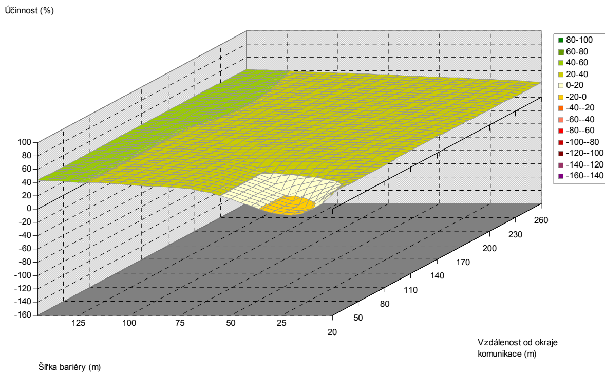
Obr. 5.166. Závislost účinnosti vegetační bariéry na šířce bariéry a vzdálenosti od komunikace, pro výšku bariéry 6 m, jehličnaté dřeviny, PM10, 3 m nad povrchem
