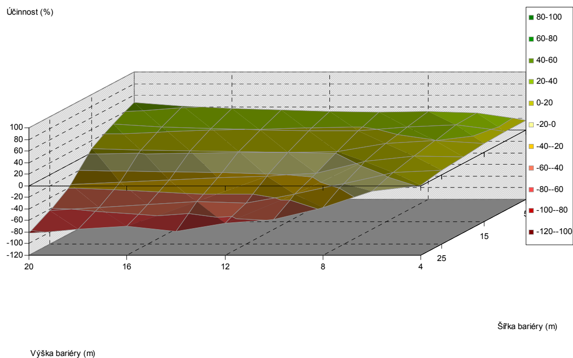
Obr. 5.268. Závislost účinnosti vegetační bariéry na výšce a šířce bariéry, pro vzdálenost od komunikace 40 m, jehličnaté dřeviny, PM10, 1,5 m nad povrchem
