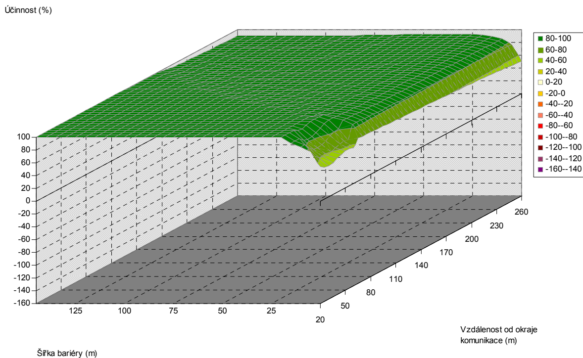
Obr. 5.230. Závislost účinnosti vegetační bariéry na šířce bariéry a vzdálenosti od komunikace, pro výšku bariéry 15 m, jehličnaté dřeviny, PM75, 3 m nad povrchem
