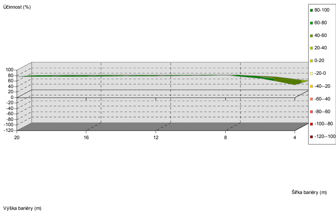
Obr. 5.370. Závislost účinnosti vegetační bariéry na výšce a šířce bariéry, pro vzdálenost od komunikace 20 m, jehličnaté dřeviny, PM75, 3 m nad povrchem
