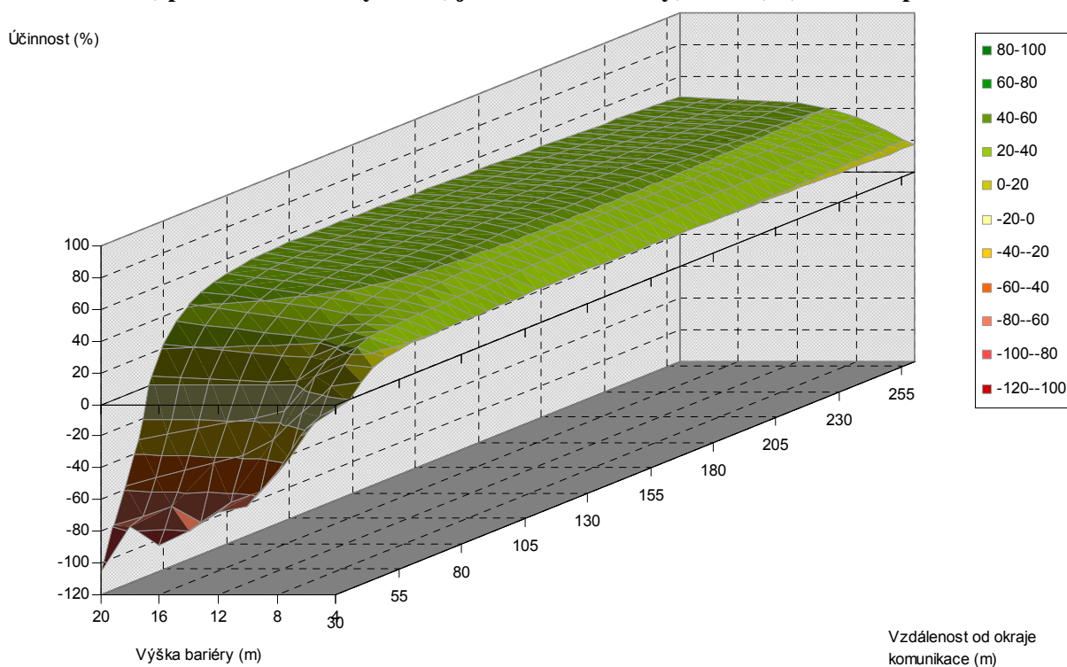
Obr. 5.16. Závislost účinnosti vegetační bariéry na výšce bariéry a vzdálenosti od komunikace, pro šířku bariéry 24 m, jehličnaté dřeviny, PM10, 1,5 m nad povrchem
