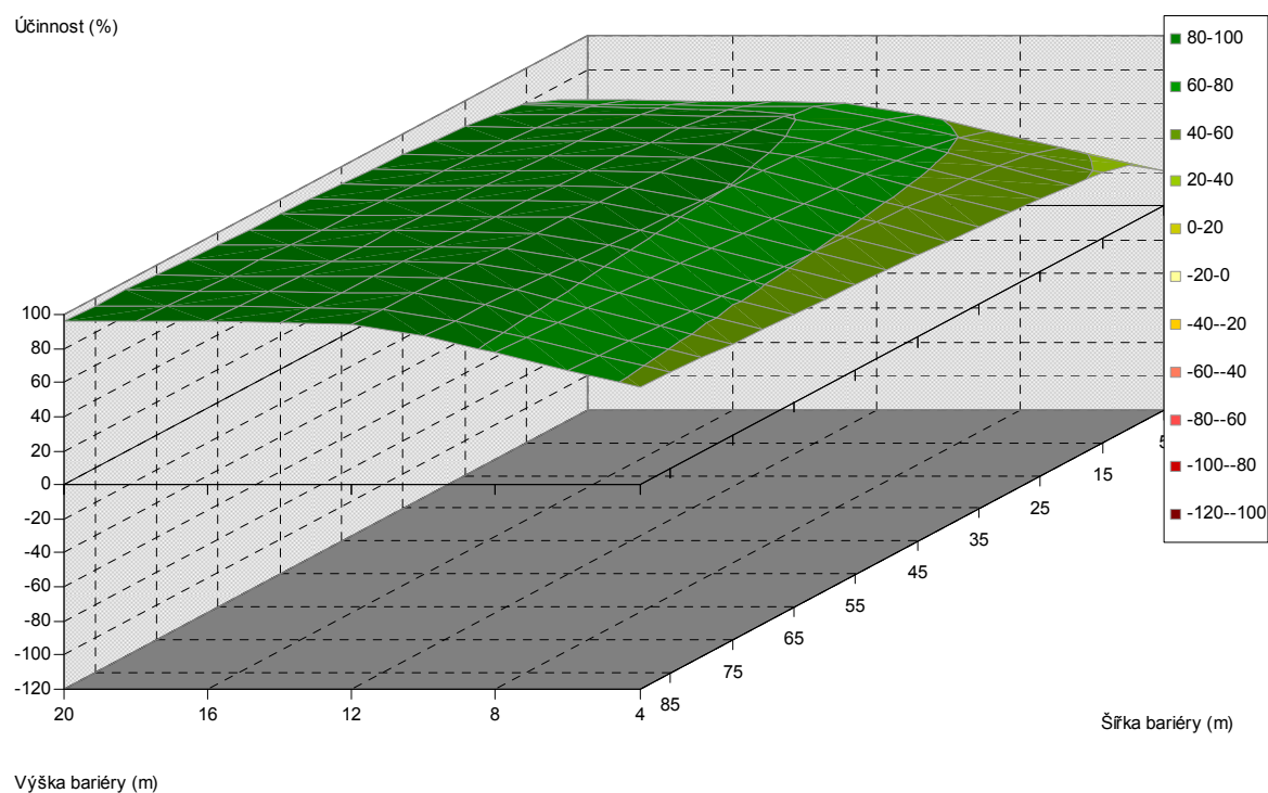
Obr. 5.388. Závislost účinnosti vegetační bariéry na výšce a šířce bariéry, pro vzdálenost od komunikace 100 m, listnaté dřeviny, PM75, 6 m nad povrchem
