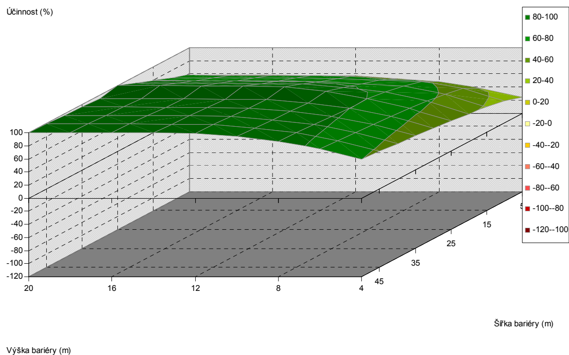
Obr. 5.334. Závislost účinnosti vegetační bariéry na výšce a šířce bariéry, pro vzdálenost od komunikace 60 m, listnaté dřeviny, PM75, 1,5 m nad povrchem
