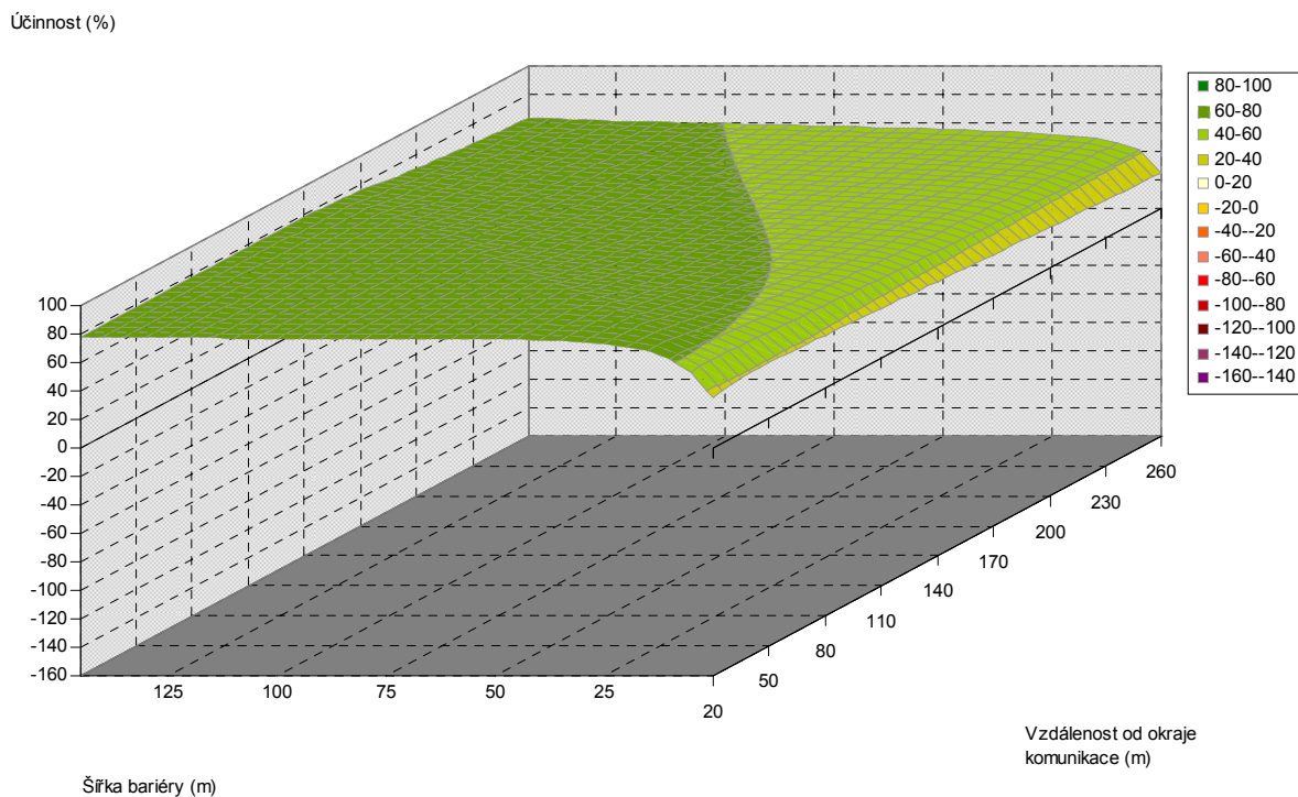
Obr. 5.196. Závislost účinnosti vegetační bariéry na šířce bariéry a vzdálenosti od komunikace, pro výšku bariéry 6 m, listnaté dřeviny, PM75, 1,5 m nad povrchem
