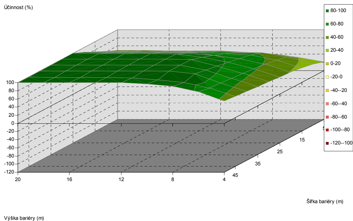
Obr. 5.360. Závislost účinnosti vegetační bariéry na výšce a šířce bariéry, pro vzdálenost od komunikace 60 m, listnaté dřeviny, PM75, 3 m nad povrchem
