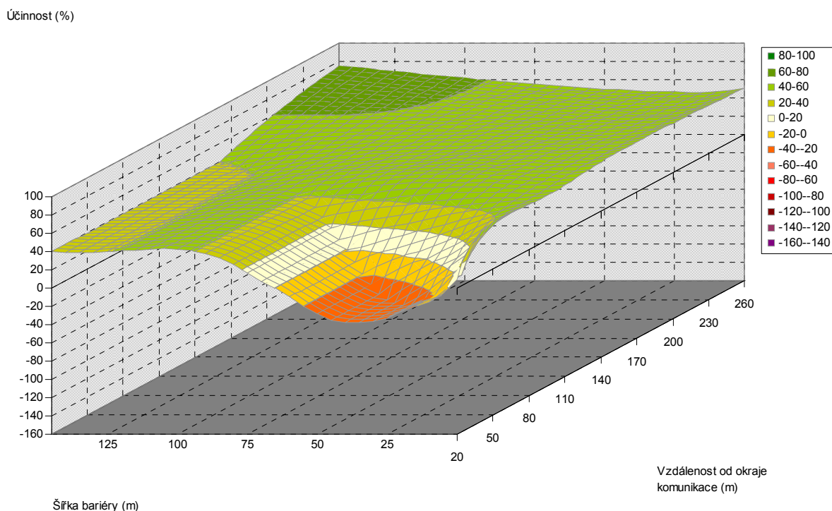
Obr. 5.172. Závislost účinnosti vegetační bariéry na šířce bariéry a vzdálenosti od komunikace, pro výšku bariéry 20 m, jehličnaté dřeviny, PM10, 3 m nad povrchem
