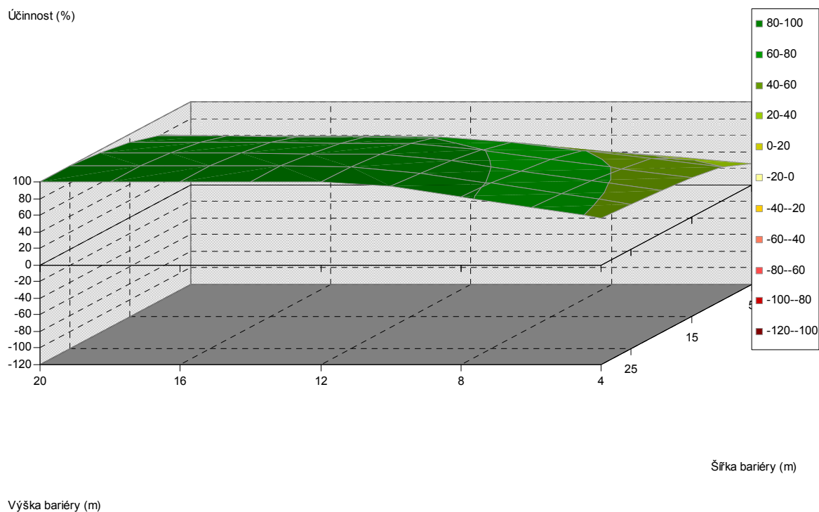
Obr. 5.398. Závislost účinnosti vegetační bariéry na výšce a šířce bariéry, pro vzdálenost od komunikace 40 m, jehličnaté dřeviny, PM75, 6 m nad povrchem
