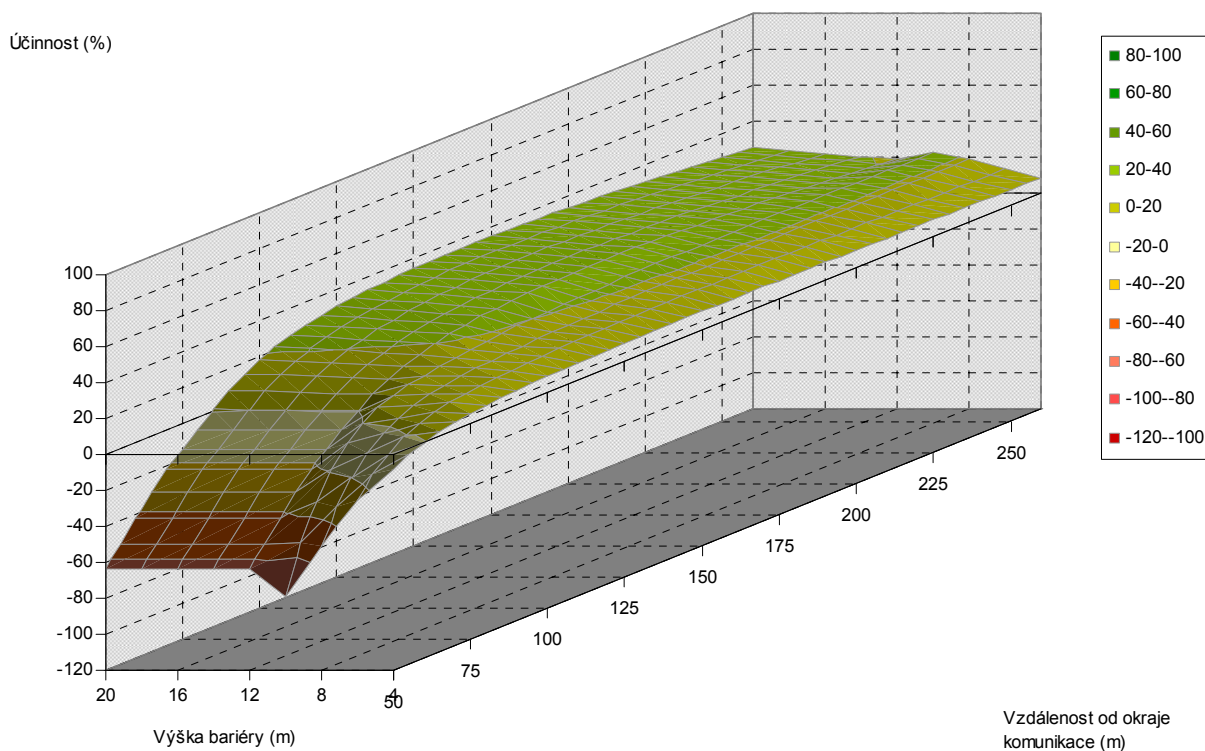
Obr. 5.30. Závislost účinnosti vegetační bariéry na výšce bariéry a vzdálenosti od komunikace, pro šířku bariéry 50 m, listnaté dřeviny, PM10, 3 m nad povrchem
