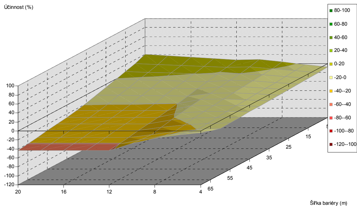
Obr. 5.309. Závislost účinnosti vegetační bariéry na výšce a šířce bariéry, pro vzdálenost od komunikace 80 m, listnaté dřeviny, PM10, 6 m nad povrchem
