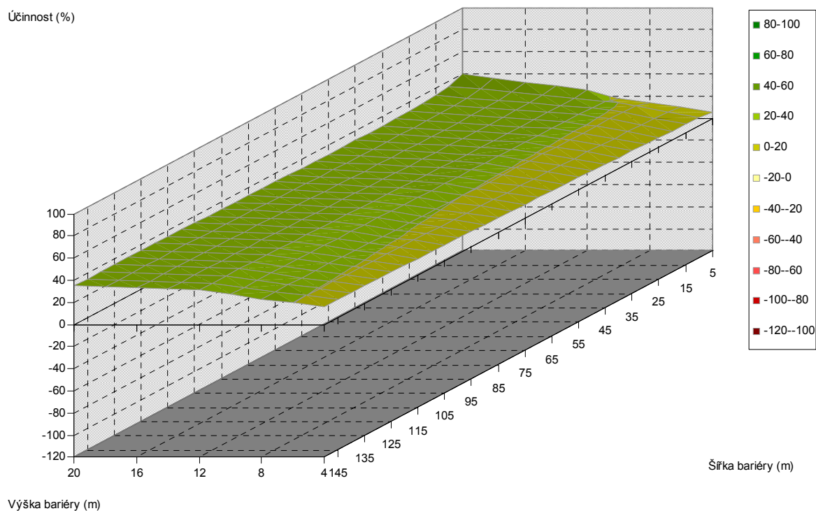
Obr. 5.290. Závislost účinnosti vegetační bariéry na výšce a šířce bariéry, pro vzdálenost od komunikace 220 m, listnaté dřeviny, PM10, 3 m nad povrchem
