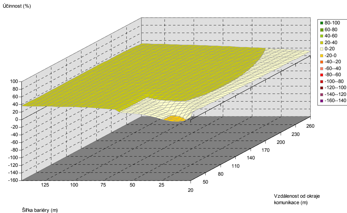
Obr. 5.144. Závislost účinnosti vegetační bariéry na šířce bariéry a vzdálenosti od komunikace, pro výšku bariéry 4 m, jehličnaté dřeviny, PM10, 1,5 m nad povrchem
