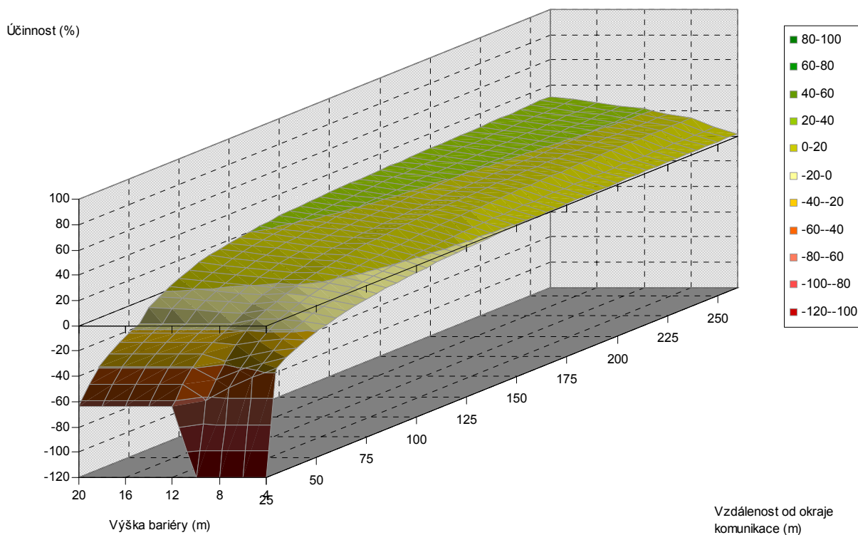
Obr. 5.48. Závislost účinnosti vegetační bariéry na výšce bariéry a vzdálenosti od komunikace, pro šířku bariéry 18 m, listnaté dřeviny, PM10, 6 m nad povrchem
