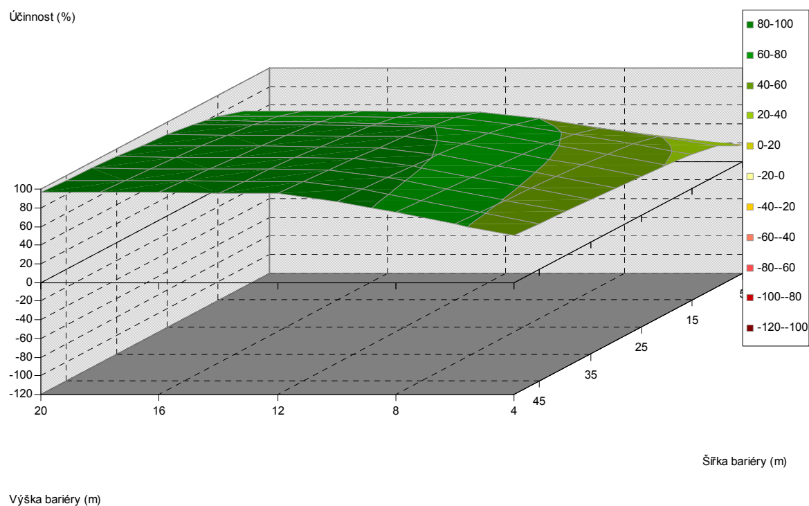
Obr. 5.386. Závislost účinnosti vegetační bariéry na výšce a šířce bariéry, pro vzdálenost od komunikace 60 m, listnaté dřeviny, PM75, 6 m nad povrchem
