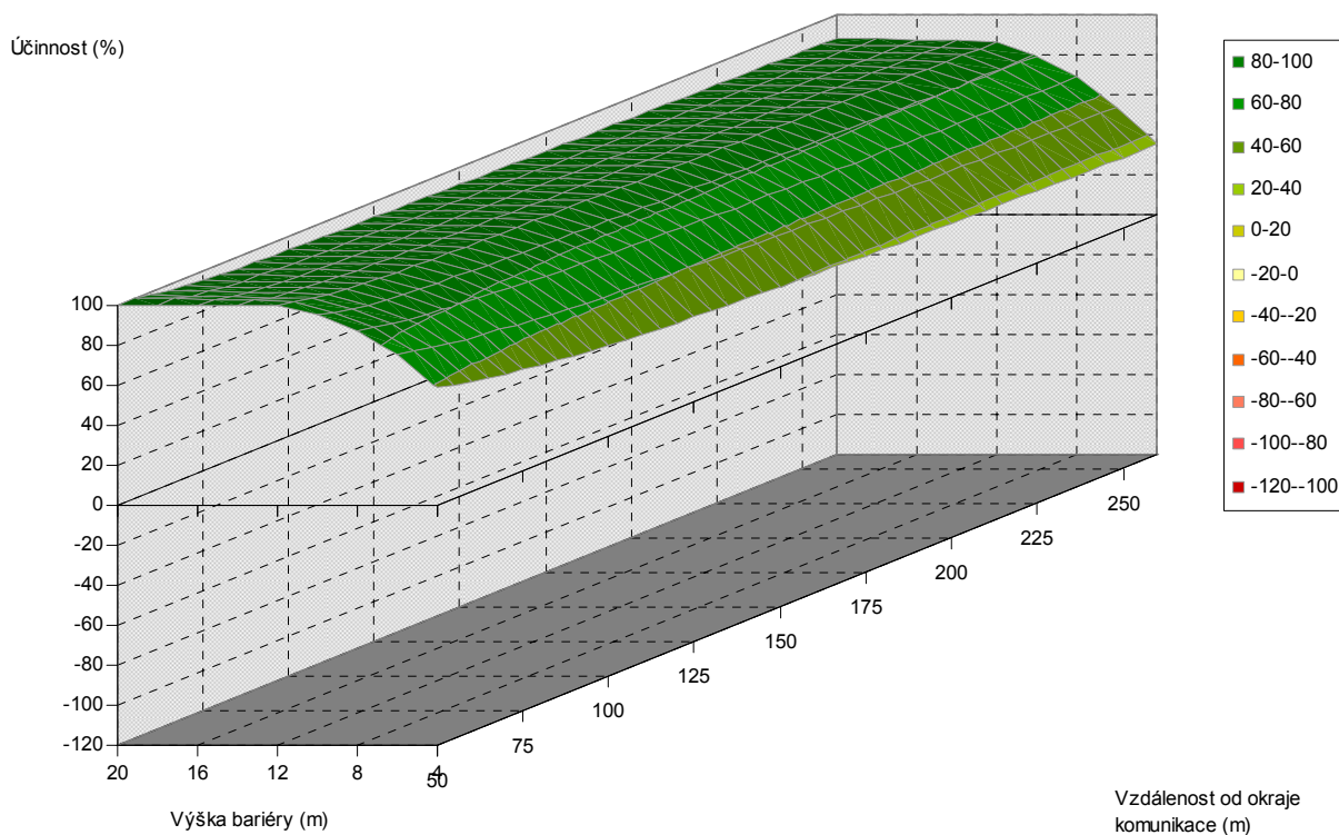
Obr. 5.74. Závislost účinnosti vegetační bariéry na výšce bariéry a vzdálenosti od komunikace, pro šířku bariéry 50 m, listnaté dřeviny, PM75, 1,5 m nad povrchem
