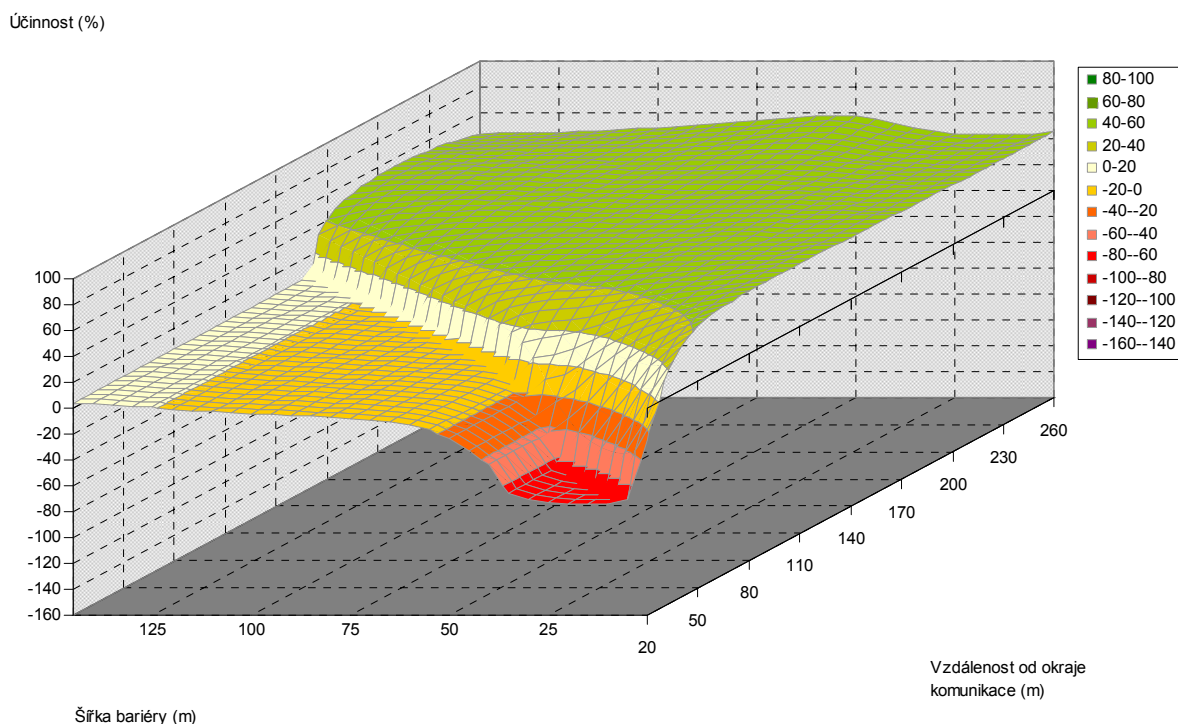
Obr. 5.150. Závislost účinnosti vegetační bariéry na šířce bariéry a vzdálenosti od komunikace, pro výšku bariéry 15 m, jehličnaté dřeviny, PM10, 1,5 m nad povrchem
