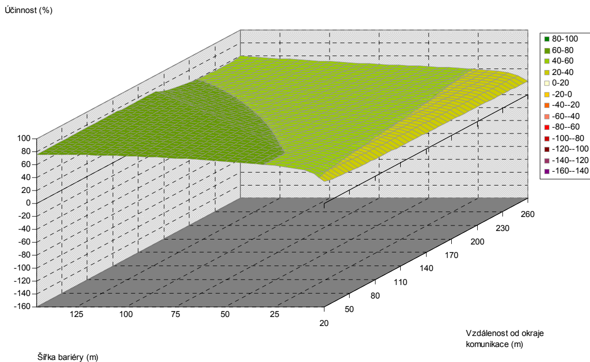
Obr. 5.224. Závislost účinnosti vegetační bariéry na šířce bariéry a vzdálenosti od komunikace, pro výšku bariéry 4 m, jehličnaté dřeviny, PM75, 3 m nad povrchem
