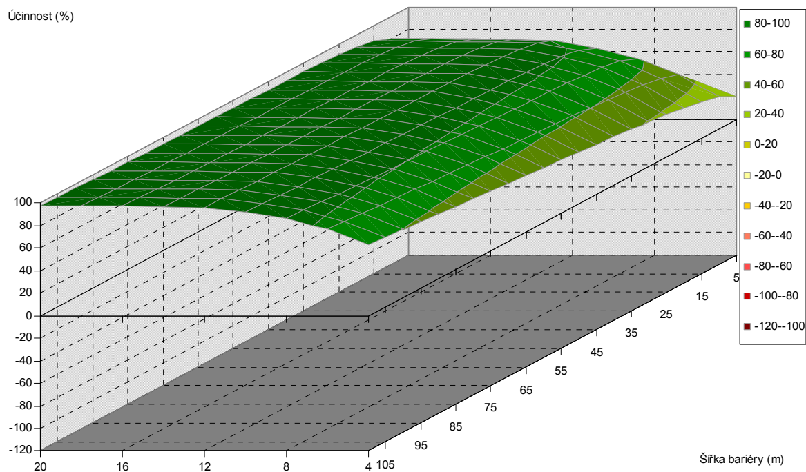
Obr. 5.337. Závislost účinnosti vegetační bariéry na výšce a šířce bariéry, pro vzdálenost od komunikace 120 m, listnaté dřeviny, PM75, 1,5 m nad povrchem
