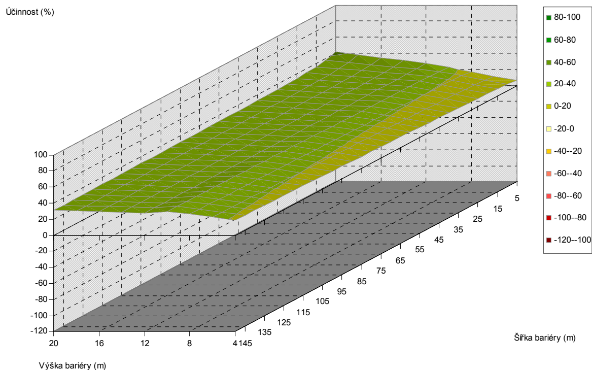
Obr. 5.264. Závislost účinnosti vegetační bariéry na výšce a šířce bariéry, pro vzdálenost od komunikace 220 m, listnaté dřeviny, PM10, 1,5 m nad povrchem
