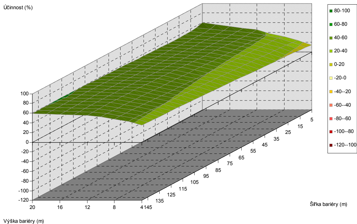
Obr. 5.302. Závislost účinnosti vegetační bariéry na výšce a šířce bariéry, pro vzdálenost od komunikace 200 m, jehličnaté dřeviny, PM10, 3 m nad povrchem
