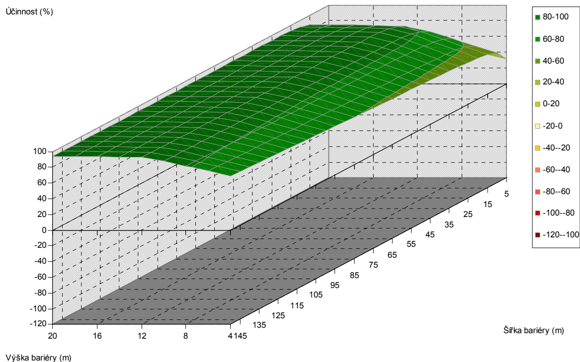
Obr. 5.406. Závislost účinnosti vegetační bariéry na výšce a šířce bariéry, pro vzdálenost od komunikace 200 m, jehličnaté dřeviny, PM75, 6 m nad povrchem
