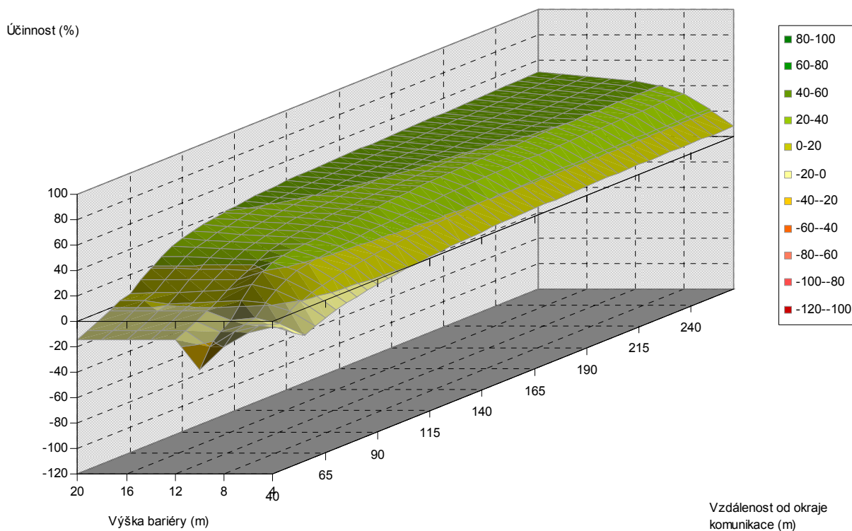
Obr. 5.62. Závislost účinnosti vegetační bariéry na výšce bariéry a vzdálenosti od komunikace, pro šířku bariéry 40 m, jehličnaté dřeviny, PM10, 6 m nad povrchem
