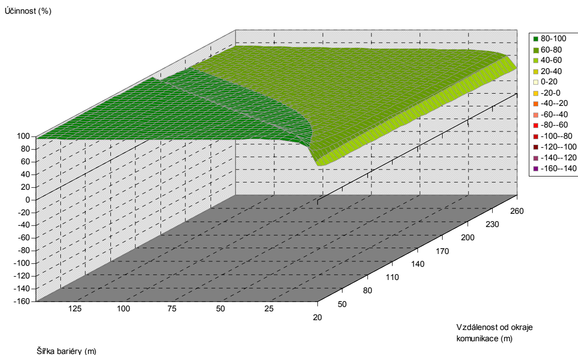
Obr. 5.228. Závislost účinnosti vegetační bariéry na šířce bariéry a vzdálenosti od komunikace, pro výšku bariéry 11 m, jehličnaté dřeviny, PM75, 3 m nad povrchem
