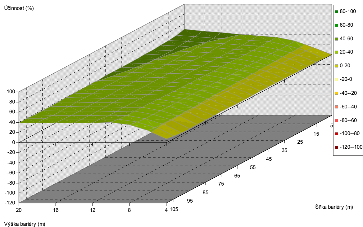
Obr. 5.324. Závislost účinnosti vegetační bariéry na výšce a šířce bariéry, pro vzdálenost od komunikace 120 m, jehličnaté dřeviny, PM10, 6 m nad povrchem
