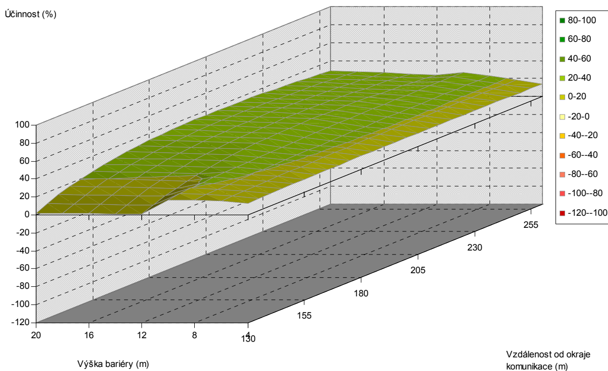
Obr. 5.34. Závislost účinnosti vegetační bariéry na výšce bariéry a vzdálenosti od komunikace, pro šířku bariéry 4 m, jehličnaté dřeviny, PM10, 3 m nad povrchem
