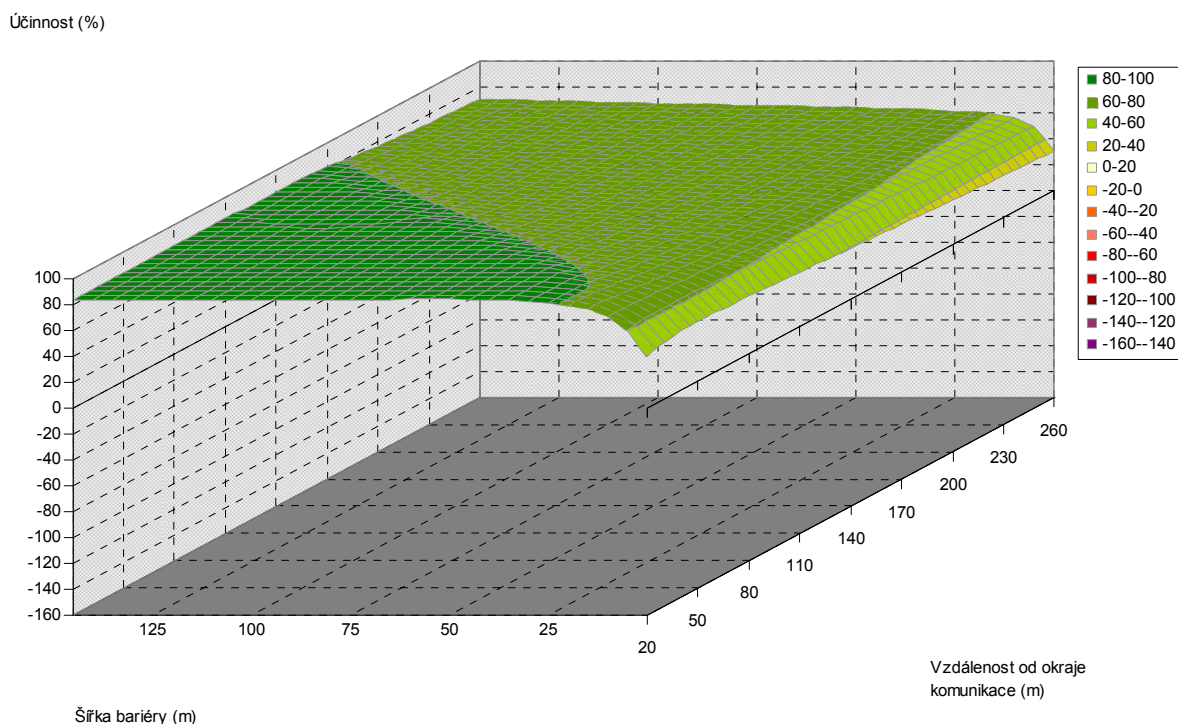
Obr. 5.198. Závislost účinnosti vegetační bariéry na šířce bariéry a vzdálenosti od komunikace, pro výšku bariéry 11 m, listnaté dřeviny, PM75, 1,5 m nad povrchem
