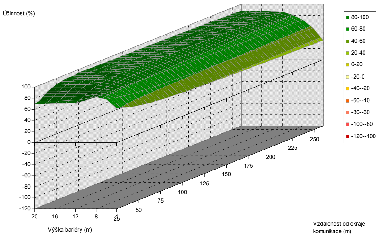
Obr. 5.82. Závislost účinnosti vegetační bariéry na výšce bariéry a vzdálenosti od komunikace, pro šířku bariéry 24 m, jehličnaté dřeviny, PM75, 1,5 m nad povrchem
