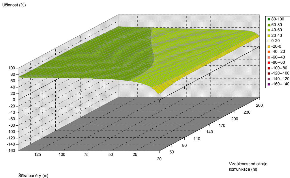
Obr. 5.244. Závislost účinnosti vegetační bariéry na šířce bariéry a vzdálenosti od komunikace, pro výšku bariéry 4 m, jehličnaté dřeviny, PM75, 6 m nad povrchem
