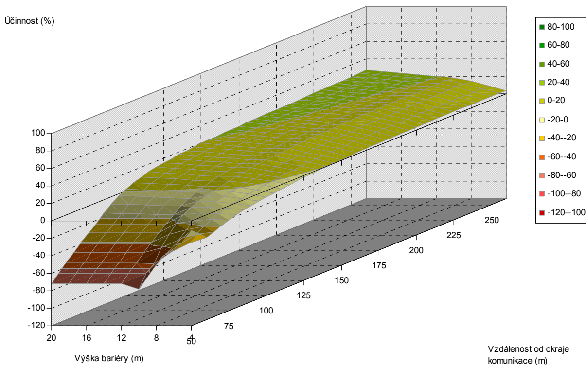
Obr. 5.52. Závislost účinnosti vegetační bariéry na výšce bariéry a vzdálenosti od komunikace, pro šířku bariéry 50 m, listnaté dřeviny, PM10, 6 m nad povrchem
