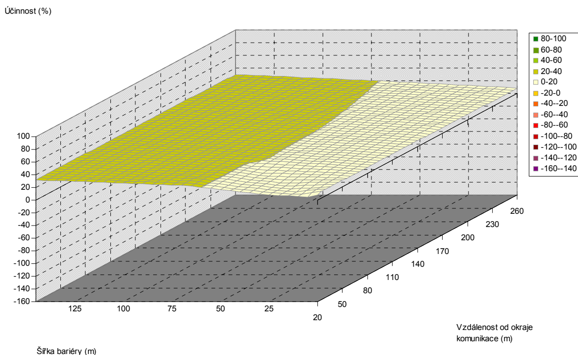
Obr. 5.164. Závislost účinnosti vegetační bariéry na šířce bariéry a vzdálenosti od komunikace, pro výšku bariéry 4 m, jehličnaté dřeviny, PM10, 3 m nad povrchem
