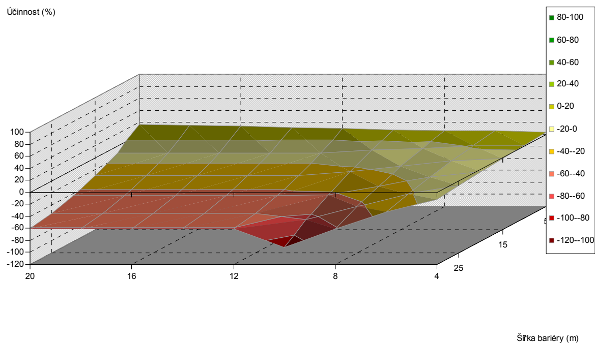
Obr. 5.281. Závislost účinnosti vegetační bariéry na výšce a šířce bariéry, pro vzdálenost od komunikace 40 m, listnaté dřeviny, PM10, 3 m nad povrchem
