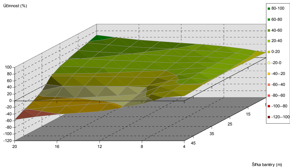
Obr. 5.269. Závislost účinnosti vegetační bariéry na výšce a šířce bariéry, pro vzdálenost od komunikace 60 m, jehličnaté dřeviny, PM10, 1,5 m nad povrchem
