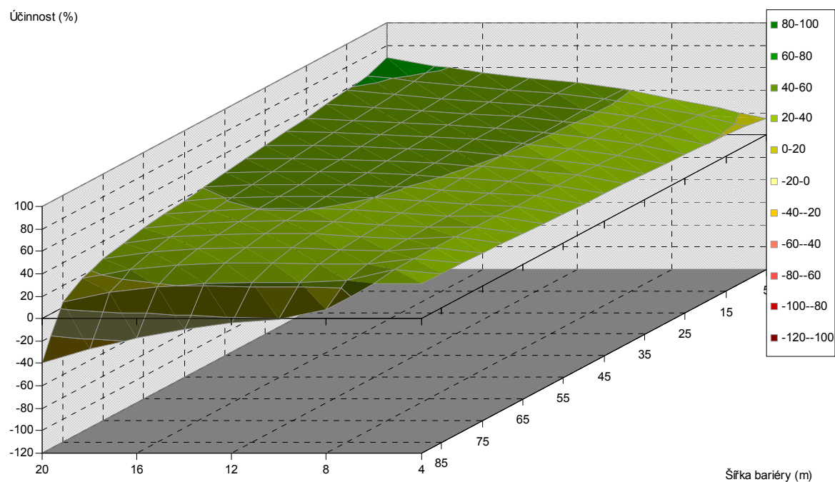
Obr. 5.271. Závislost účinnosti vegetační bariéry na výšce a šířce bariéry, pro vzdálenost od komunikace 100 m, jehličnaté dřeviny, PM10, 1,5 m nad povrchem
