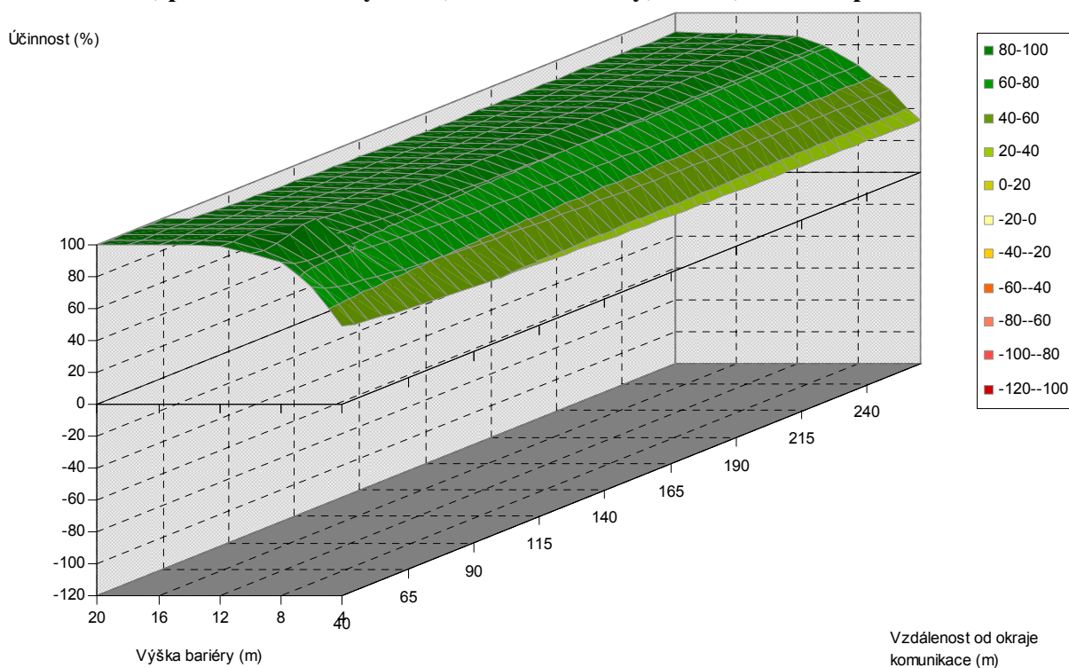
Obr. 5.94. Závislost účinnosti vegetační bariéry na výšce bariéry a vzdálenosti od komunikace, pro šířku bariéry 30 m, listnaté dřeviny, PM75, 3 m nad povrchem
