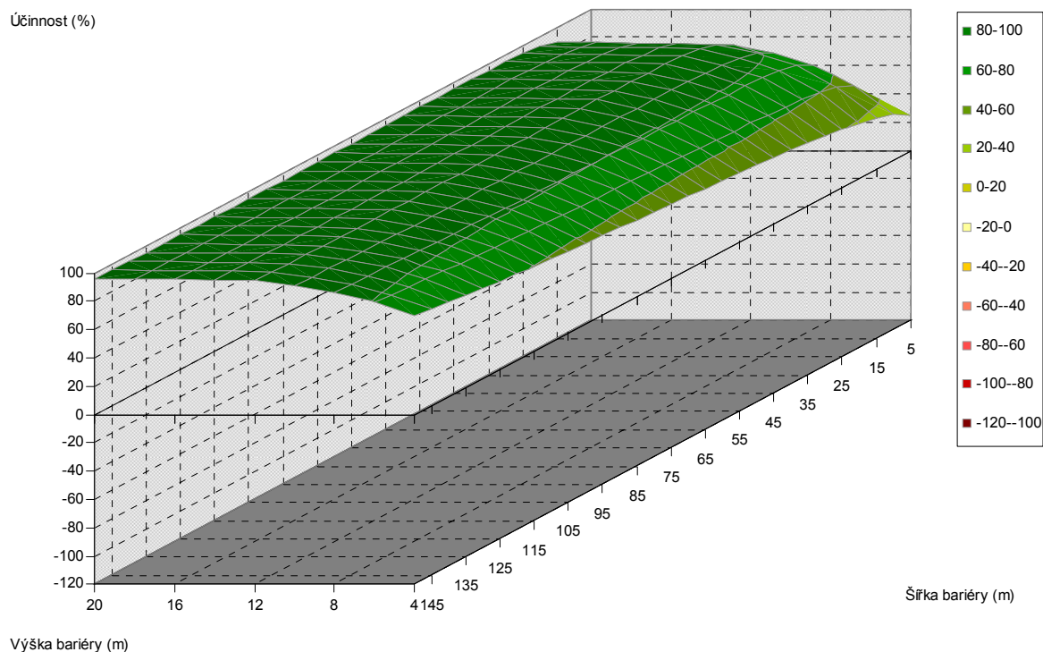
Obr. 5.354. Závislost účinnosti vegetační bariéry na výšce a šířce bariéry, pro vzdálenost od komunikace 200 m, jehličnaté dřeviny, PM75, 1,5 m nad povrchem
