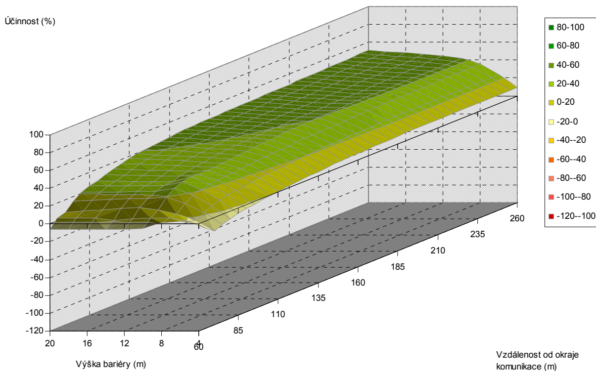
Obr. 5.64. Závislost účinnosti vegetační bariéry na výšce bariéry a vzdálenosti od komunikace, pro šířku bariéry 70 m, jehličnaté dřeviny, PM10, 6 m nad povrchem
