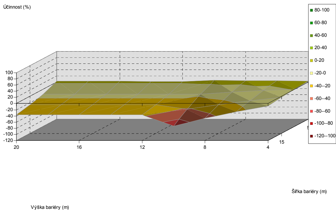
Obr. 5.254. Závislost účinnosti vegetační bariéry na výšce a šířce bariéry, pro vzdálenost od komunikace 30 m, listnaté dřeviny, PM10, 1,5 m nad povrchem
