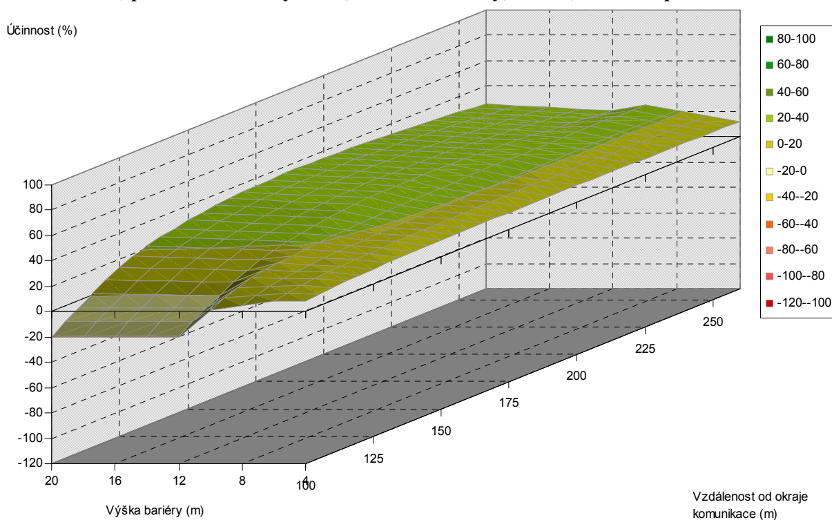
Obr. 5.32. Závislost účinnosti vegetační bariéry na výšce bariéry a vzdálenosti od komunikace, pro šířku bariéry 90 m, listnaté dřeviny, PM10, 3 m nad povrchem
