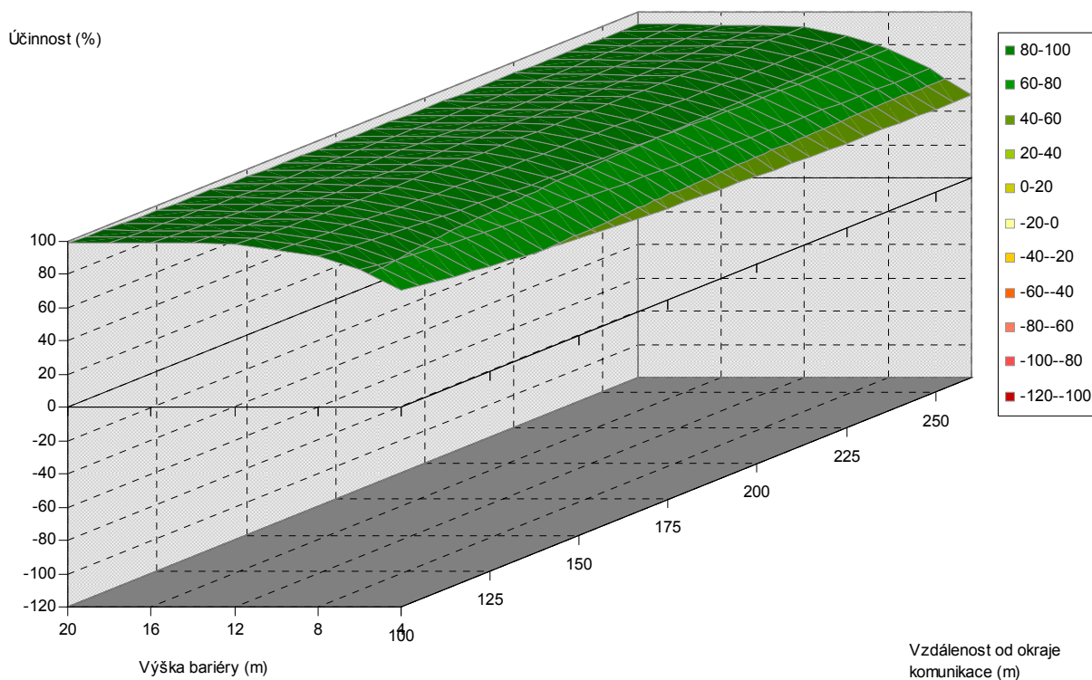
Obr. 5.88. Závislost účinnosti vegetační bariéry na výšce bariéry a vzdálenosti od komunikace, pro šířku bariéry 120 m, jehličnaté dřeviny, PM75, 1,5 m nad povrchem
