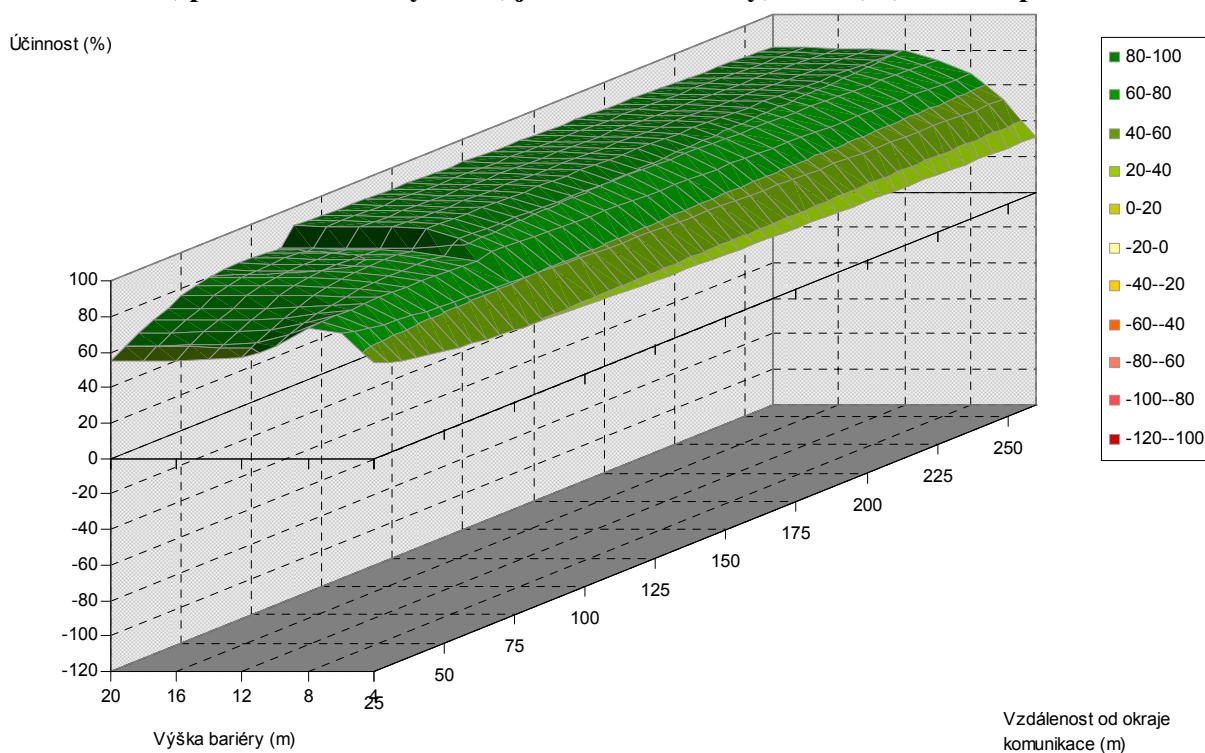
Obr. 5.80. Závislost účinnosti vegetační bariéry na výšce bariéry a vzdálenosti od komunikace, pro šířku bariéry 12 m, jehličnaté dřeviny, PM75, 1,5 m nad povrchem
