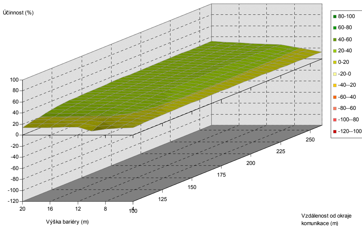
Obr. 5.10. Závislost účinnosti vegetační bariéry na výšce bariéry a vzdálenosti od komunikace, pro šířku bariéry 90 m, listnaté dřeviny, PM10, 1,5 m nad povrchem
