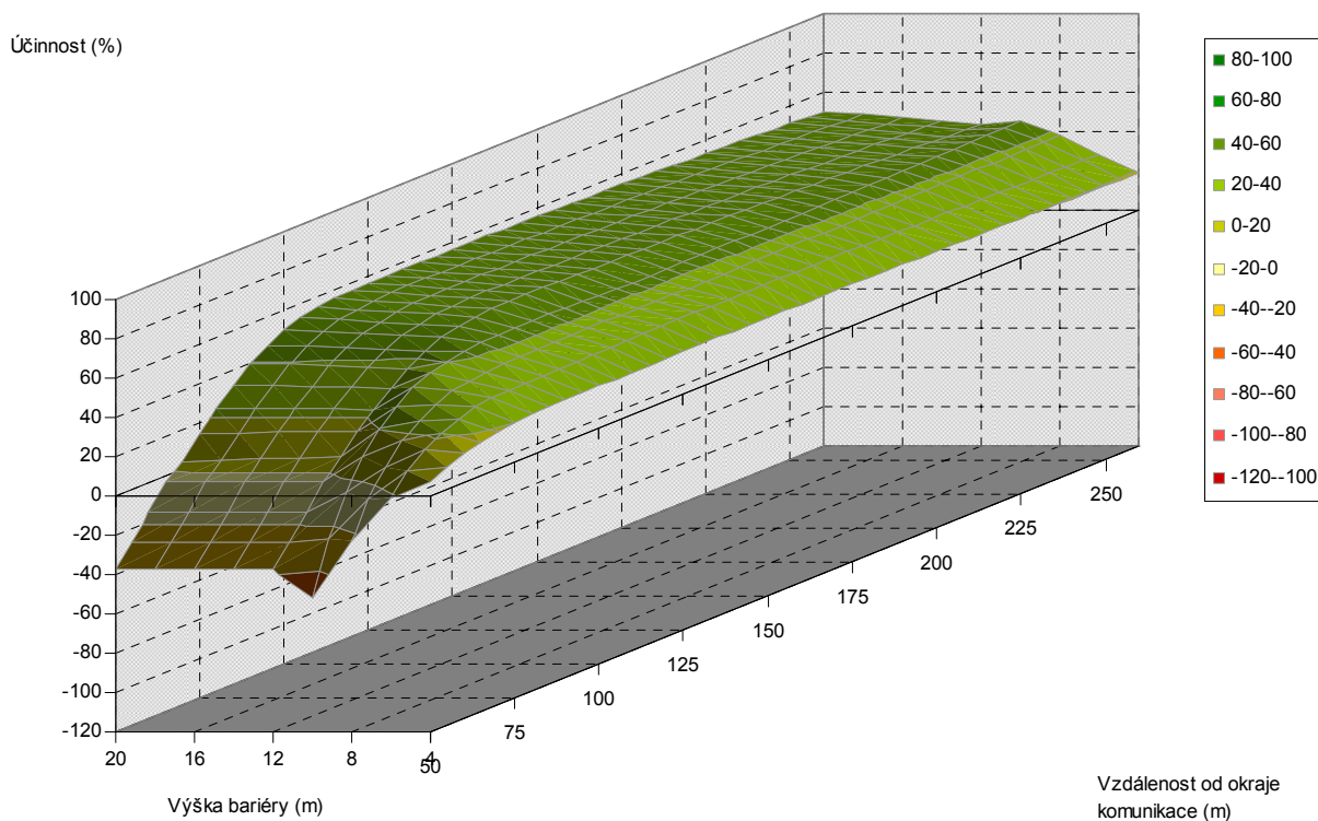
Obr. 5.40. Závislost účinnosti vegetační bariéry na výšce bariéry a vzdálenosti od komunikace, pro šířku bariéry 40 m, jehličnaté dřeviny, PM10, 3 m nad povrchem
