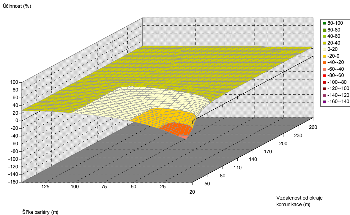
Obr. 5.138. Závislost účinnosti vegetační bariéry na šířce bariéry a vzdálenosti od komunikace, pro výšku bariéry 11 m, listnaté dřeviny, PM10, 1,5 m nad povrchem
