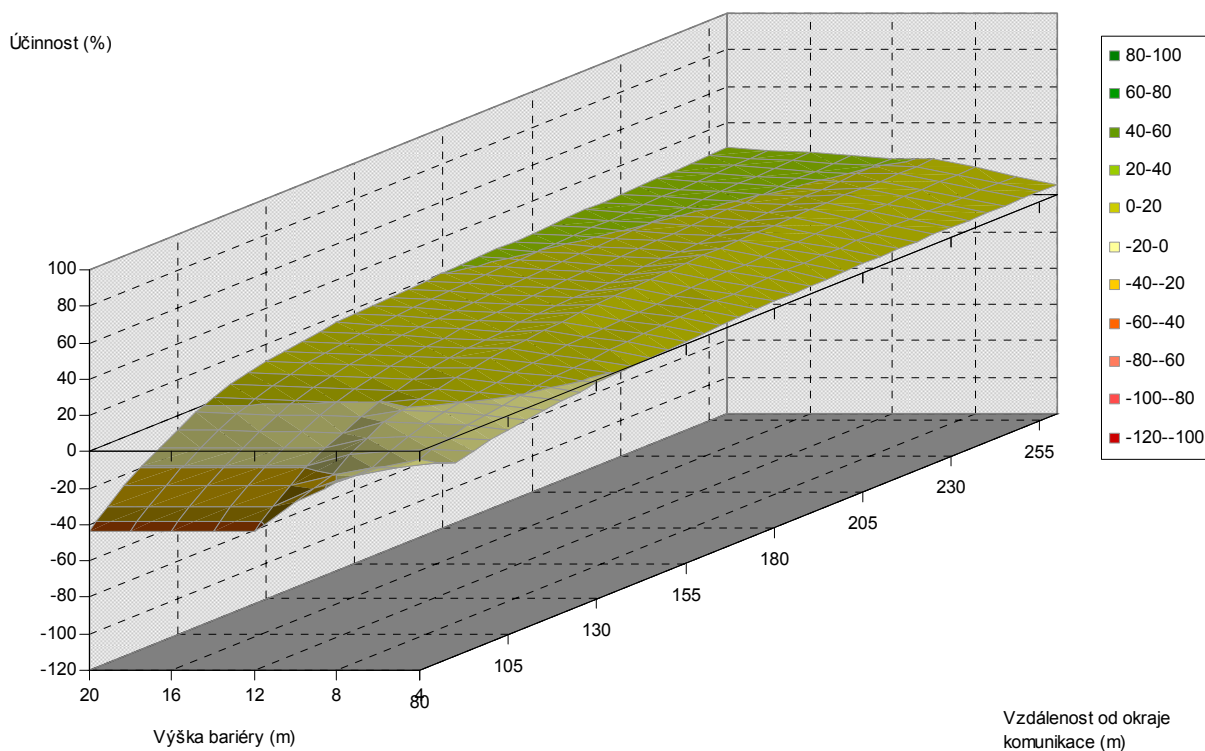
Obr. 5.54. Závislost účinnosti vegetační bariéry na výšce bariéry a vzdálenosti od komunikace, pro šířku bariéry 90 m, listnaté dřeviny, PM10, 6 m nad povrchem
