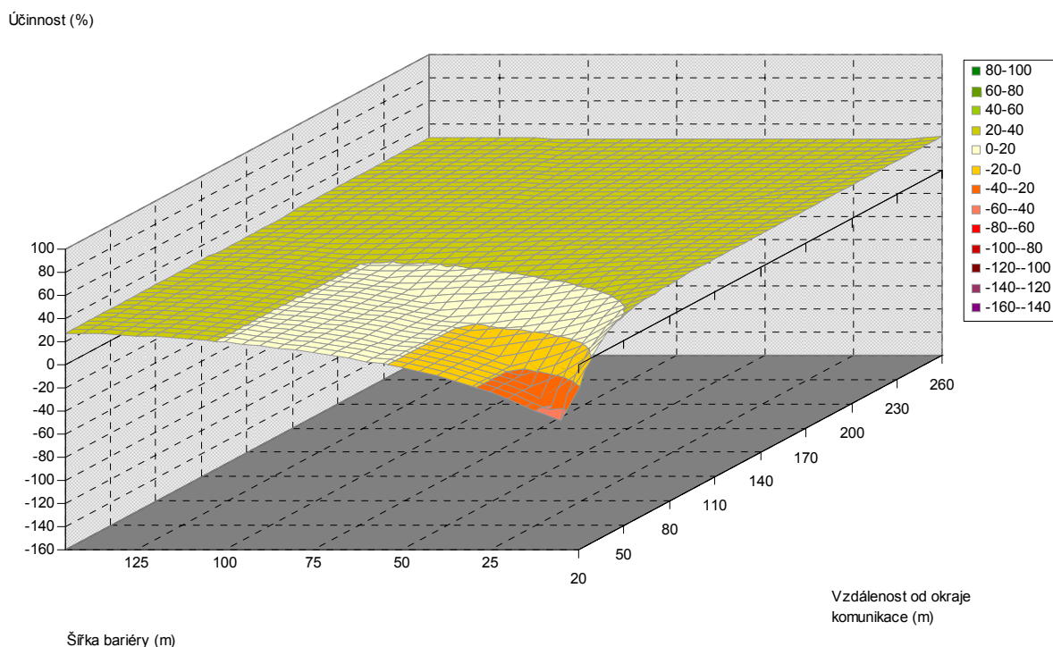
Obr. 5.140. Závislost účinnosti vegetační bariéry na šířce bariéry a vzdálenosti od komunikace, pro výšku bariéry 15 m, listnaté dřeviny, PM10, 1,5 m nad povrchem
