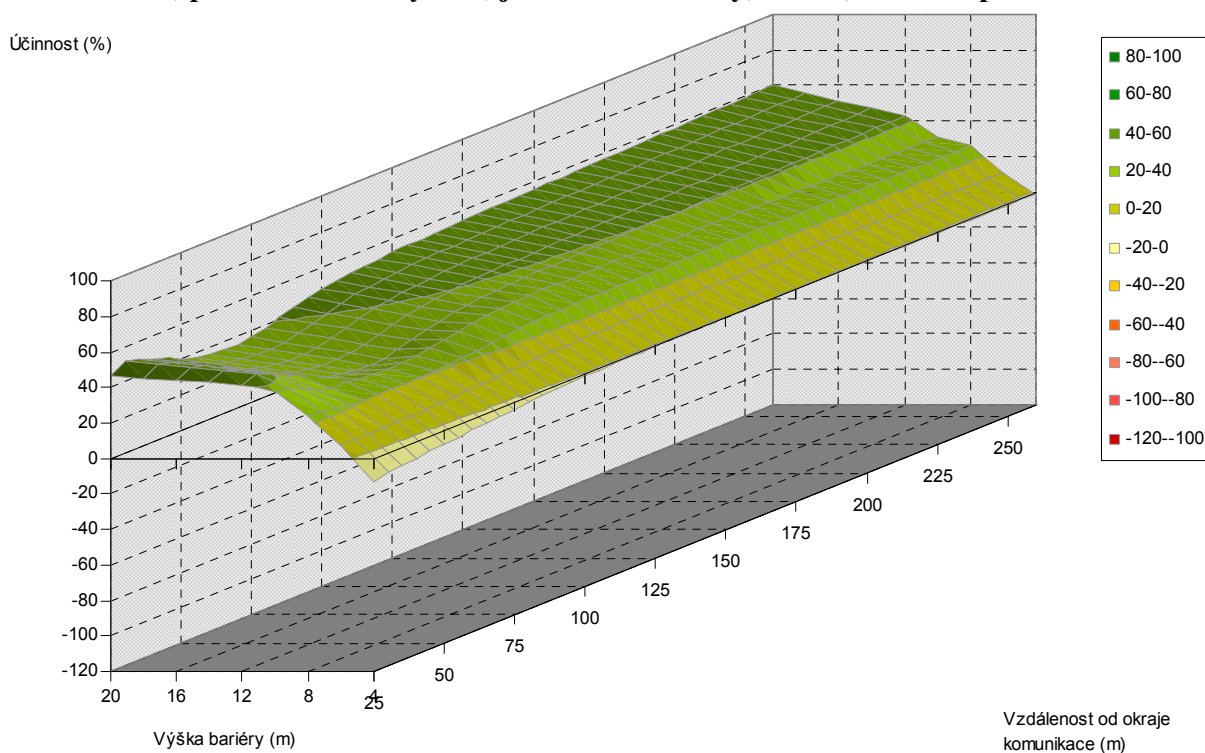
Obr. 5.56. Závislost účinnosti vegetační bariéry na výšce bariéry a vzdálenosti od komunikace, pro šířku bariéry 4 m, jehličnaté dřeviny, PM10, 6 m nad povrchem
