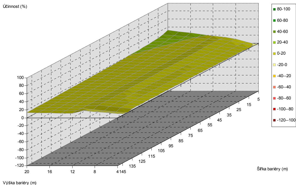
Obr. 5.314. Závislost účinnosti vegetační bariéry na výšce a šířce bariéry, pro vzdálenost od komunikace 180 m, listnaté dřeviny, PM10, 6 m nad povrchem
