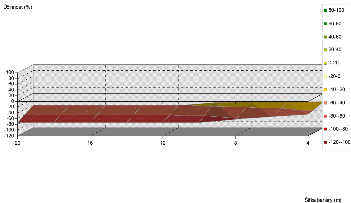
Obr. 5.305. Závislost účinnosti vegetační bariéry na výšce a šířce bariéry, pro vzdálenost od komunikace 20 m, listnaté dřeviny, PM10, 6 m nad povrchem
