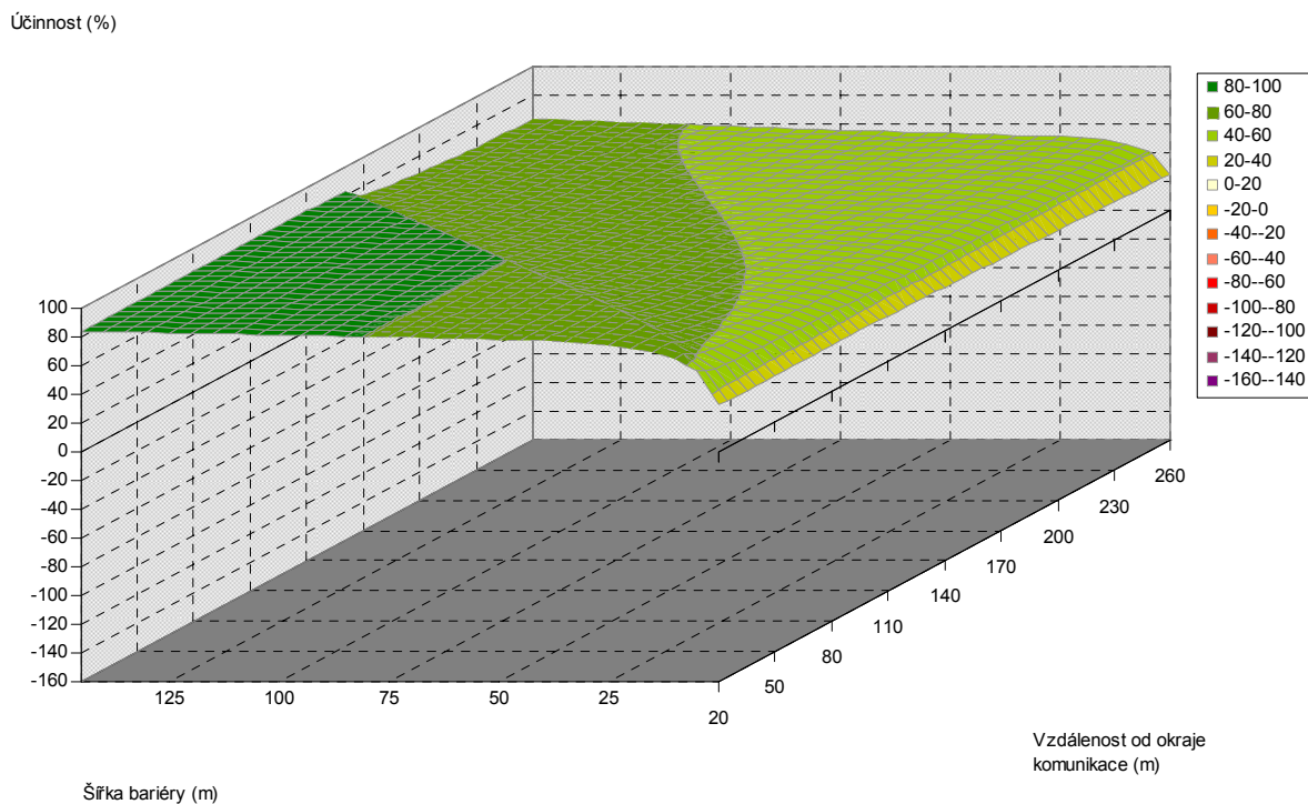
Obr. 5.216. Závislost účinnosti vegetační bariéry na šířce bariéry a vzdálenosti od komunikace, pro výšku bariéry 6 m, listnaté dřeviny, PM75, 3 m nad povrchem
