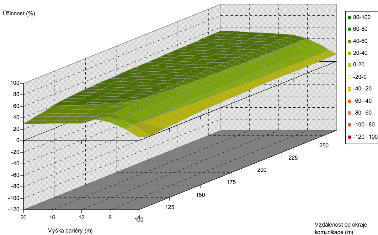
Obr. 5.66. Závislost účinnosti vegetační bariéry na výšce bariéry a vzdálenosti od komunikace, pro šířku bariéry 120 m, jehličnaté dřeviny, PM10, 6 m nad povrchem
