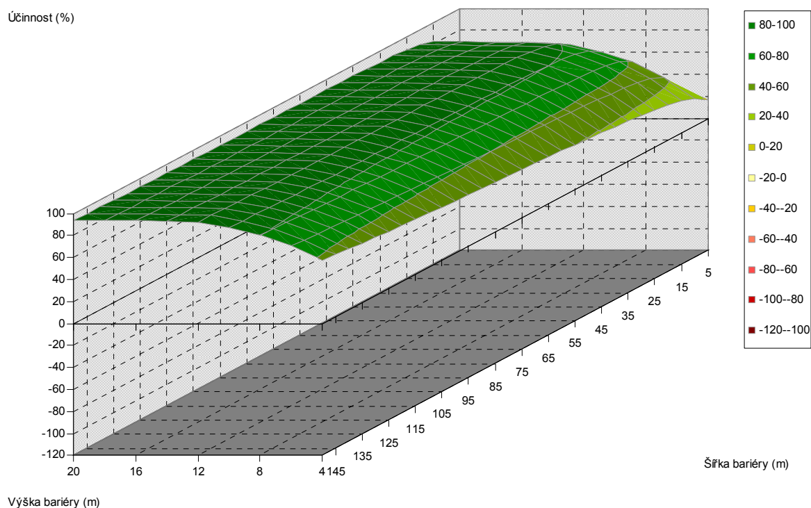
Obr. 5.342. Závislost účinnosti vegetační bariéry na výšce a šířce bariéry, pro vzdálenost od komunikace 220 m, listnaté dřeviny, PM75, 1,5 m nad povrchem
