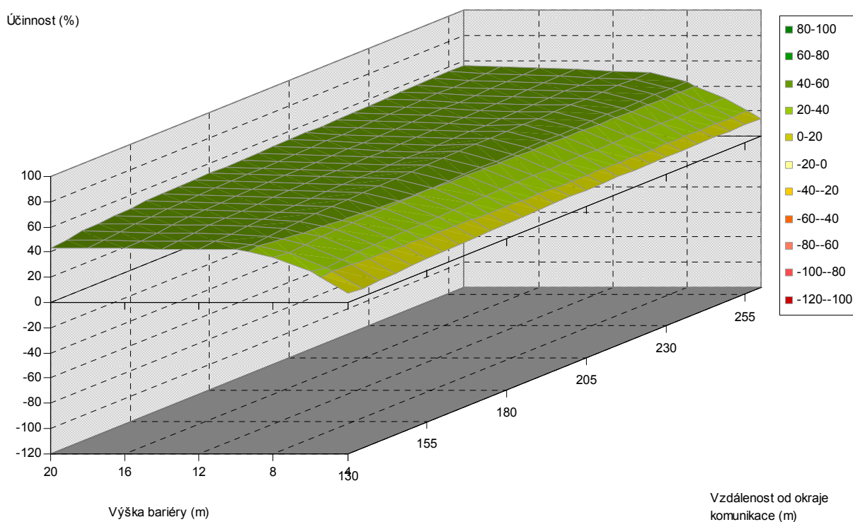
Obr. 5.66. Závislost účinnosti vegetační bariéry na výšce bariéry a vzdálenosti od komunikace, pro šířku bariéry 120 m, jehličnaté dřeviny, PM10, 6 m nad povrchem
