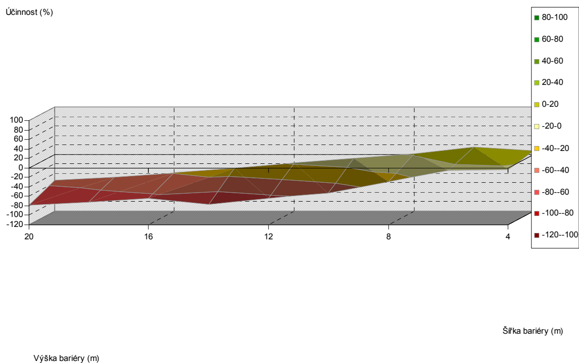
Obr. 5.266. Závislost účinnosti vegetační bariéry na výšce a šířce bariéry, pro vzdálenost od komunikace 20 m, jehličnaté dřeviny, PM10, 1,5 m nad povrchem
