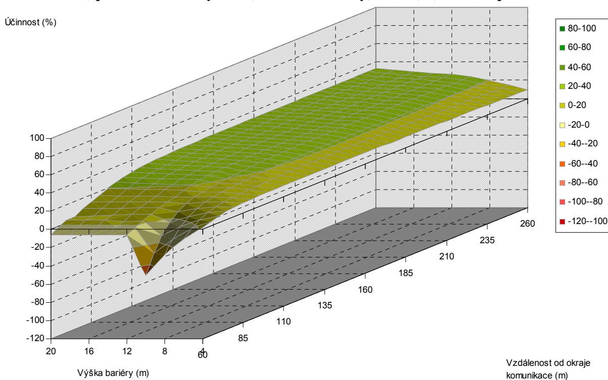
Obr. 5.8. Závislost účinnosti vegetační bariéry na výšce bariéry a vzdálenosti od komunikace, pro šířku bariéry 50 m, listnaté dřeviny, PM10, 1,5 m nad povrchem
