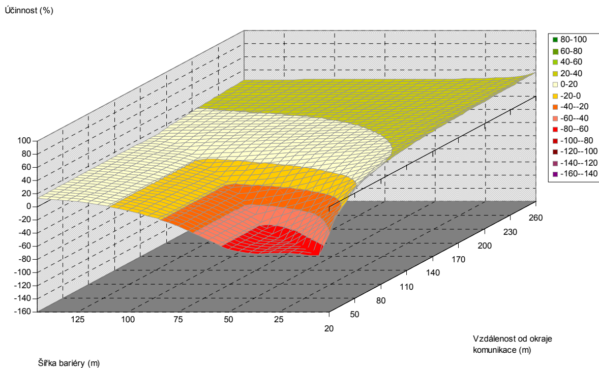
Obr. 5.182. Závislost účinnosti vegetační bariéry na šířce bariéry a vzdálenosti od komunikace, pro výšku bariéry 20 m, listnaté dřeviny, PM10, 6 m nad povrchem
