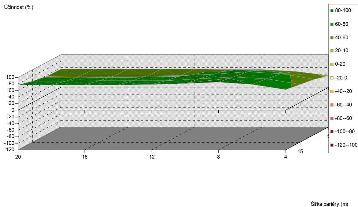
Obr. 5.345. Závislost účinnosti vegetační bariéry na výšce a šířce bariéry, pro vzdálenost od komunikace 30 m, jehličnaté dřeviny, PM75, 1,5 m nad povrchem
