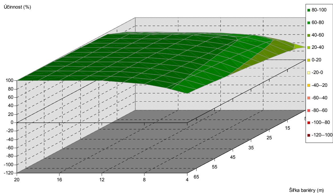
Obr. 5.348. Závislost účinnosti vegetační bariéry na výšce a šířce bariéry, pro vzdálenost od komunikace 80 m, jehličnaté dřeviny, PM75, 1,5 m nad povrchem
