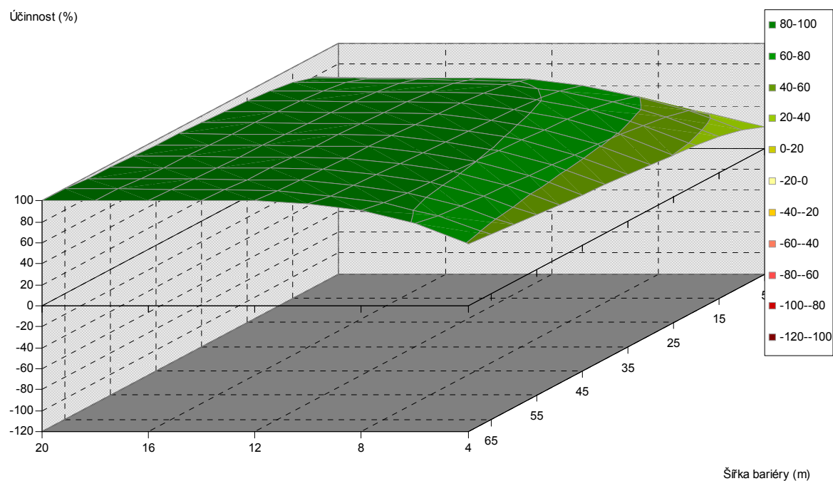
Obr. 5.361. Závislost účinnosti vegetační bariéry na výšce a šířce bariéry, pro vzdálenost od komunikace 80 m, listnaté dřeviny, PM75, 3 m nad povrchem
