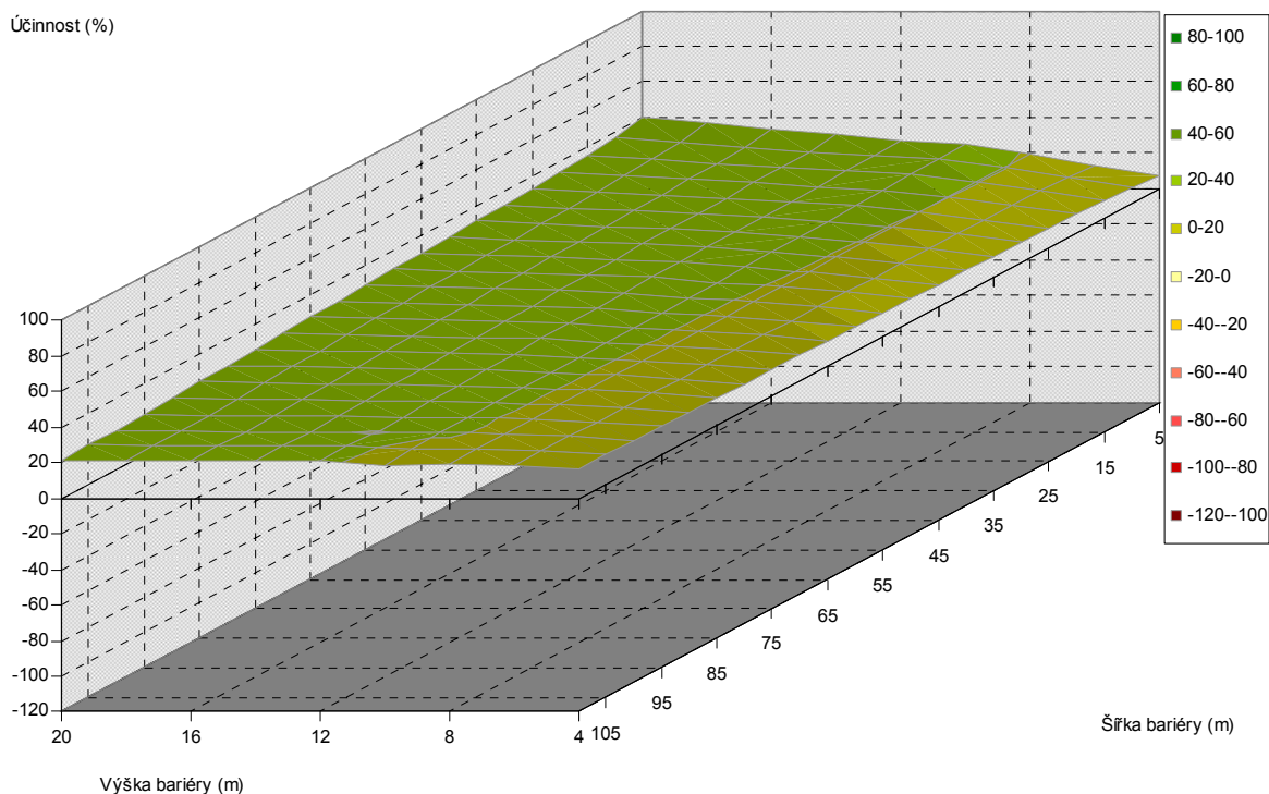
Obr. 5.260. Závislost účinnosti vegetační bariéry na výšce a šířce bariéry, pro vzdálenost od komunikace 140 m, listnaté dřeviny, PM10, 1,5 m nad povrchem
