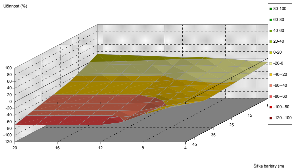
Obr. 5.308. Závislost účinnosti vegetační bariéry na výšce a šířce bariéry, pro vzdálenost od komunikace 60 m, listnaté dřeviny, PM10, 6 m nad povrchem
