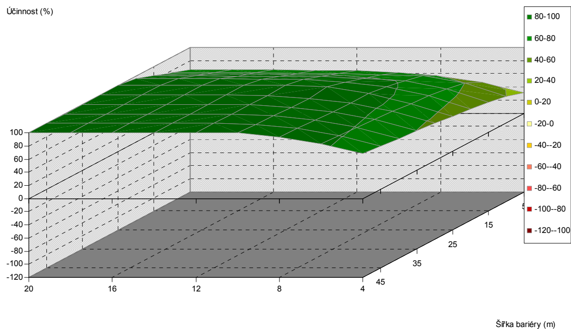
Obr. 5.347. Závislost účinnosti vegetační bariéry na výšce a šířce bariéry, pro vzdálenost od komunikace 60 m, jehličnaté dřeviny, PM75, 1,5 m nad povrchem
