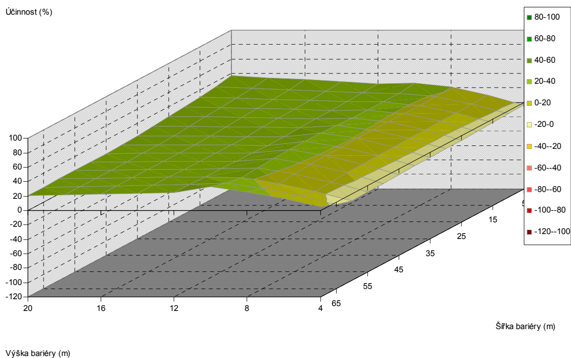
Obr. 5.322. Závislost účinnosti vegetační bariéry na výšce a šířce bariéry, pro vzdálenost od komunikace 80 m, jehličnaté dřeviny, PM10, 6 m nad povrchem
