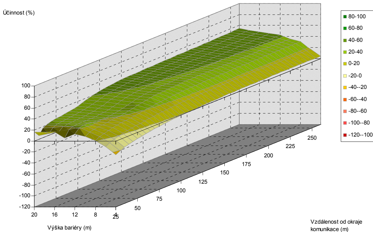
Obr. 5.58. Závislost účinnosti vegetační bariéry na výšce bariéry a vzdálenosti od komunikace, pro šířku bariéry 12 m, jehličnaté dřeviny, PM10, 6 m nad povrchem
