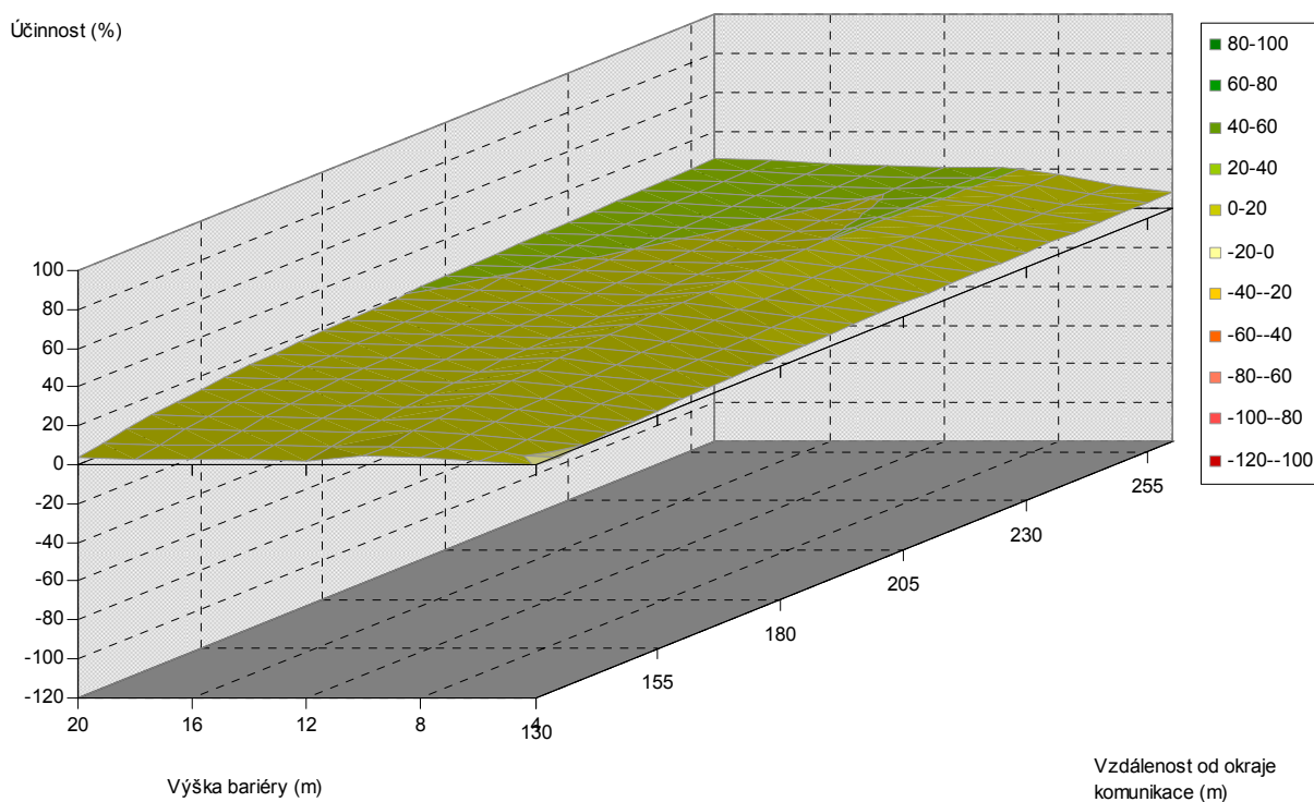
Obr. 5.56. Závislost účinnosti vegetační bariéry na výšce bariéry a vzdálenosti od komunikace, pro šířku bariéry 4 m, jehličnaté dřeviny, PM10, 6 m nad povrchem
