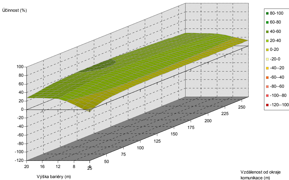
Obr. 5.112. Závislost účinnosti vegetační bariéry na výšce bariéry a vzdálenosti od komunikace, pro šířku bariéry 8 m, listnaté dřeviny, PM75, 6 m nad povrchem
