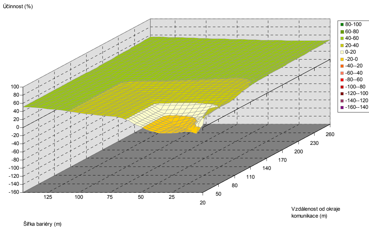
Obr. 5.190. Závislost účinnosti vegetační bariéry na šířce bariéry a vzdálenosti od komunikace, pro výšku bariéry 15 m, jehličnaté dřeviny, PM10, 6 m nad povrchem
