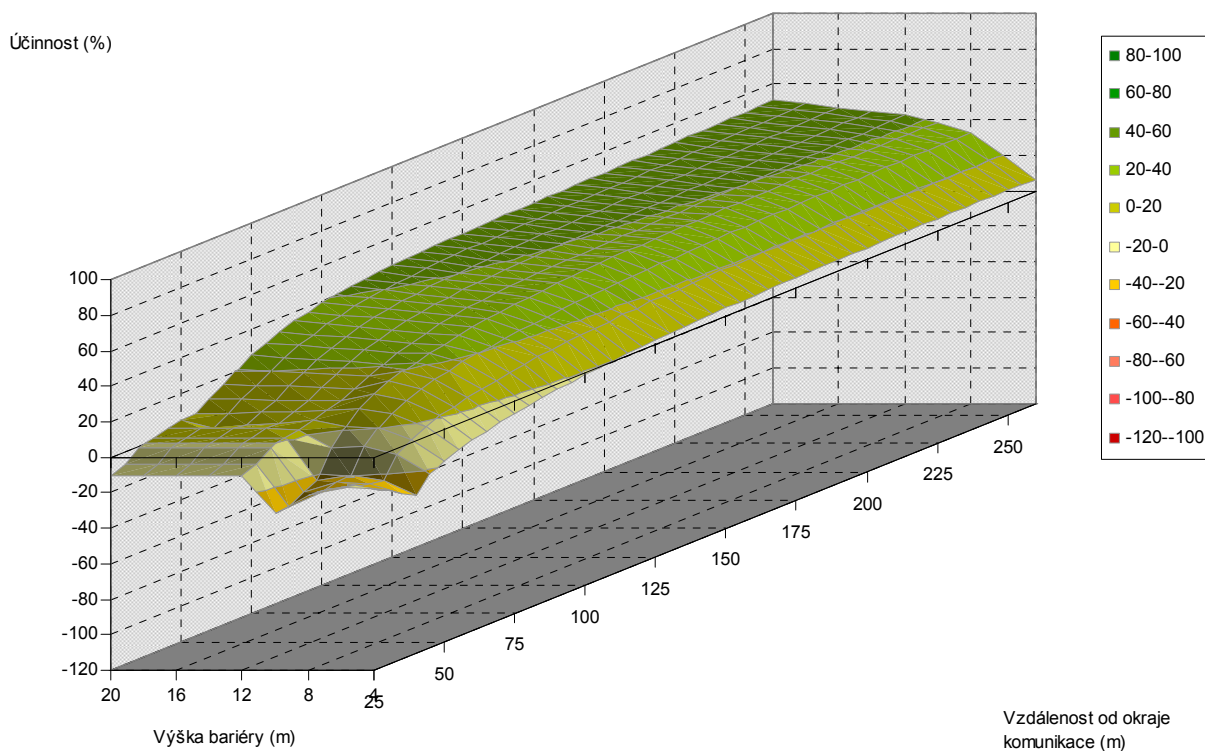
Obr. 5.60. Závislost účinnosti vegetační bariéry na výšce bariéry a vzdálenosti od komunikace, pro šířku bariéry 24 m, jehličnaté dřeviny, PM10, 6 m nad povrchem
