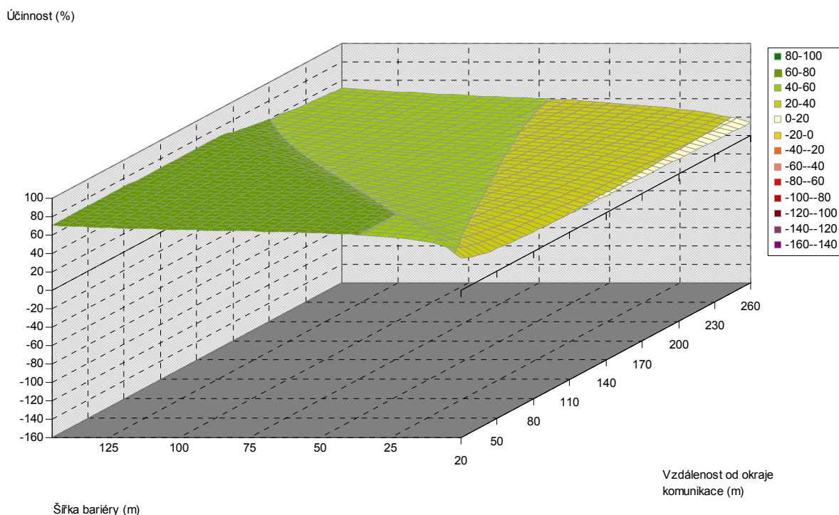
Obr. 5.204. Závislost účinnosti vegetační bariéry na šířce bariéry a vzdálenosti od komunikace, pro výšku bariéry 4 m, jehličnaté dřeviny, PM75, 1,5 m nad povrchem
