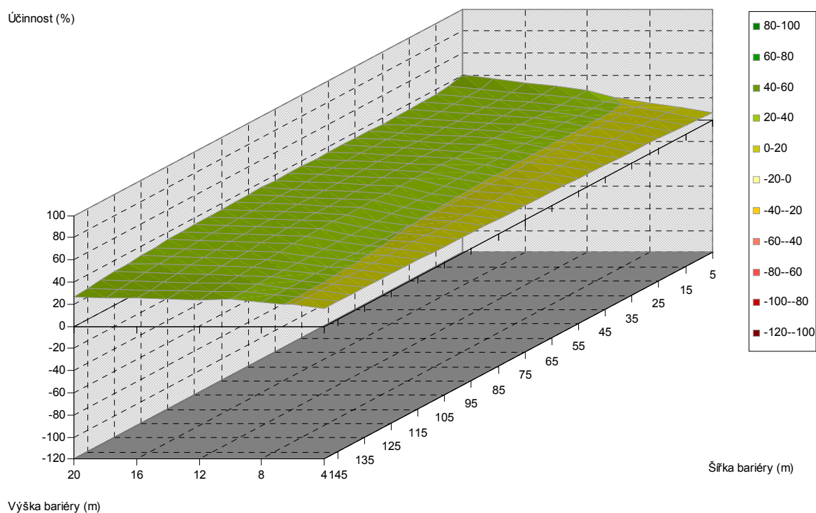
Obr. 5.288. Závislost účinnosti vegetační bariéry na výšce a šířce bariéry, pro vzdálenost od komunikace 180 m, listnaté dřeviny, PM10, 3 m nad povrchem
