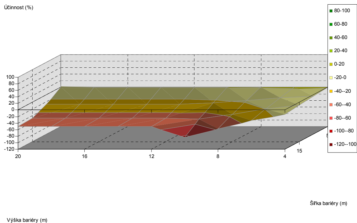
Obr. 5.280. Závislost účinnosti vegetační bariéry na výšce a šířce bariéry, pro vzdálenost od komunikace 30 m, listnaté dřeviny, PM10, 3 m nad povrchem
