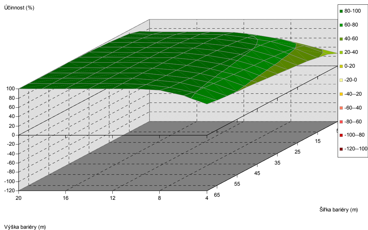
Obr. 5.374. Závislost účinnosti vegetační bariéry na výšce a šířce bariéry, pro vzdálenost od komunikace 80 m, jehličnaté dřeviny, PM75, 3 m nad povrchem
