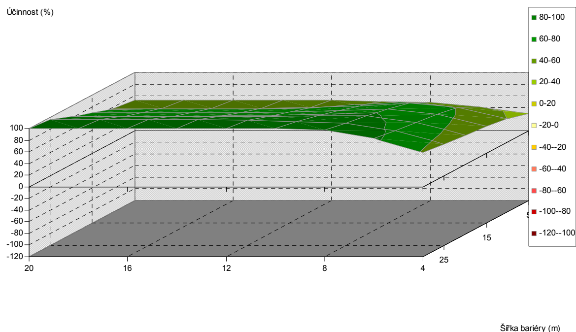
Obr. 5.372. Závislost účinnosti vegetační bariéry na výšce a šířce bariéry, pro vzdálenost od komunikace 40 m, jehličnaté dřeviny, PM75, 3 m nad povrchem
