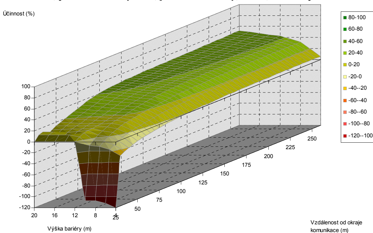
Obr. 5.58. Závislost účinnosti vegetační bariéry na výšce bariéry a vzdálenosti od komunikace, pro šířku bariéry 12 m, jehličnaté dřeviny, PM10, 6 m nad povrchem
