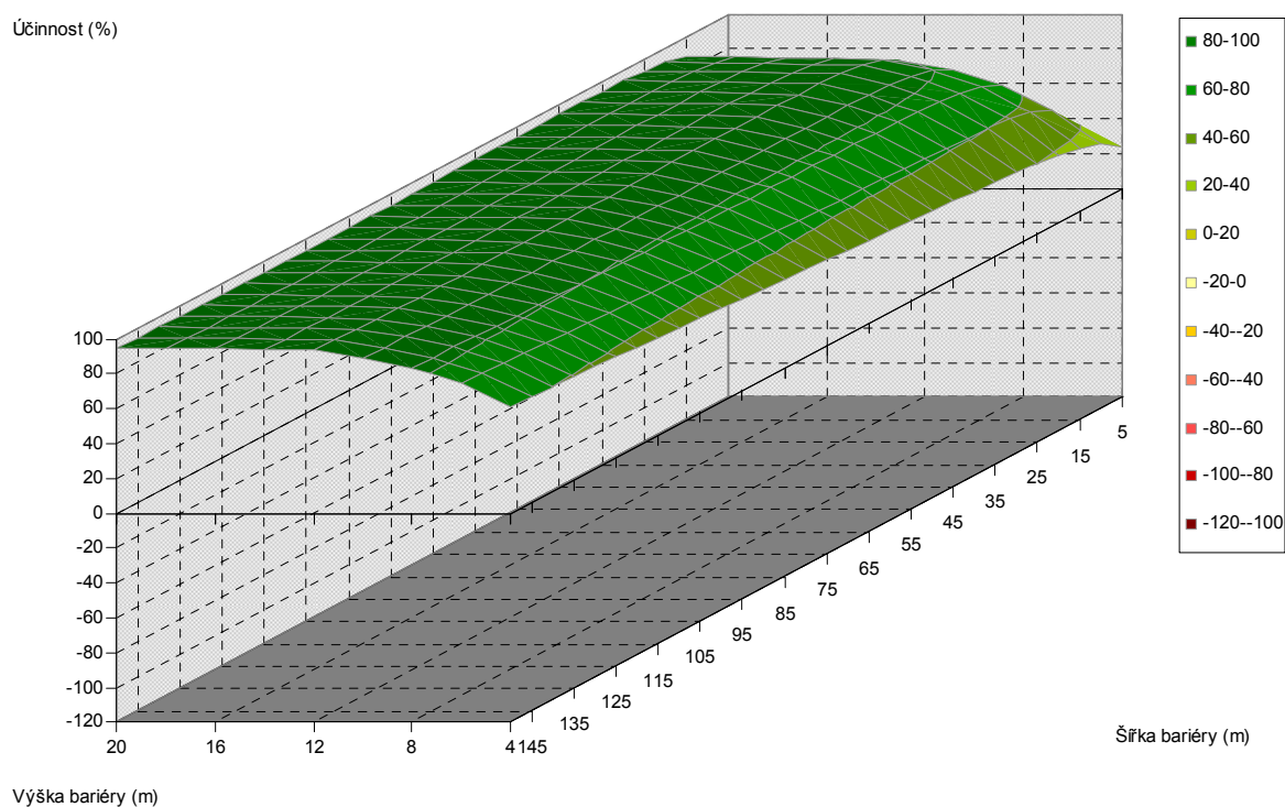
Obr. 5.380. Závislost účinnosti vegetační bariéry na výšce a šířce bariéry, pro vzdálenost od komunikace 200 m, jehličnaté dřeviny, PM75, 3 m nad povrchem
