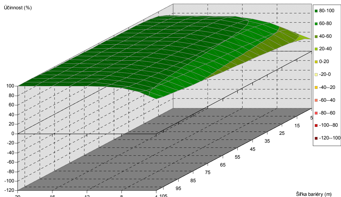
Obr. 5.376. Závislost účinnosti vegetační bariéry na výšce a šířce bariéry, pro vzdálenost od komunikace 120 m, jehličnaté dřeviny, PM75, 3 m nad povrchem
