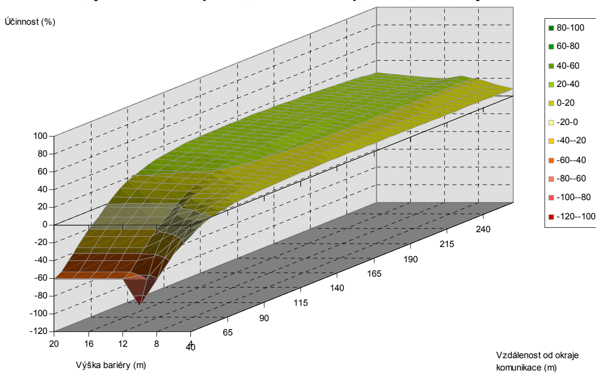
Obr. 5.28. Závislost účinnosti vegetační bariéry na výšce bariéry a vzdálenosti od komunikace, pro šířku bariéry 30 m, listnaté dřeviny, PM10, 3 m nad povrchem
