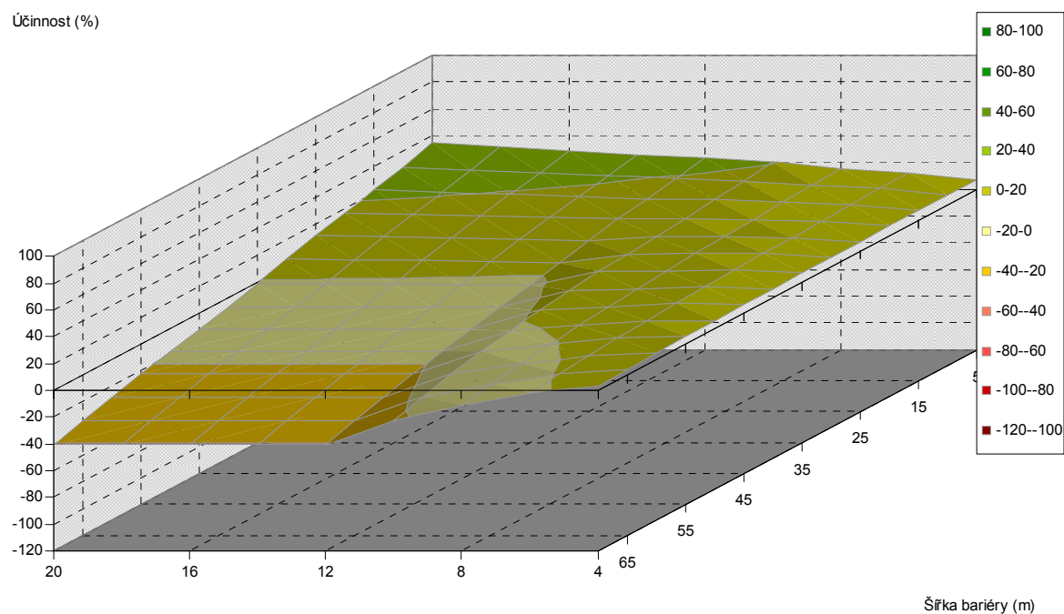
Obr. 5.283. Závislost účinnosti vegetační bariéry na výšce a šířce bariéry, pro vzdálenost od komunikace 80 m, listnaté dřeviny, PM10, 3 m nad povrchem
