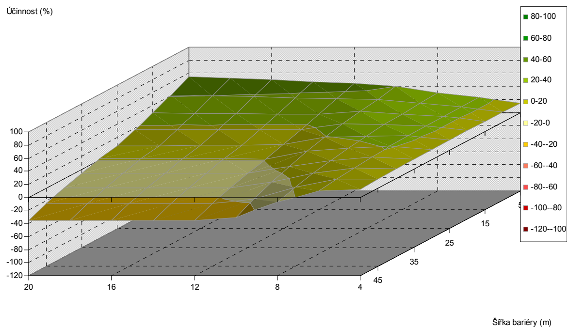
Obr. 5.295. Závislost účinnosti vegetační bariéry na výšce a šířce bariéry, pro vzdálenost od komunikace 60 m, jehličnaté dřeviny, PM10, 3 m nad povrchem
