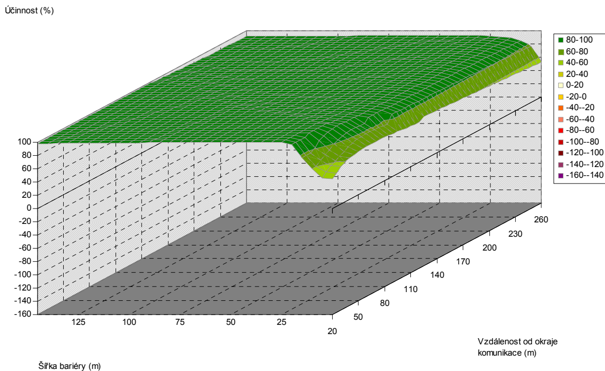
Obr. 5.212. Závislost účinnosti vegetační bariéry na šířce bariéry a vzdálenosti od komunikace, pro výšku bariéry 20 m, jehličnaté dřeviny, PM75, 1,5 m nad povrchem
