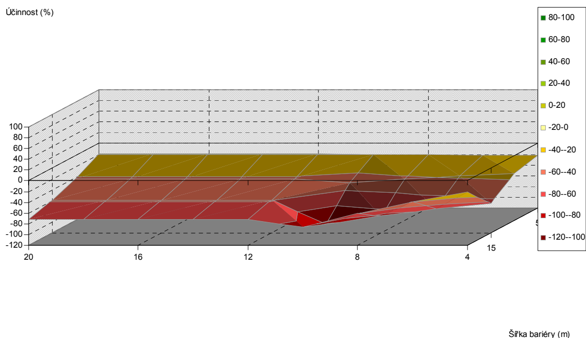
Obr. 5.306. Závislost účinnosti vegetační bariéry na výšce a šířce bariéry, pro vzdálenost od komunikace 30 m, listnaté dřeviny, PM10, 6 m nad povrchem
