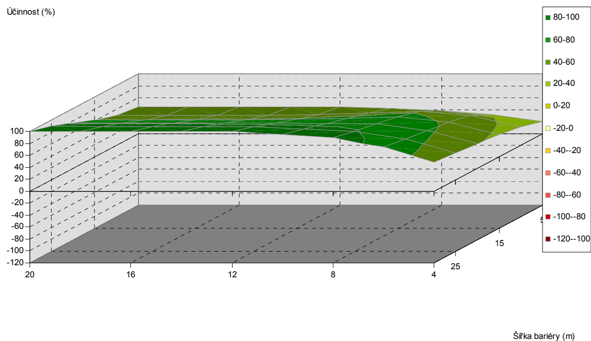
Obr. 5.359. Závislost účinnosti vegetační bariéry na výšce a šířce bariéry, pro vzdálenost od komunikace 40 m, listnaté dřeviny, PM75, 3 m nad povrchem
