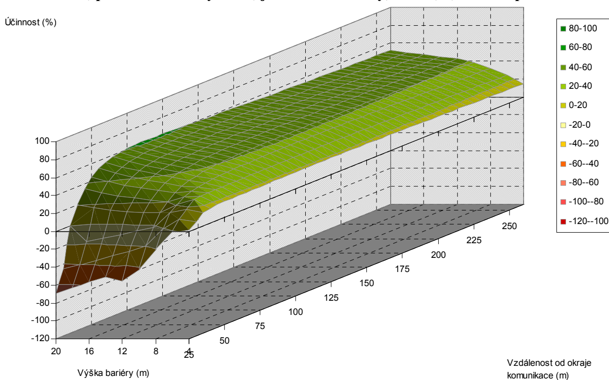
Obr. 5.14. Závislost účinnosti vegetační bariéry na výšce bariéry a vzdálenosti od komunikace, pro šířku bariéry 12 m, jehličnaté dřeviny, PM10, 1,5 m nad povrchem
