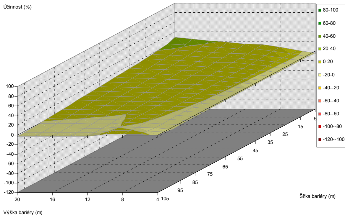
Obr. 5.312. Závislost účinnosti vegetační bariéry na výšce a šířce bariéry, pro vzdálenost od komunikace 140 m, listnaté dřeviny, PM10, 6 m nad povrchem
