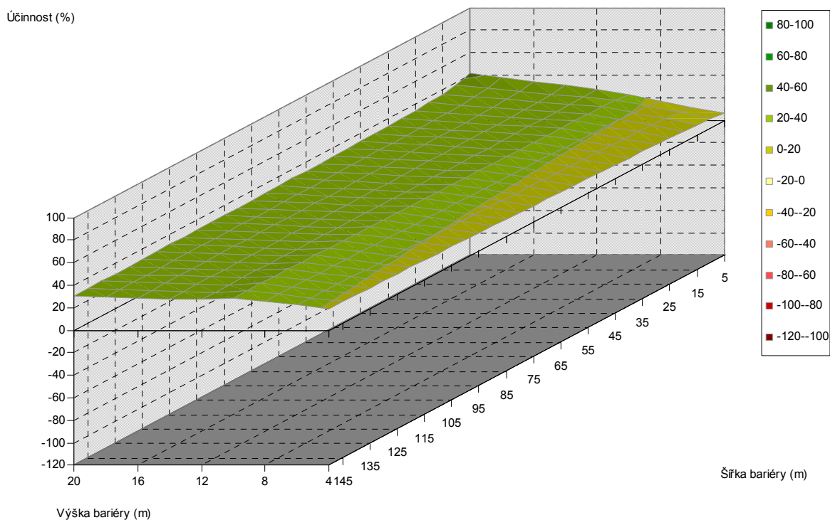
Obr. 5.262. Závislost účinnosti vegetační bariéry na výšce a šířce bariéry, pro vzdálenost od komunikace 180 m, listnaté dřeviny, PM10, 1,5 m nad povrchem
