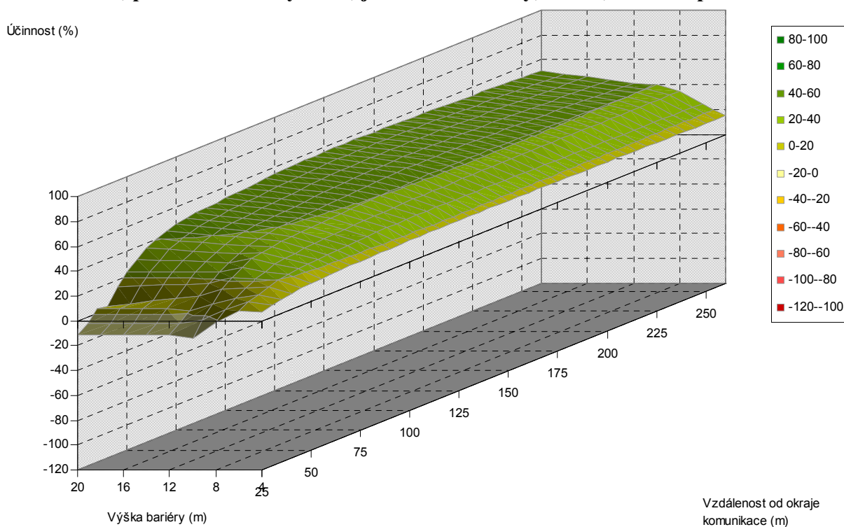
Obr. 5.36. Závislost účinnosti vegetační bariéry na výšce bariéry a vzdálenosti od komunikace, pro šířku bariéry 12 m, jehličnaté dřeviny, PM10, 3 m nad povrchem
