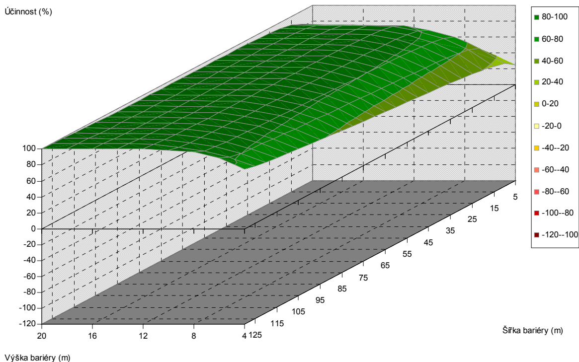
Obr. 5.378. Závislost účinnosti vegetační bariéry na výšce a šířce bariéry, pro vzdálenost od komunikace 160 m, jehličnaté dřeviny, PM75, 3 m nad povrchem
