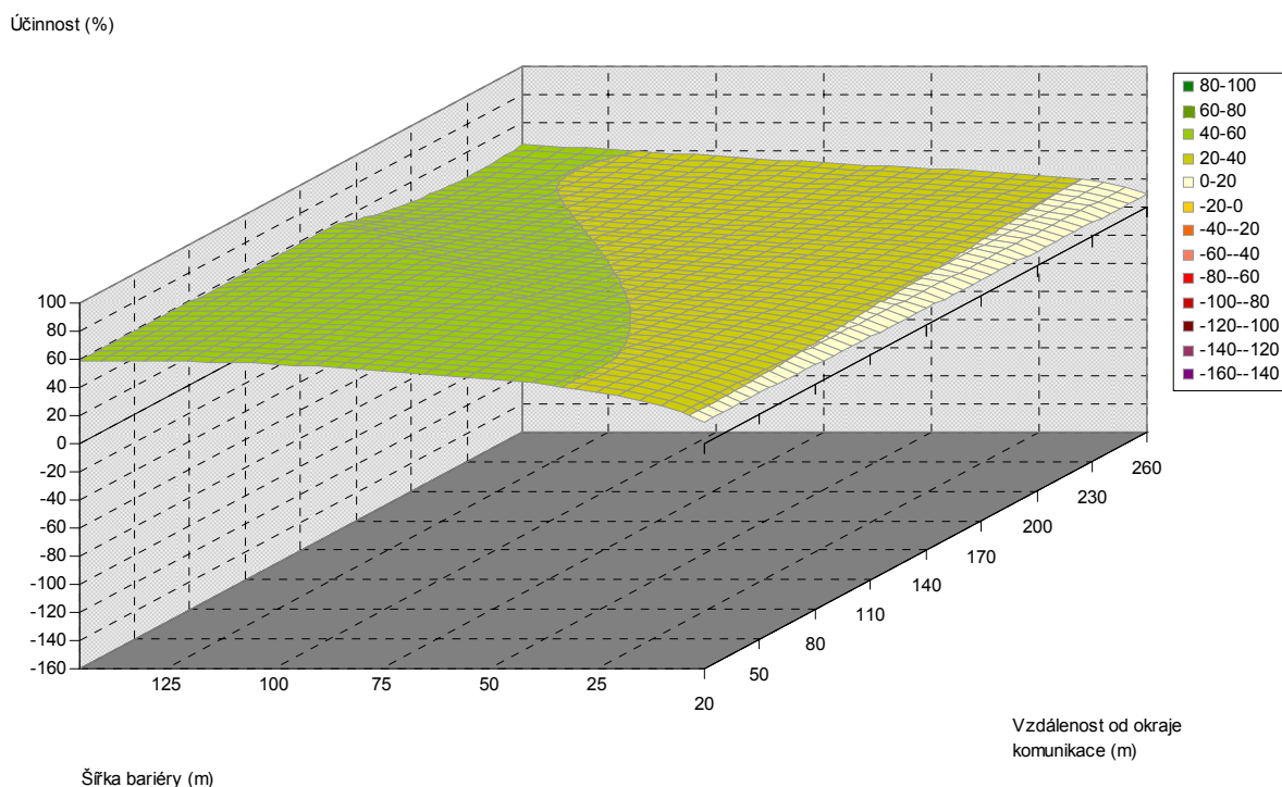
Obr. 5.214. Závislost účinnosti vegetační bariéry na šířce bariéry a vzdálenosti od komunikace, pro výšku bariéry 4 m, listnaté dřeviny, PM75, 3 m nad povrchem
