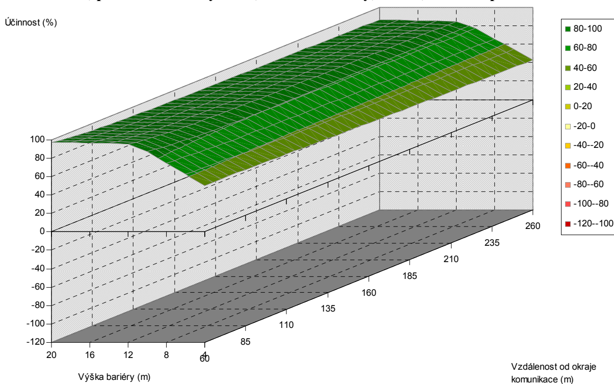
Obr. 5.118. Závislost účinnosti vegetační bariéry na výšce bariéry a vzdálenosti od komunikace, pro šířku bariéry 50 m, listnaté dřeviny, PM75, 6 m nad povrchem
