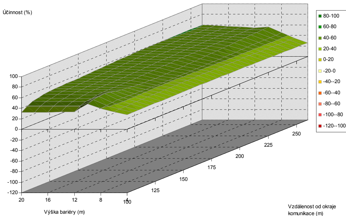
Obr. 5.44. Závislost účinnosti vegetační bariéry na výšce bariéry a vzdálenosti od komunikace, pro šířku bariéry 120 m, jehličnaté dřeviny, PM10, 3 m nad povrchem
