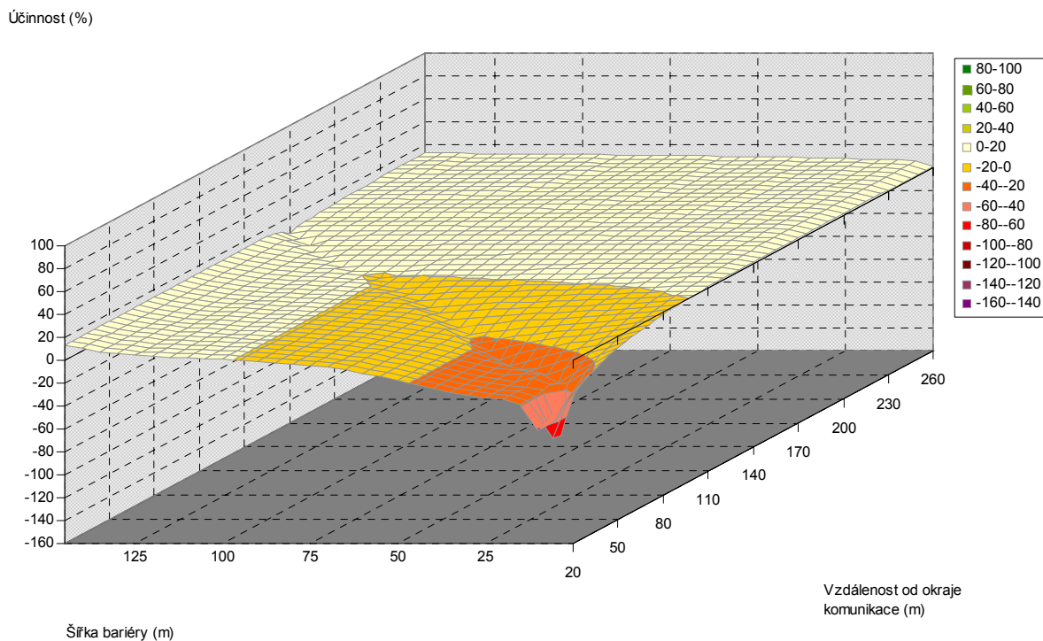
Obr. 5.176. Závislost účinnosti vegetační bariéry na šířce bariéry a vzdálenosti od komunikace, pro výšku bariéry 6 m, listnaté dřeviny, PM10, 6 m nad povrchem
