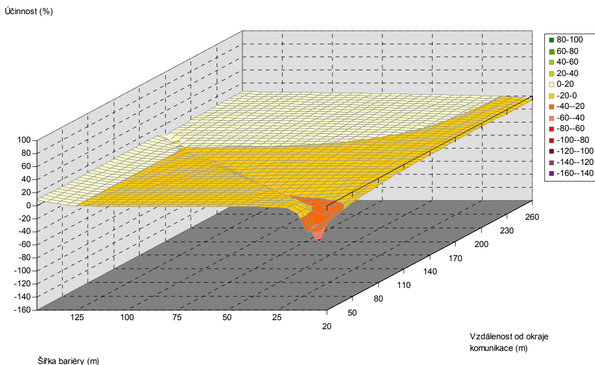
Obr. 5.184. Závislost účinnosti vegetační bariéry na šířce bariéry a vzdálenosti od komunikace, pro výšku bariéry 4 m, jehličnaté dřeviny, PM10, 6 m nad povrchem
