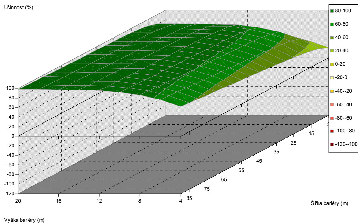
Obr. 5.336. Závislost účinnosti vegetační bariéry na výšce a šířce bariéry, pro vzdálenost od komunikace 100 m, listnaté dřeviny, PM75, 1,5 m nad povrchem
