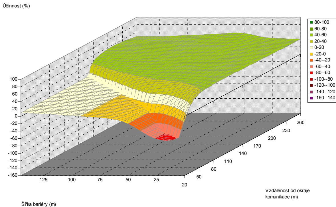
Obr. 5.148. Závislost účinnosti vegetační bariéry na šířce bariéry a vzdálenosti od komunikace, pro výšku bariéry 11 m, jehličnaté dřeviny, PM10, 1,5 m nad povrchem
