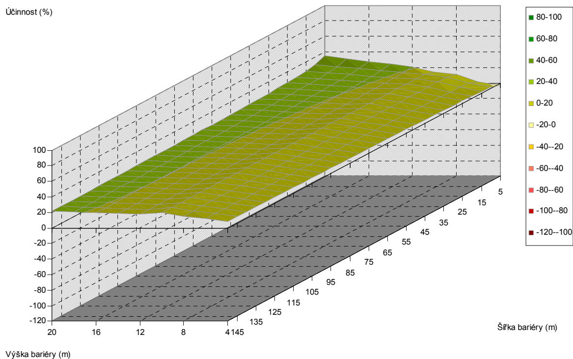
Obr. 5.316. Závislost účinnosti vegetační bariéry na výšce a šířce bariéry, pro vzdálenost od komunikace 220 m, listnaté dřeviny, PM10, 6 m nad povrchem
