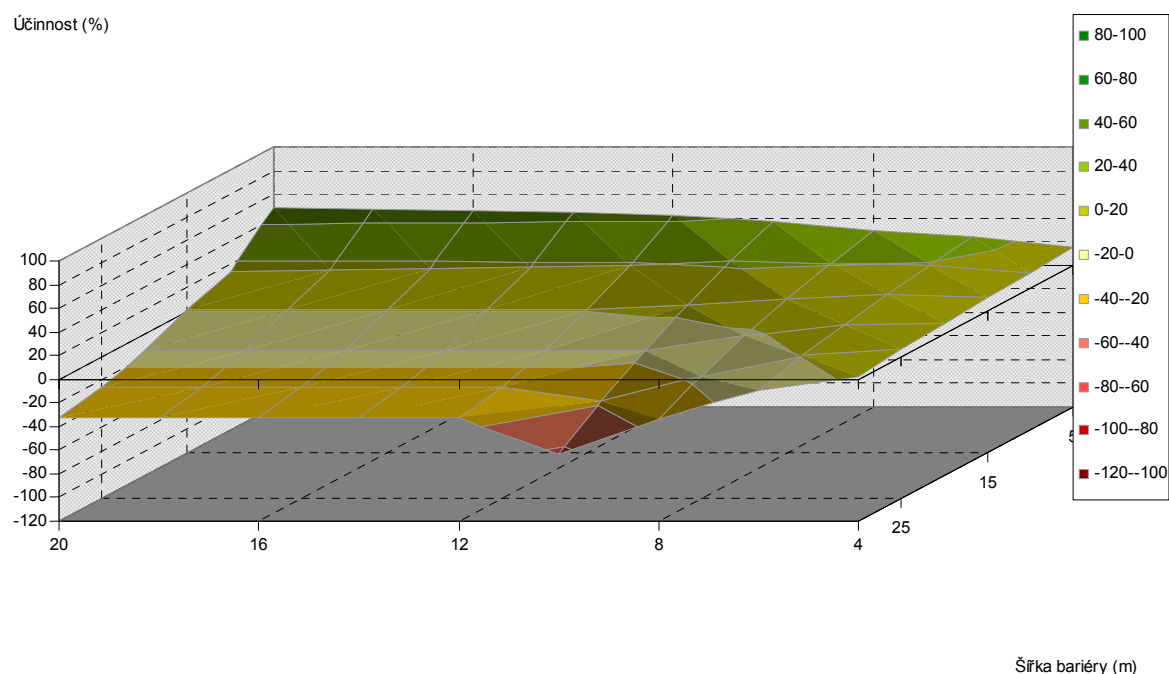
Obr. 5.294. Závislost účinnosti vegetační bariéry na výšce a šířce bariéry, pro vzdálenost od komunikace 40 m, jehličnaté dřeviny, PM10, 3 m nad povrchem
