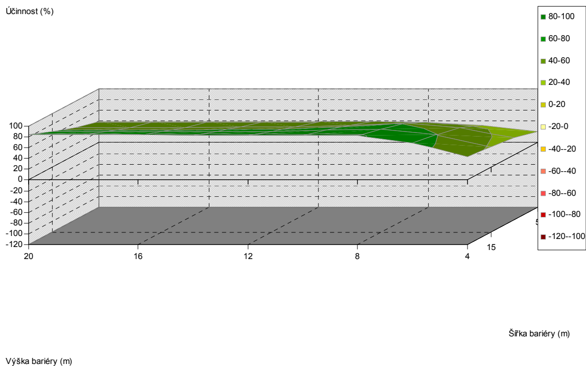
Obr. 5.358. Závislost účinnosti vegetační bariéry na výšce a šířce bariéry, pro vzdálenost od komunikace 30 m, listnaté dřeviny, PM75, 3 m nad povrchem
