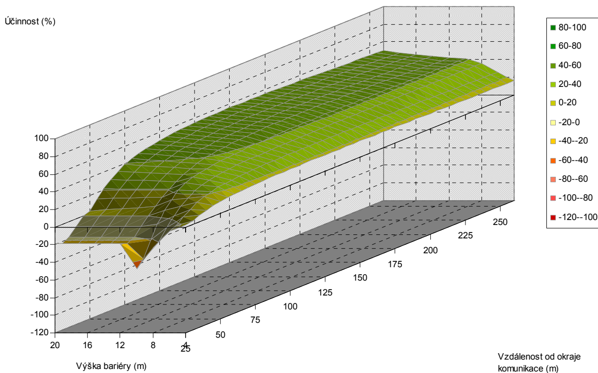
Obr. 5.38. Závislost účinnosti vegetační bariéry na výšce bariéry a vzdálenosti od komunikace, pro šířku bariéry 24 m, jehličnaté dřeviny, PM10, 3 m nad povrchem
