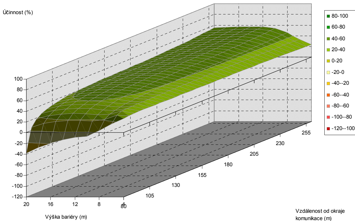
Obr. 5.20. Závislost účinnosti vegetační bariéry na výšce bariéry a vzdálenosti od komunikace, pro šířku bariéry 70 m, jehličnaté dřeviny, PM10, 1,5 m nad povrchem
