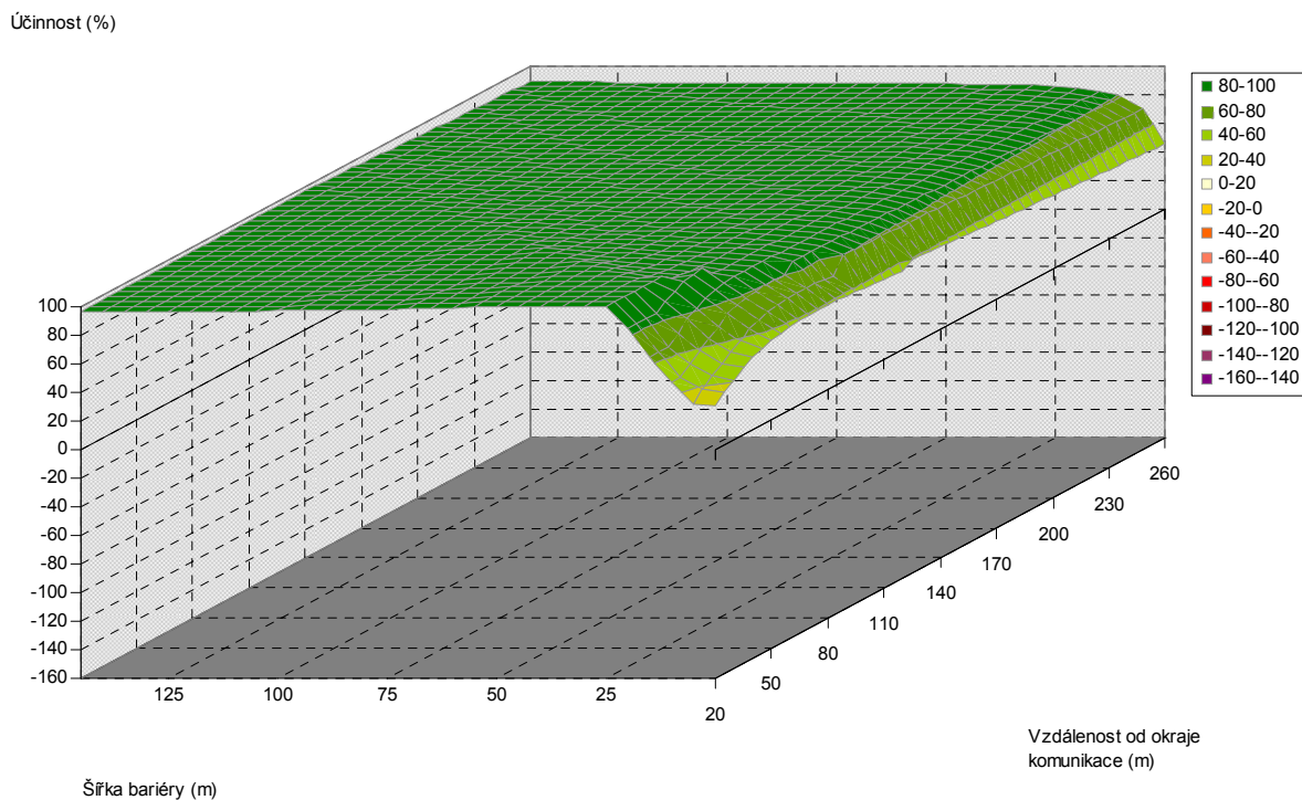
Obr. 5.200. Závislost účinnosti vegetační bariéry na šířce bariéry a vzdálenosti od komunikace, pro výšku bariéry 15 m, listnaté dřeviny, PM75, 1,5 m nad povrchem
