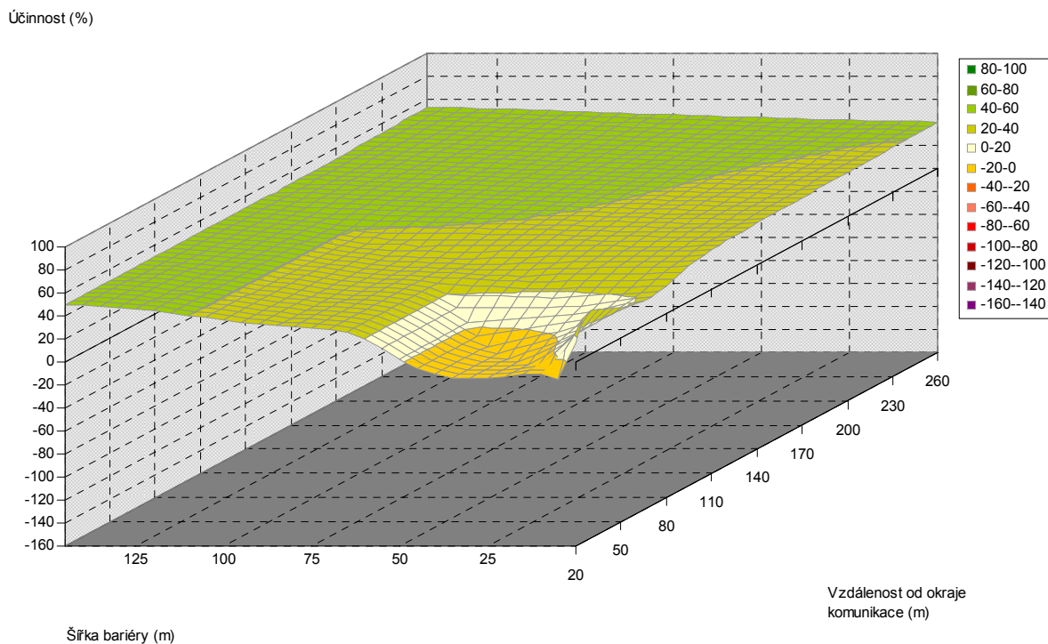
Obr. 5.188. Závislost účinnosti vegetační bariéry na šířce bariéry a vzdálenosti od komunikace, pro výšku bariéry 11 m, jehličnaté dřeviny, PM10, 6 m nad povrchem
