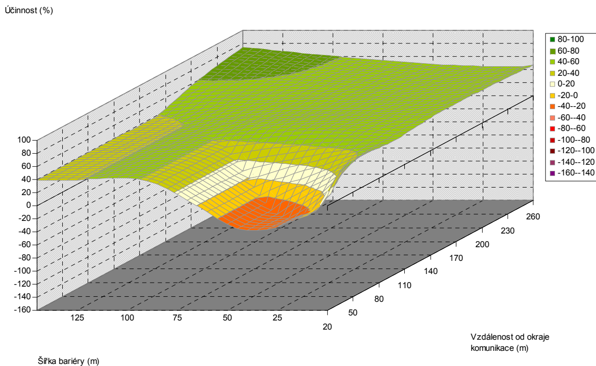
Obr. 5.170. Závislost účinnosti vegetační bariéry na šířce bariéry a vzdálenosti od komunikace, pro výšku bariéry 15 m, jehličnaté dřeviny, PM10, 3 m nad povrchem
