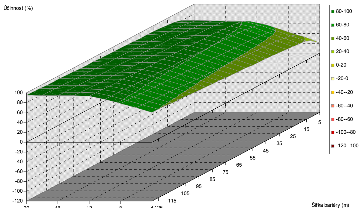
Obr. 5.390. Závislost účinnosti vegetační bariéry na výšce a šířce bariéry, pro vzdálenost od komunikace 140 m, listnaté dřeviny, PM75, 6 m nad povrchem
