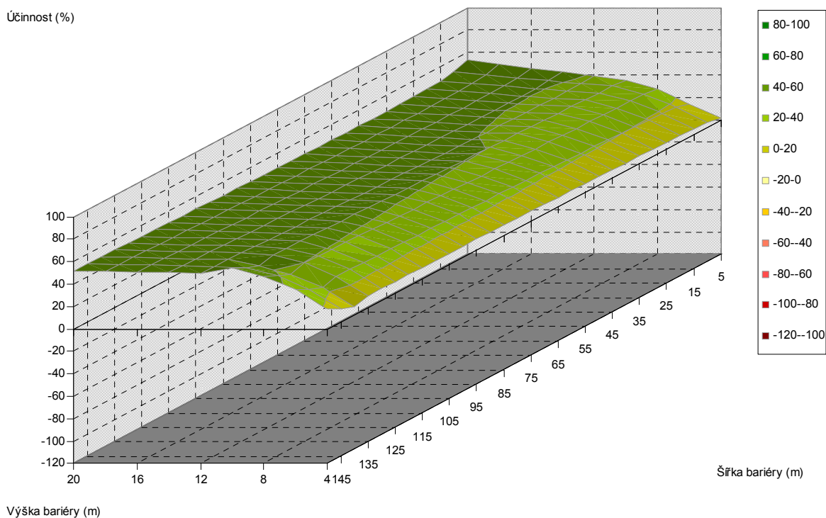
Obr. 5.326. Závislost účinnosti vegetační bariéry na výšce a šířce bariéry, pro vzdálenost od komunikace 160 m, jehličnaté dřeviny, PM10, 6 m nad povrchem
