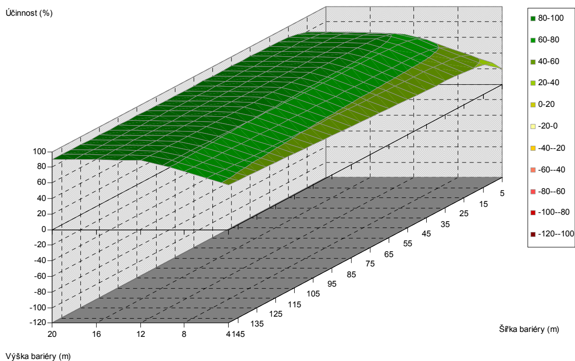
Obr. 5.394. Závislost účinnosti vegetační bariéry na výšce a šířce bariéry, pro vzdálenost od komunikace 220 m, listnaté dřeviny, PM75, 6 m nad povrchem
