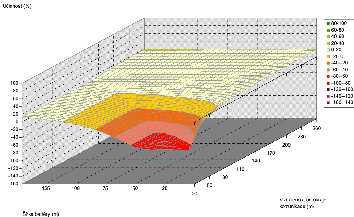
Obr. 5.178. Závislost účinnosti vegetační bariéry na šířce bariéry a vzdálenosti od komunikace, pro výšku bariéry 11 m, listnaté dřeviny, PM10, 6 m nad povrchem
