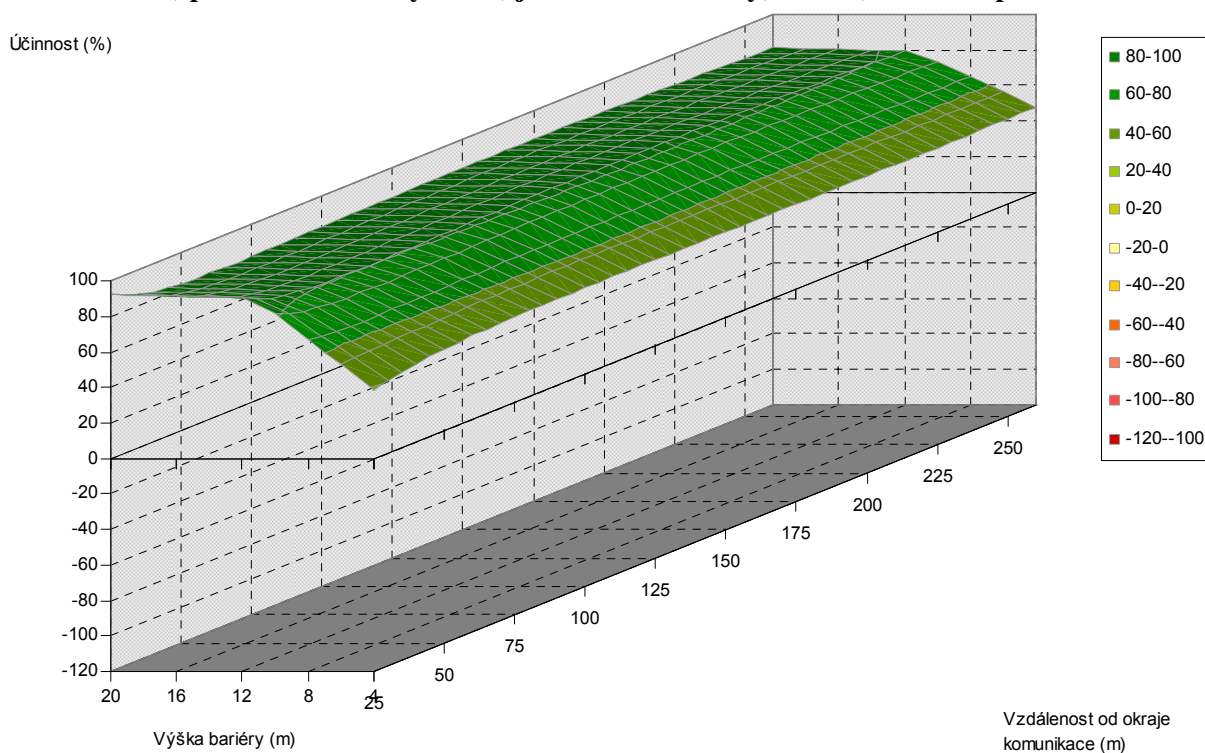
Obr. 5.124. Závislost účinnosti vegetační bariéry na výšce bariéry a vzdálenosti od komunikace, pro šířku bariéry 12 m, jehličnaté dřeviny, PM75, 6 m nad povrchem
