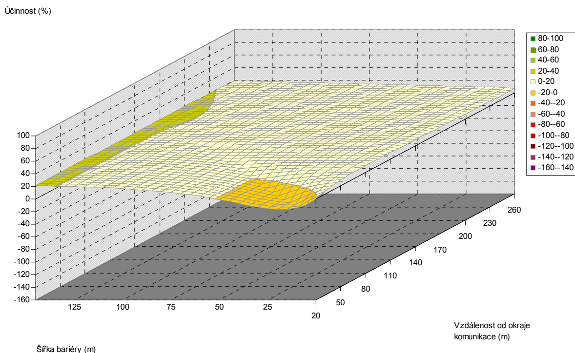
Obr. 5.136. Závislost účinnosti vegetační bariéry na šířce bariéry a vzdálenosti od komunikace, pro výšku bariéry 6 m, listnaté dřeviny, PM10, 1,5 m nad povrchem
