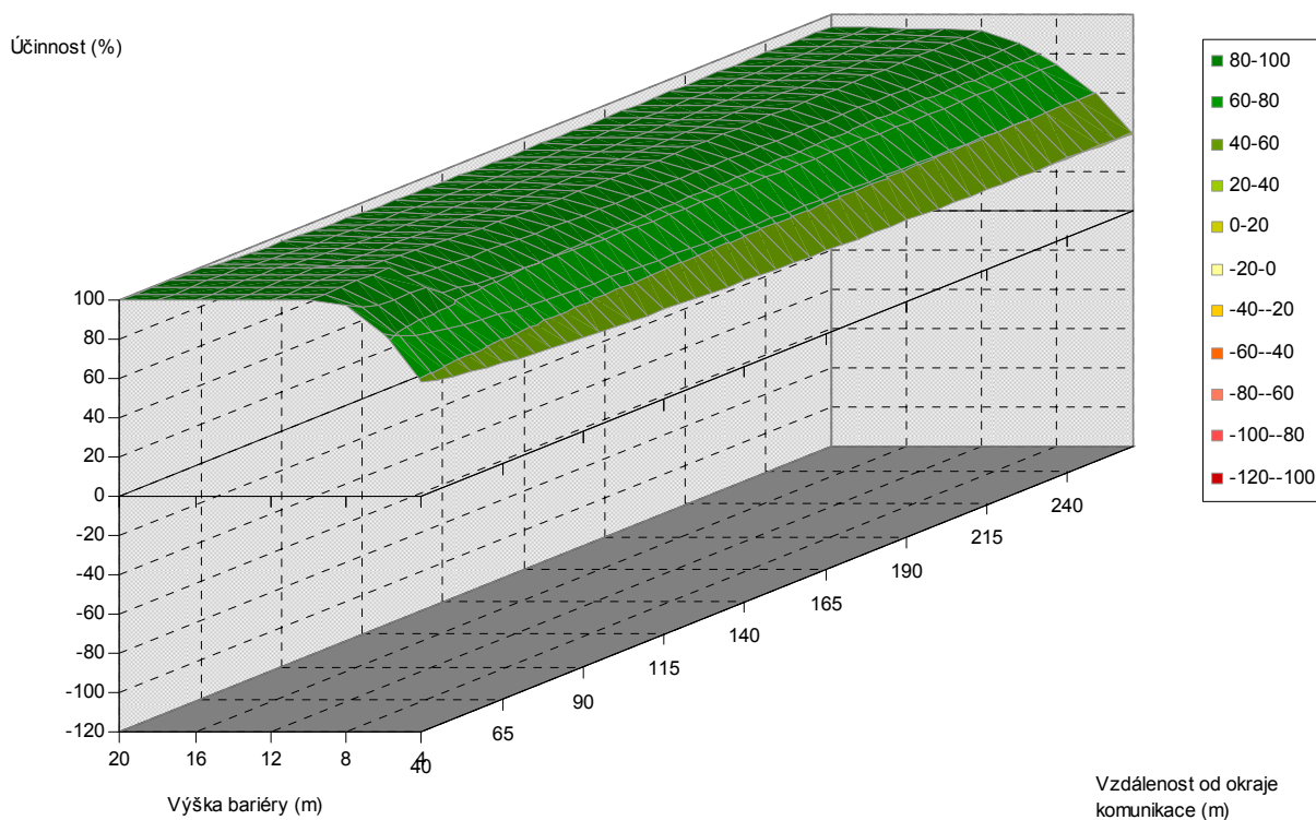
Obr. 5.106. Závislost účinnosti vegetační bariéry na výšce bariéry a vzdálenosti od komunikace, pro šířku bariéry 40 m, jehličnaté dřeviny, PM75, 3 m nad povrchem
