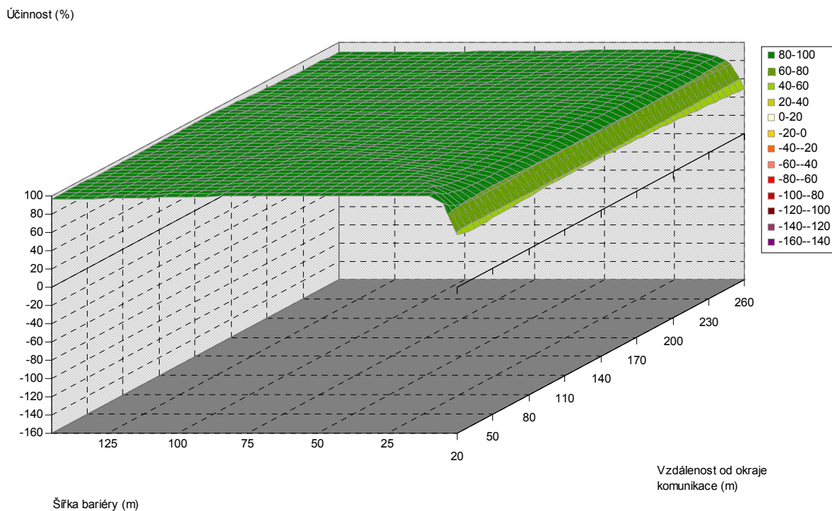
Obr. 5.252. Závislost účinnosti vegetační bariéry na šířce bariéry a vzdálenosti od komunikace, pro výšku bariéry 20 m, jehličnaté dřeviny, PM75, 6 m nad povrchem
