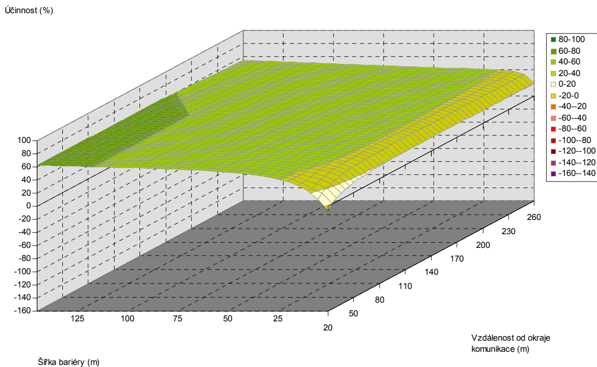
Obr. 5.234. Závislost účinnosti vegetační bariéry na šířce bariéry a vzdálenosti od komunikace, pro výšku bariéry 4 m, listnaté dřeviny, PM75, 6 m nad povrchem
