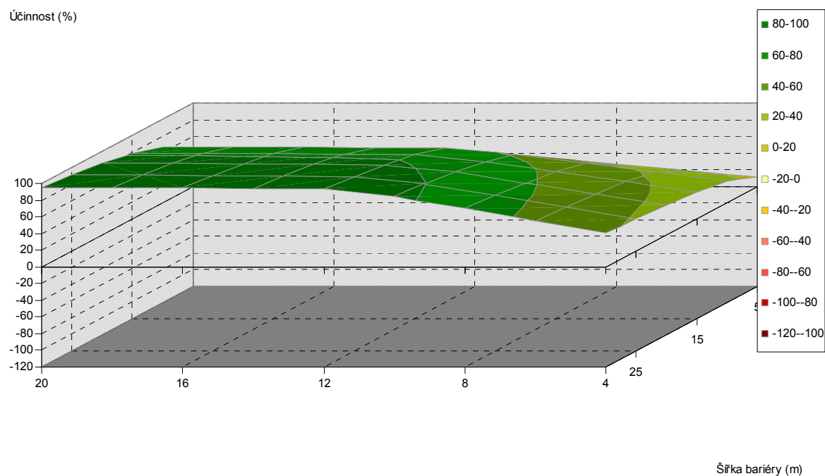
Obr. 5.385. Závislost účinnosti vegetační bariéry na výšce a šířce bariéry, pro vzdálenost od komunikace 40 m, listnaté dřeviny, PM75, 6 m nad povrchem
