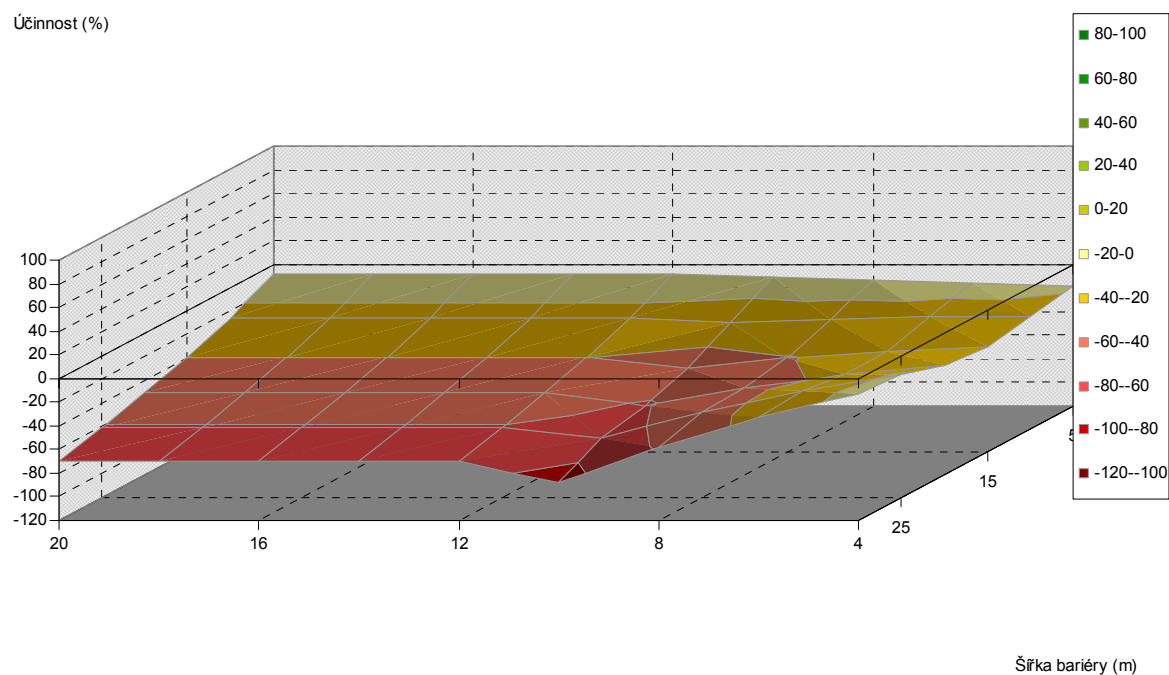
Obr. 5.307. Závislost účinnosti vegetační bariéry na výšce a šířce bariéry, pro vzdálenost od komunikace 40 m, listnaté dřeviny, PM10, 6 m nad povrchem
