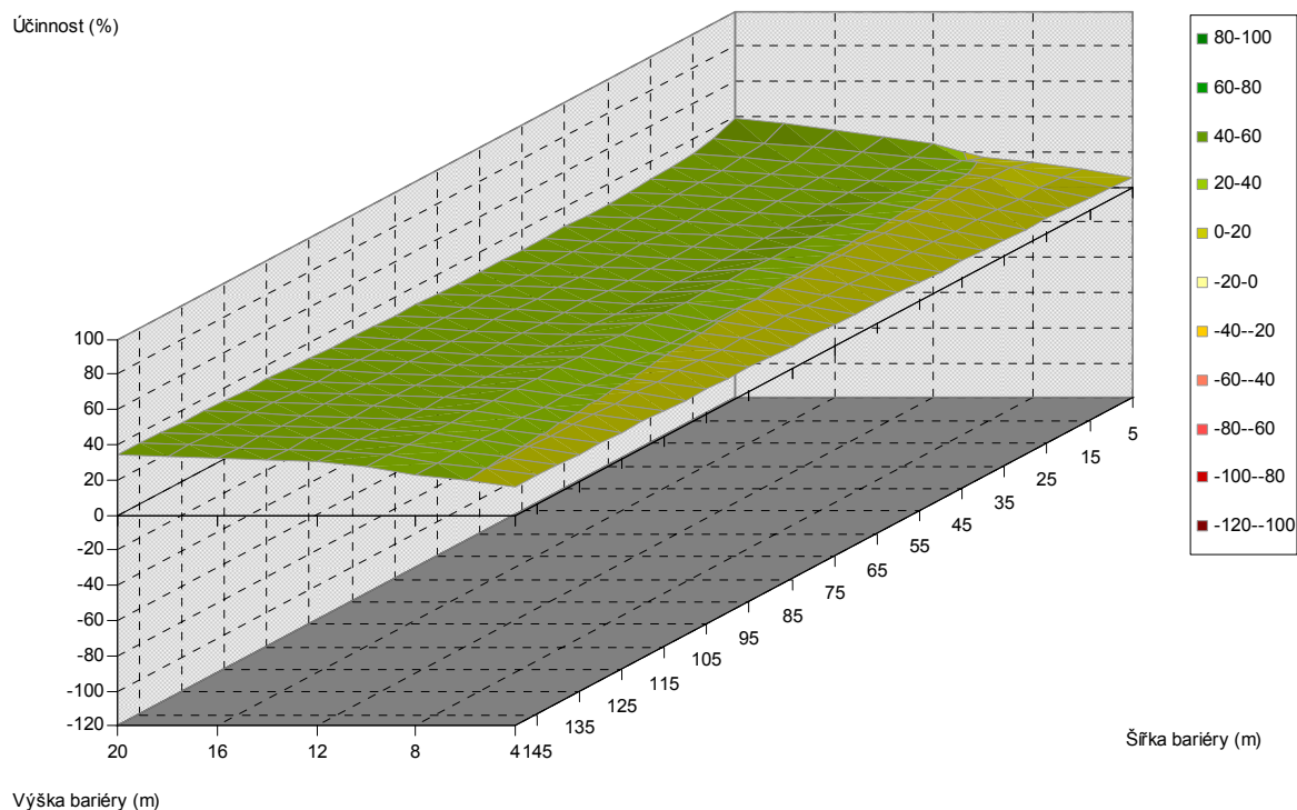
Obr. 5.292. Závislost účinnosti vegetační bariéry na výšce a šířce bariéry, pro vzdálenost od komunikace 20 m, jehličnaté dřeviny, PM10, 3 m nad povrchem
