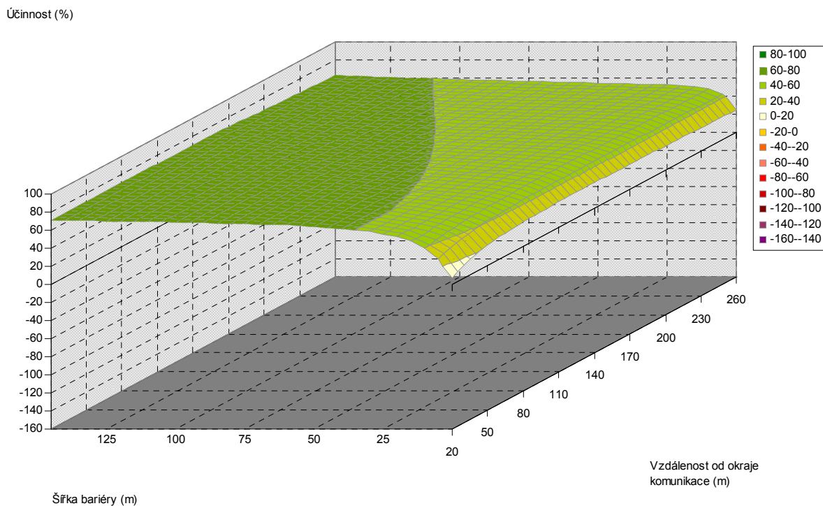
Obr. 5.236. Závislost účinnosti vegetační bariéry na šířce bariéry a vzdálenosti od komunikace, pro výšku bariéry 6 m, listnaté dřeviny, PM75, 6 m nad povrchem
