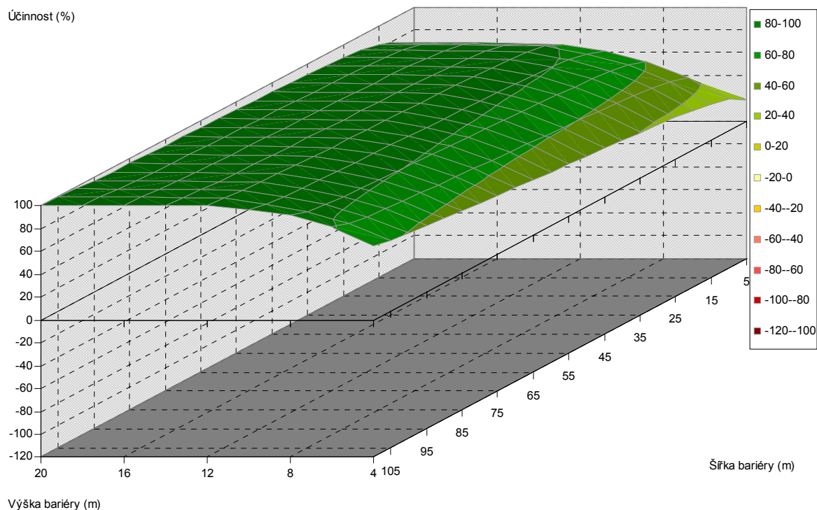
Obr. 5.364. Závislost účinnosti vegetační bariéry na výšce a šířce bariéry, pro vzdálenost od komunikace 140 m, listnaté dřeviny, PM75, 3 m nad povrchem
