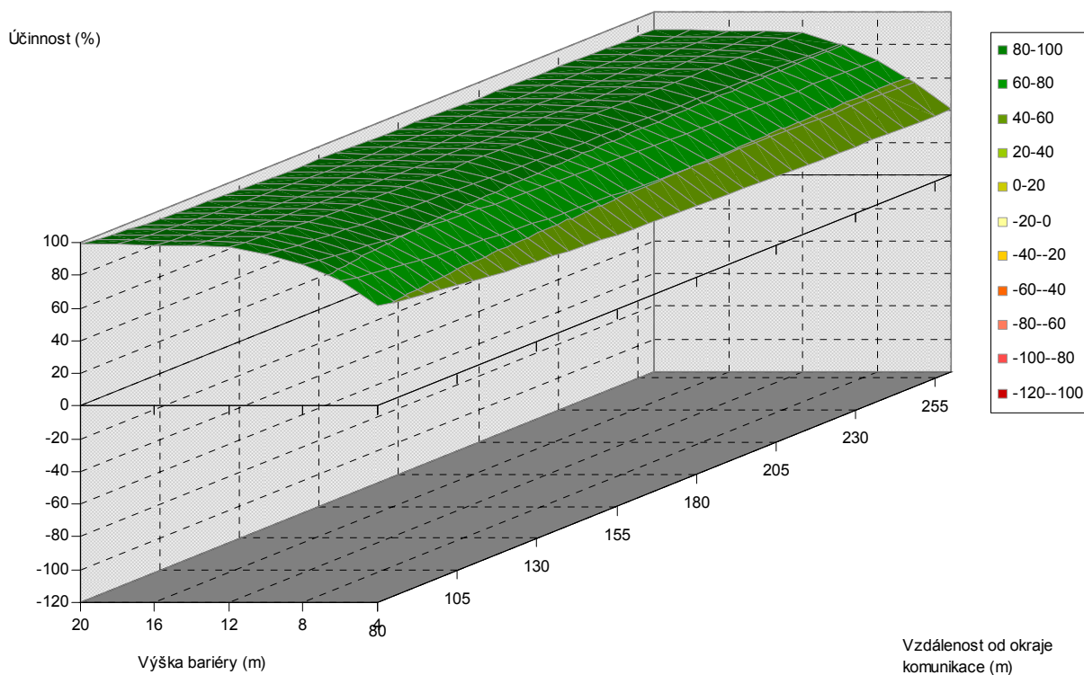
Obr. 5.76. Závislost účinnosti vegetační bariéry na výšce bariéry a vzdálenosti od komunikace, pro šířku bariéry 90 m, listnaté dřeviny, PM75, 1,5 m nad povrchem
