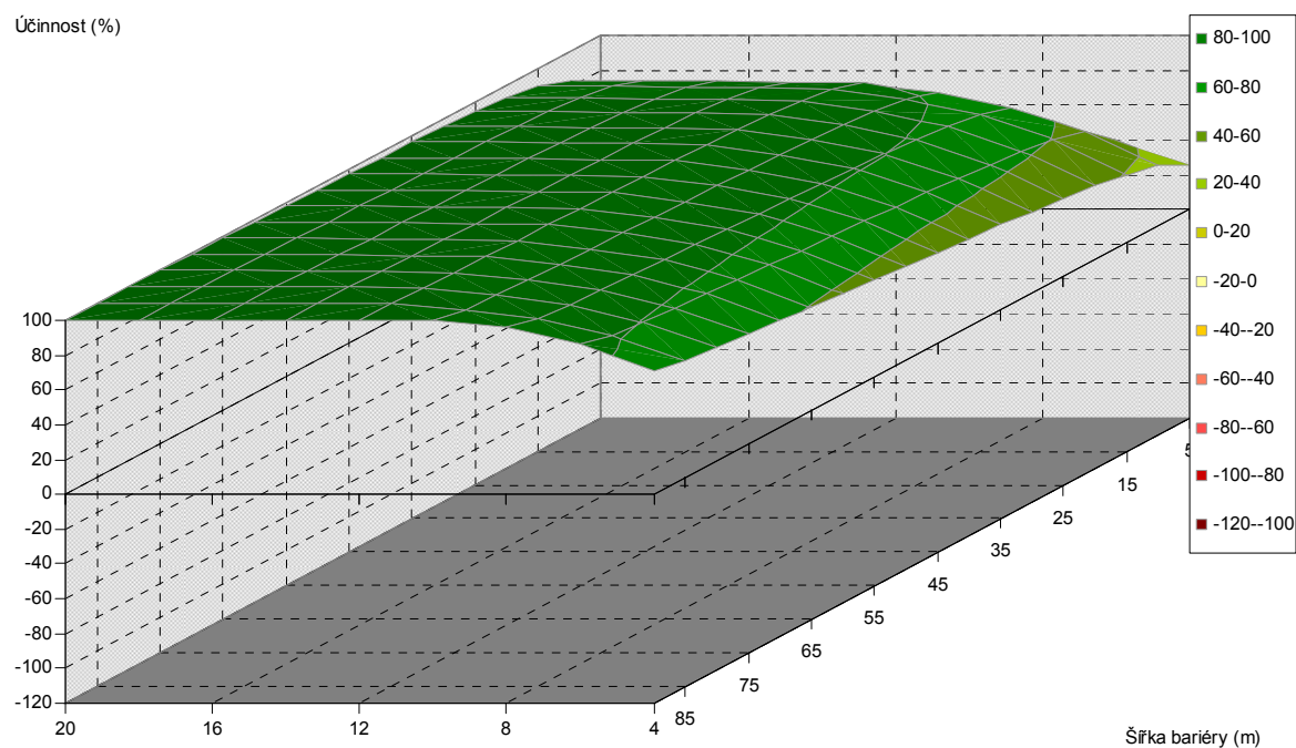
Obr. 5.375. Závislost účinnosti vegetační bariéry na výšce a šířce bariéry, pro vzdálenost od komunikace 100 m, jehličnaté dřeviny, PM75, 3 m nad povrchem
