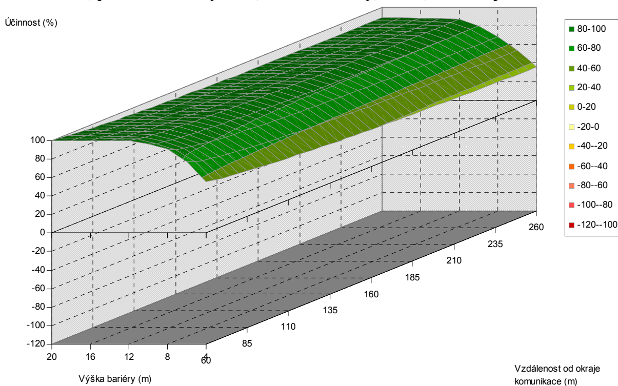
Obr. 5.96. Závislost účinnosti vegetační bariéry na výšce bariéry a vzdálenosti od komunikace, pro šířku bariéry 50 m, listnaté dřeviny, PM75, 3 m nad povrchem
