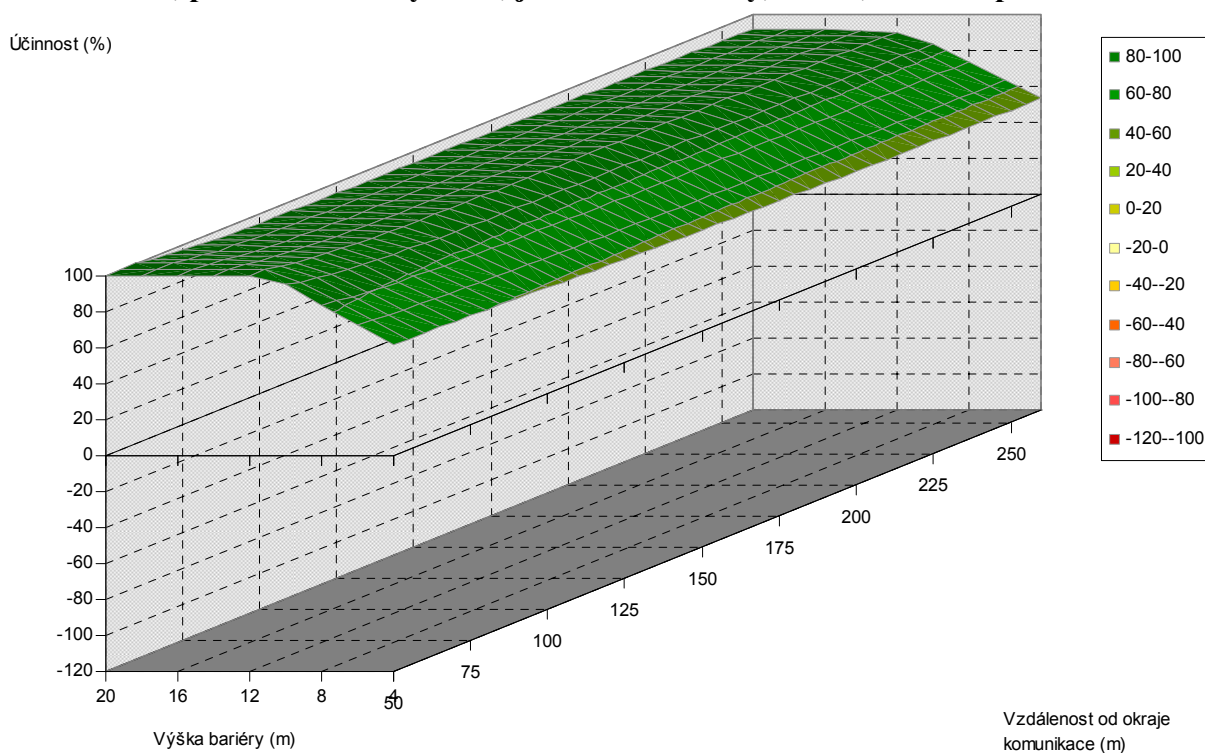
Obr. 5.128. Závislost účinnosti vegetační bariéry na výšce bariéry a vzdálenosti od komunikace, pro šířku bariéry 40 m, jehličnaté dřeviny, PM75, 6 m nad povrchem
