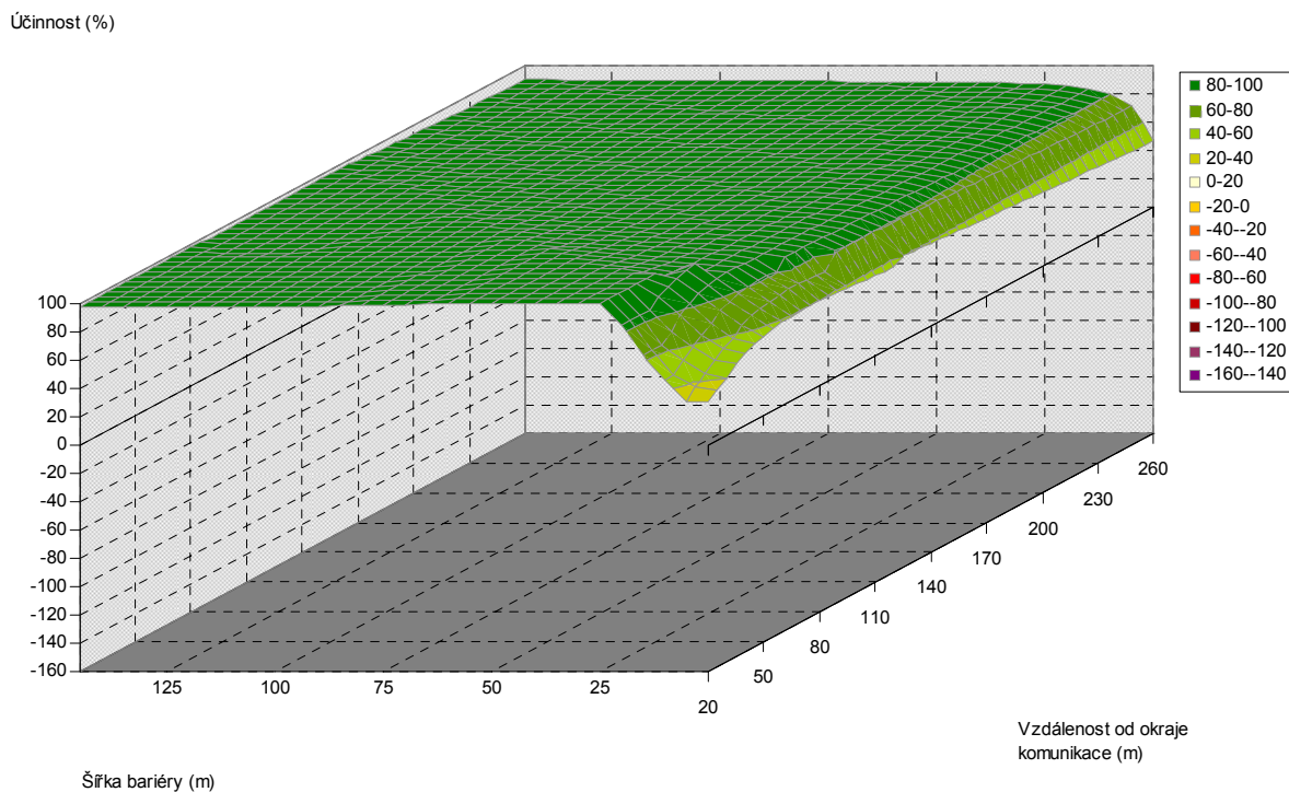
Obr. 5.202. Závislost účinnosti vegetační bariéry na šířce bariéry a vzdálenosti od komunikace, pro výšku bariéry 20 m, listnaté dřeviny, PM75, 1,5 m nad povrchem
