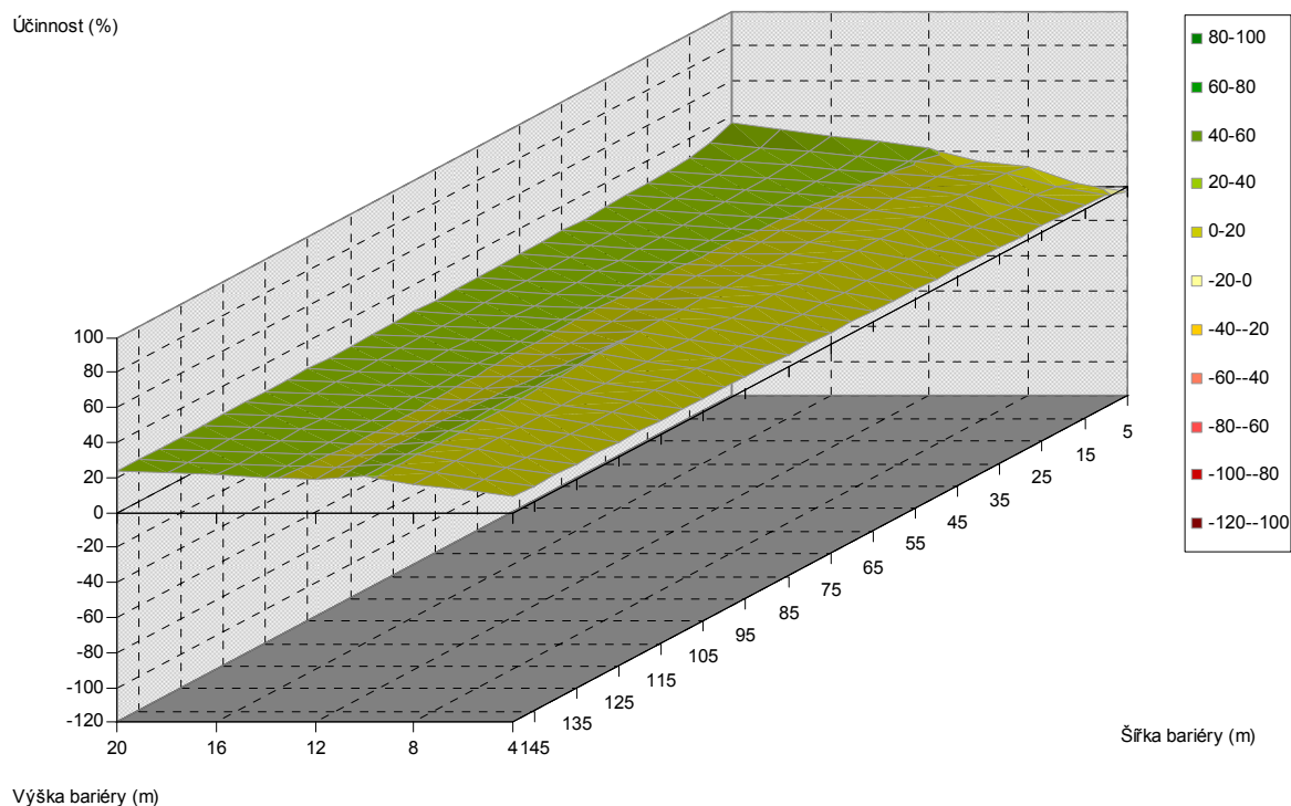
Obr. 5.318. Závislost účinnosti vegetační bariéry na výšce a šířce bariéry, pro vzdálenost od komunikace 20 m, jehličnaté dřeviny, PM10, 6 m nad povrchem
