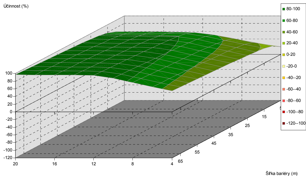
Obr. 5.387. Závislost účinnosti vegetační bariéry na výšce a šířce bariéry, pro vzdálenost od komunikace 80 m, listnaté dřeviny, PM75, 6 m nad povrchem
