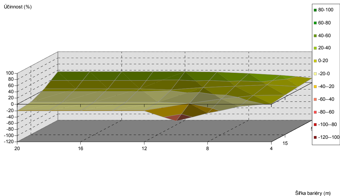
Obr. 5.293. Závislost účinnosti vegetační bariéry na výšce a šířce bariéry, pro vzdálenost od komunikace 30 m, jehličnaté dřeviny, PM10, 3 m nad povrchem
