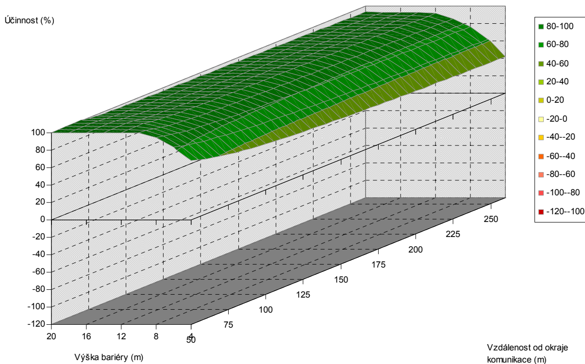
Obr. 5.84. Závislost účinnosti vegetační bariéry na výšce bariéry a vzdálenosti od komunikace, pro šířku bariéry 40 m, jehličnaté dřeviny, PM75, 1,5 m nad povrchem
