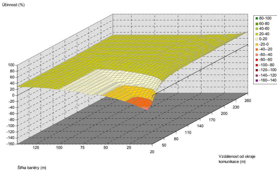
Obr. 5.142. Závislost účinnosti vegetační bariéry na šířce bariéry a vzdálenosti od komunikace, pro výšku bariéry 20 m, listnaté dřeviny, PM10, 1,5 m nad povrchem
