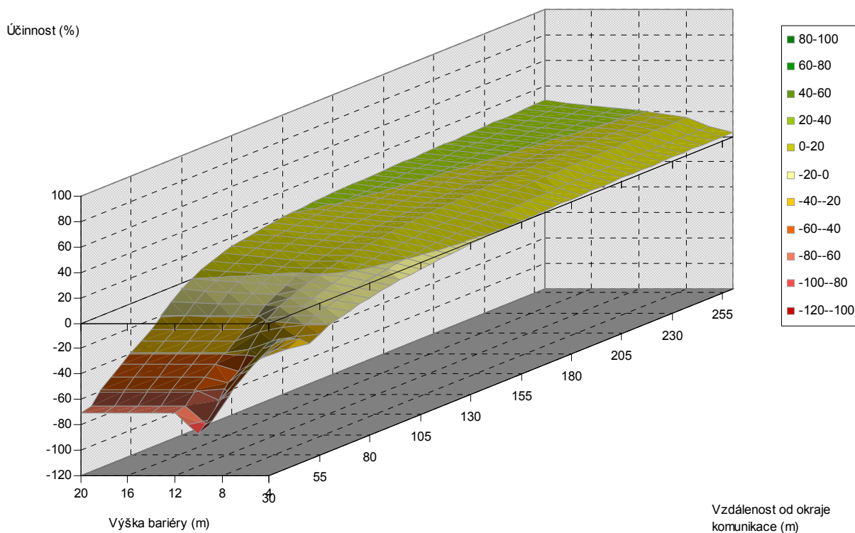
Obr. 5.50. Závislost účinnosti vegetační bariéry na výšce bariéry a vzdálenosti od komunikace, pro šířku bariéry 30 m, listnaté dřeviny, PM10, 6 m nad povrchem
