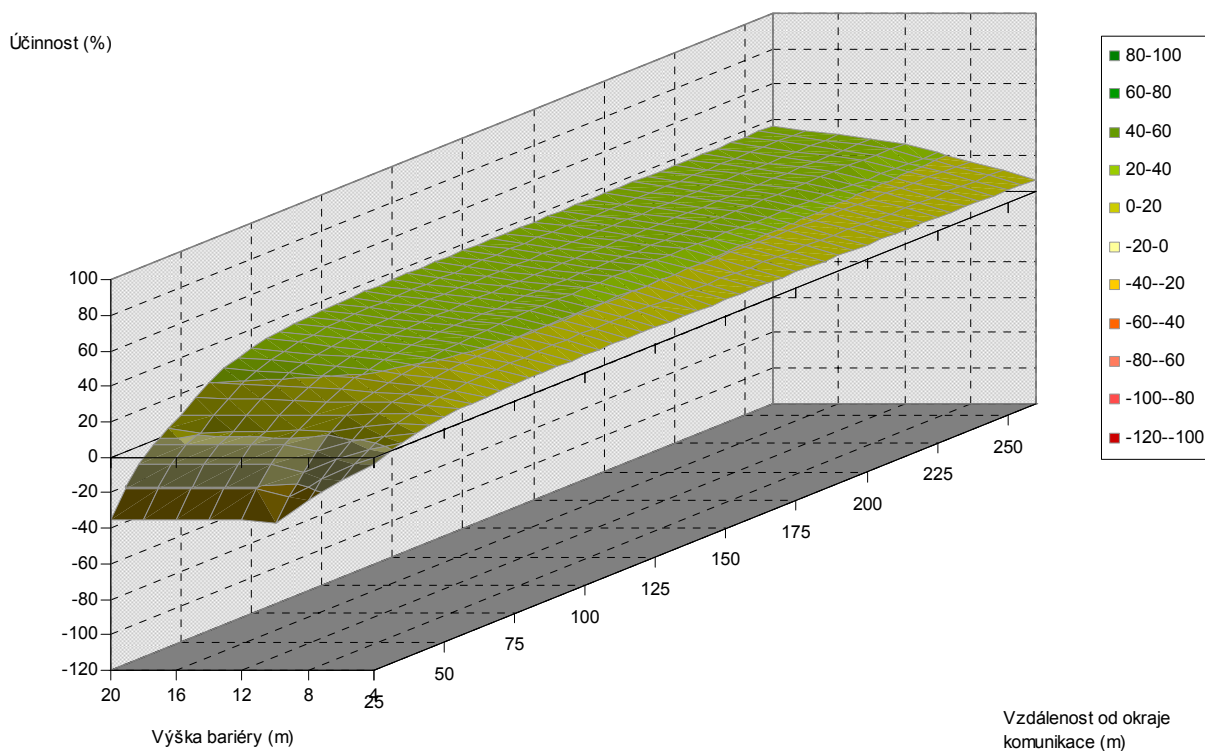
Obr. 5.4. Závislost účinnosti vegetační bariéry na výšce bariéry a vzdálenosti od komunikace, pro šířku bariéry 18 m, listnaté dřeviny, PM10, 1,5 m nad povrchem
