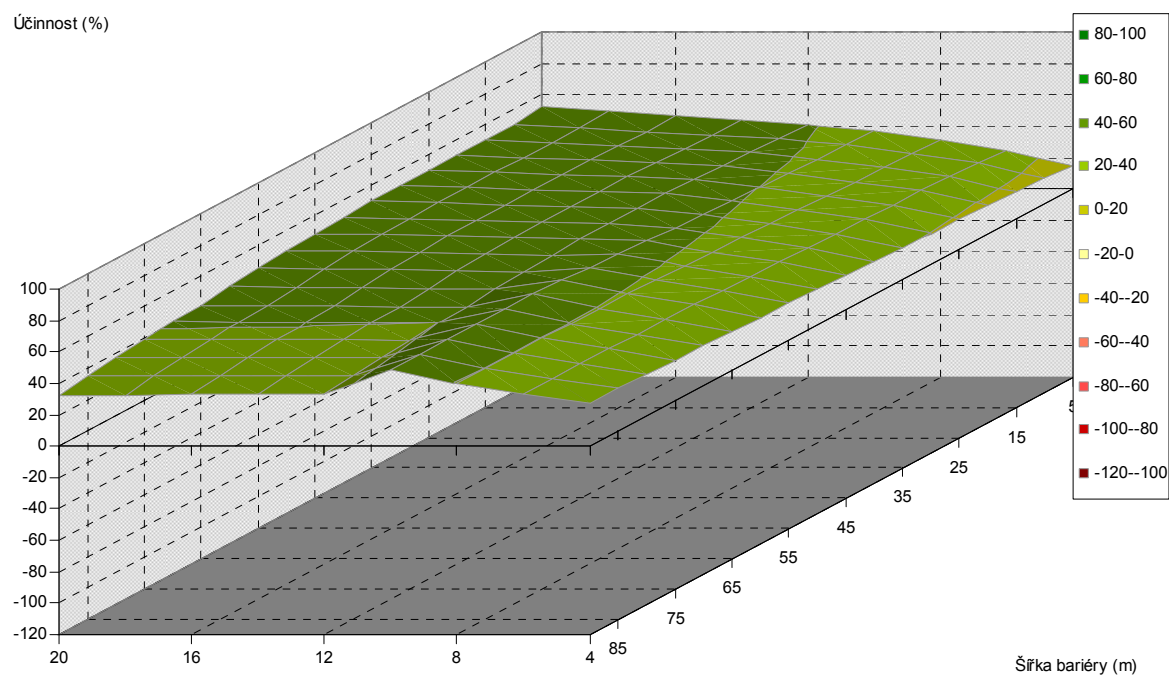
Obr. 5.297. Závislost účinnosti vegetační bariéry na výšce a šířce bariéry, pro vzdálenost od komunikace 100 m, jehličnaté dřeviny, PM10, 3 m nad povrchem
