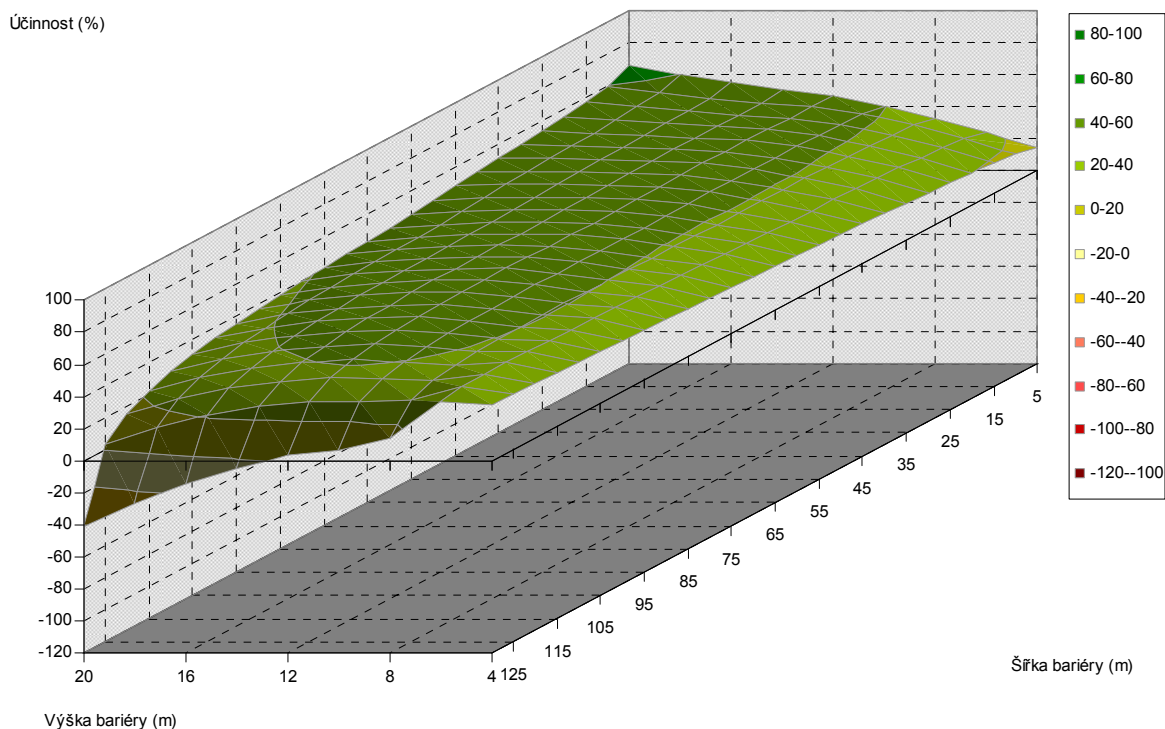
Obr. 5.274. Závislost účinnosti vegetační bariéry na výšce a šířce bariéry, pro vzdálenost od komunikace 160 m, jehličnaté dřeviny, PM10, 1,5 m nad povrchem
