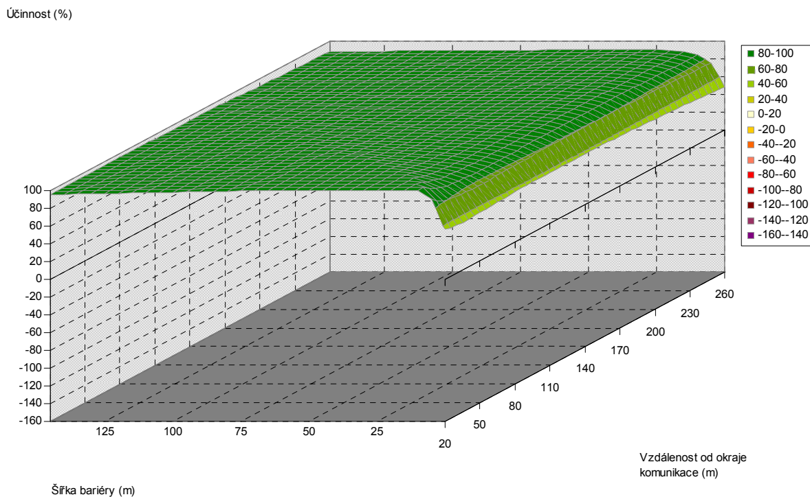
Obr. 5.250. Závislost účinnosti vegetační bariéry na šířce bariéry a vzdálenosti od komunikace, pro výšku bariéry 15 m, jehličnaté dřeviny, PM75, 6 m nad povrchem
