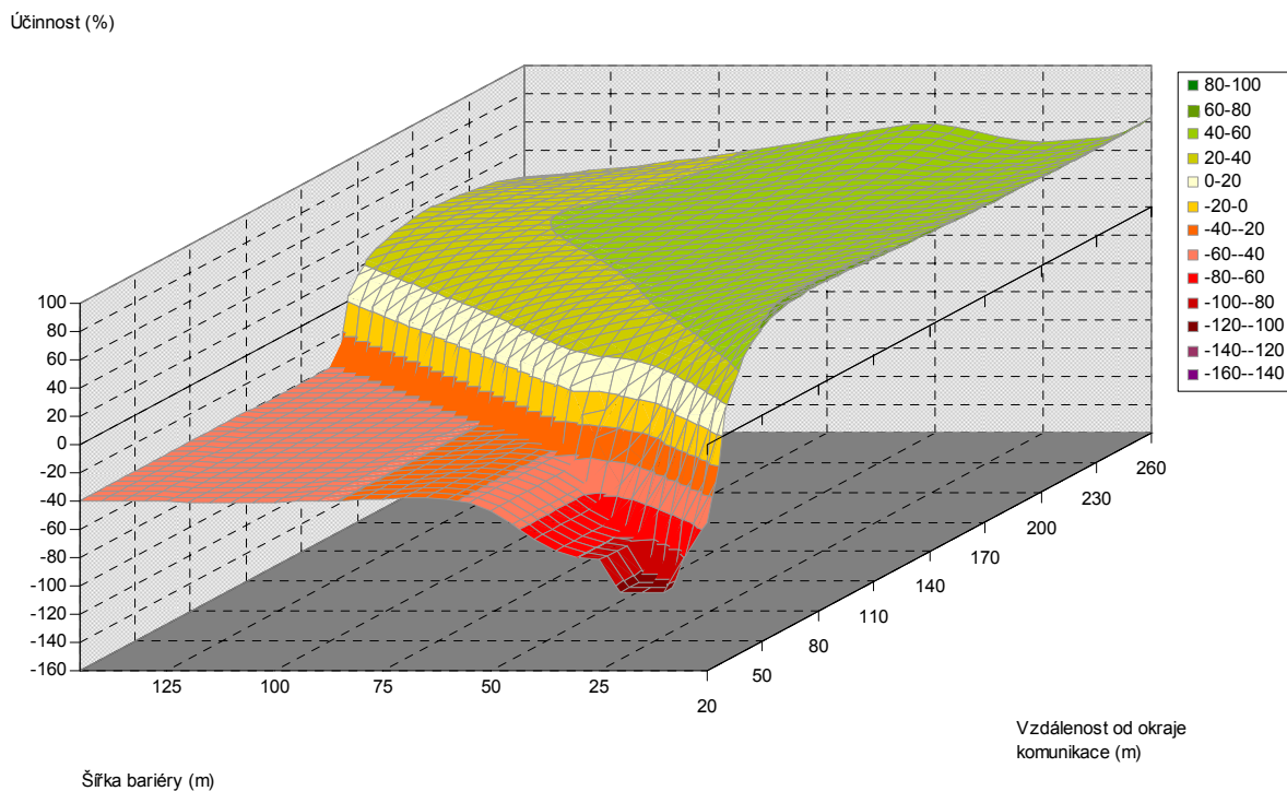
Obr. 5.152. Závislost účinnosti vegetační bariéry na šířce bariéry a vzdálenosti od komunikace, pro výšku bariéry 20 m, jehličnaté dřeviny, PM10, 1,5 m nad povrchem
