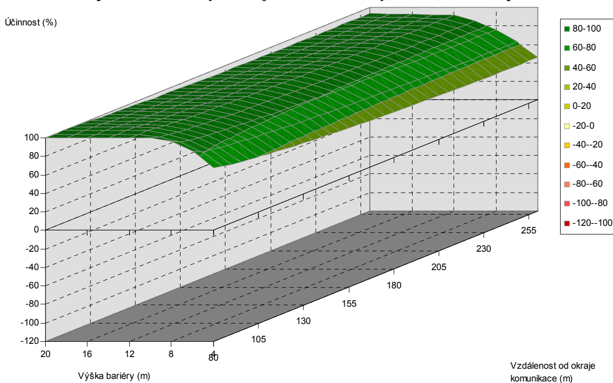
Obr. 5.108. Závislost účinnosti vegetační bariéry na výšce bariéry a vzdálenosti od komunikace, pro šířku bariéry 70 m, jehličnaté dřeviny, PM75, 3 m nad povrchem
