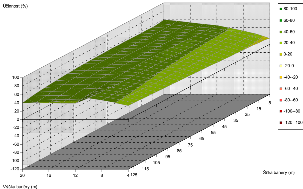
Obr. 5.300. Závislost účinnosti vegetační bariéry na výšce a šířce bariéry, pro vzdálenost od komunikace 160 m, jehličnaté dřeviny, PM10, 3 m nad povrchem
