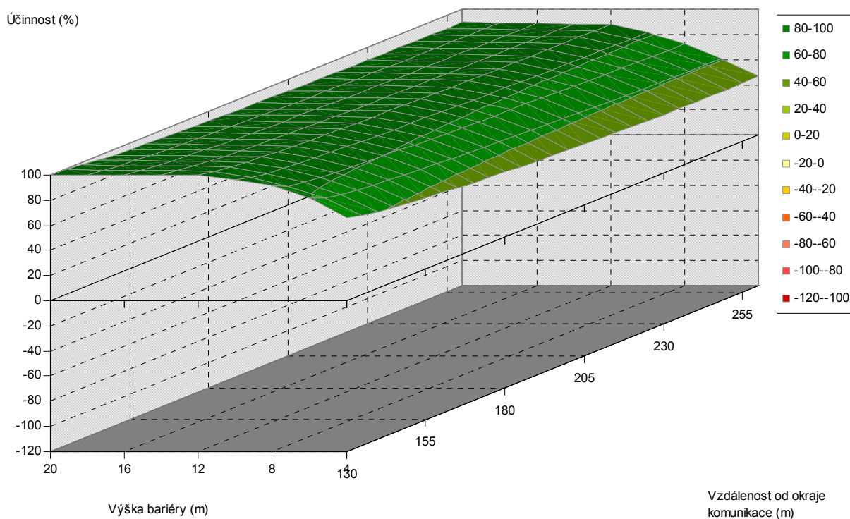
Obr. 5.100. Závislost účinnosti vegetační bariéry na výšce bariéry a vzdálenosti od komunikace, pro šířku bariéry 4 m, jehličnaté dřeviny, PM75, 3 m nad povrchem
