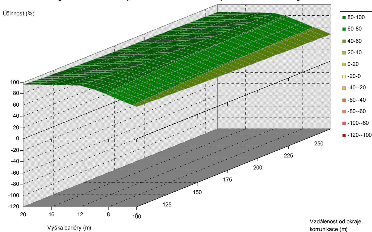
Obr. 5.120. Závislost účinnosti vegetační bariéry na výšce bariéry a vzdálenosti od komunikace, pro šířku bariéry 90 m, listnaté dřeviny, PM75, 6 m nad povrchem
