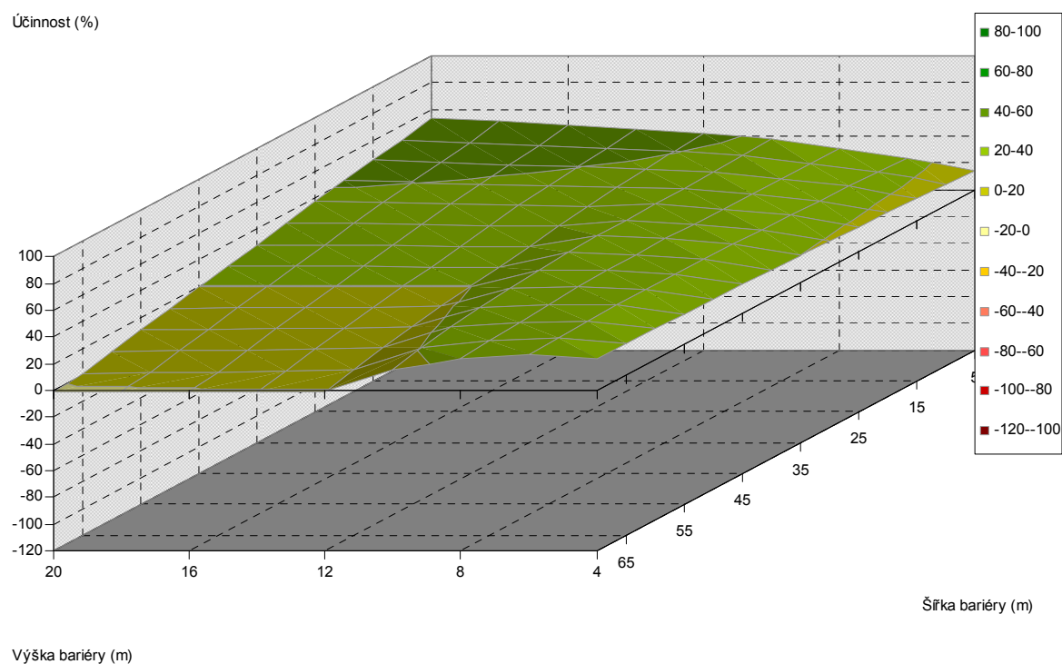
Obr. 5.296. Závislost účinnosti vegetační bariéry na výšce a šířce bariéry, pro vzdálenost od komunikace 80 m, jehličnaté dřeviny, PM10, 3 m nad povrchem
