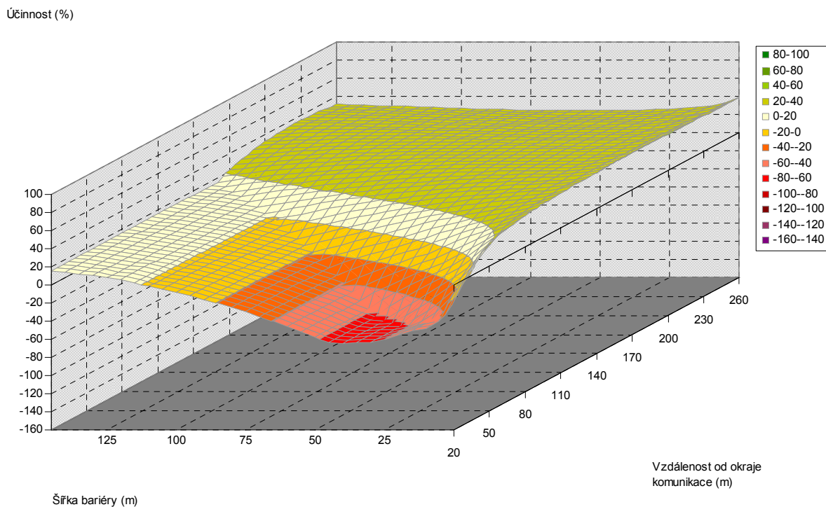
Obr. 5.162. Závislost účinnosti vegetační bariéry na šířce bariéry a vzdálenosti od komunikace, pro výšku bariéry 20 m, listnaté dřeviny, PM10, 3 m nad povrchem
