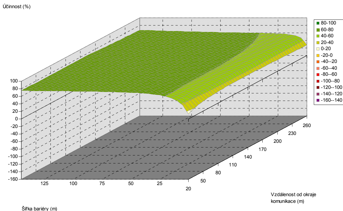
Obr. 5.238. Závislost účinnosti vegetační bariéry na šířce bariéry a vzdálenosti od komunikace, pro výšku bariéry 11 m, listnaté dřeviny, PM75, 6 m nad povrchem
