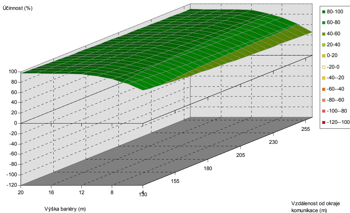
Obr. 5.78. Závislost účinnosti vegetační bariéry na výšce bariéry a vzdálenosti od komunikace, pro šířku bariéry 4 m, jehličnaté dřeviny, PM75, 1,5 m nad povrchem
