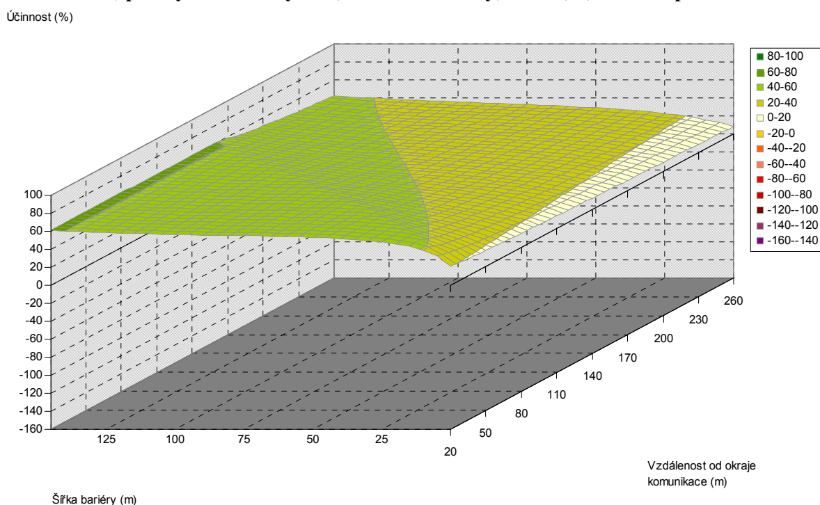
Obr. 5.194. Závislost účinnosti vegetační bariéry na šířce bariéry a vzdálenosti od komunikace, pro výšku bariéry 4 m, listnaté dřeviny, PM75, 1,5 m nad povrchem
