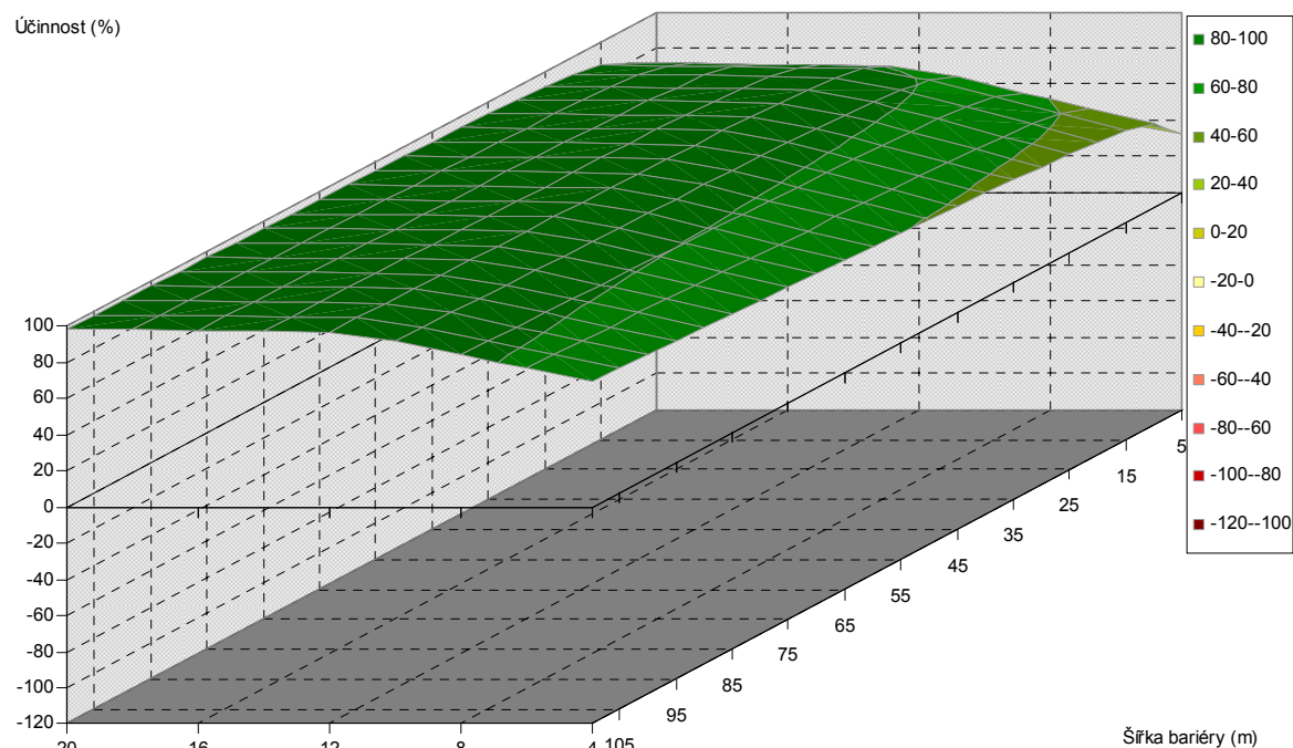
Obr. 5.402. Závislost účinnosti vegetační bariéry na výšce a šířce bariéry, pro vzdálenost od komunikace 120 m, jehličnaté dřeviny, PM75, 6 m nad povrchem
