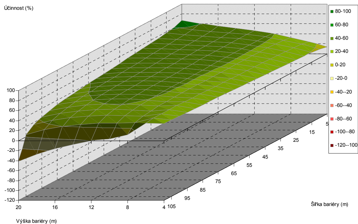
Obr. 5.272. Závislost účinnosti vegetační bariéry na výšce a šířce bariéry, pro vzdálenost od komunikace 120 m, jehličnaté dřeviny, PM10, 1,5 m nad povrchem
