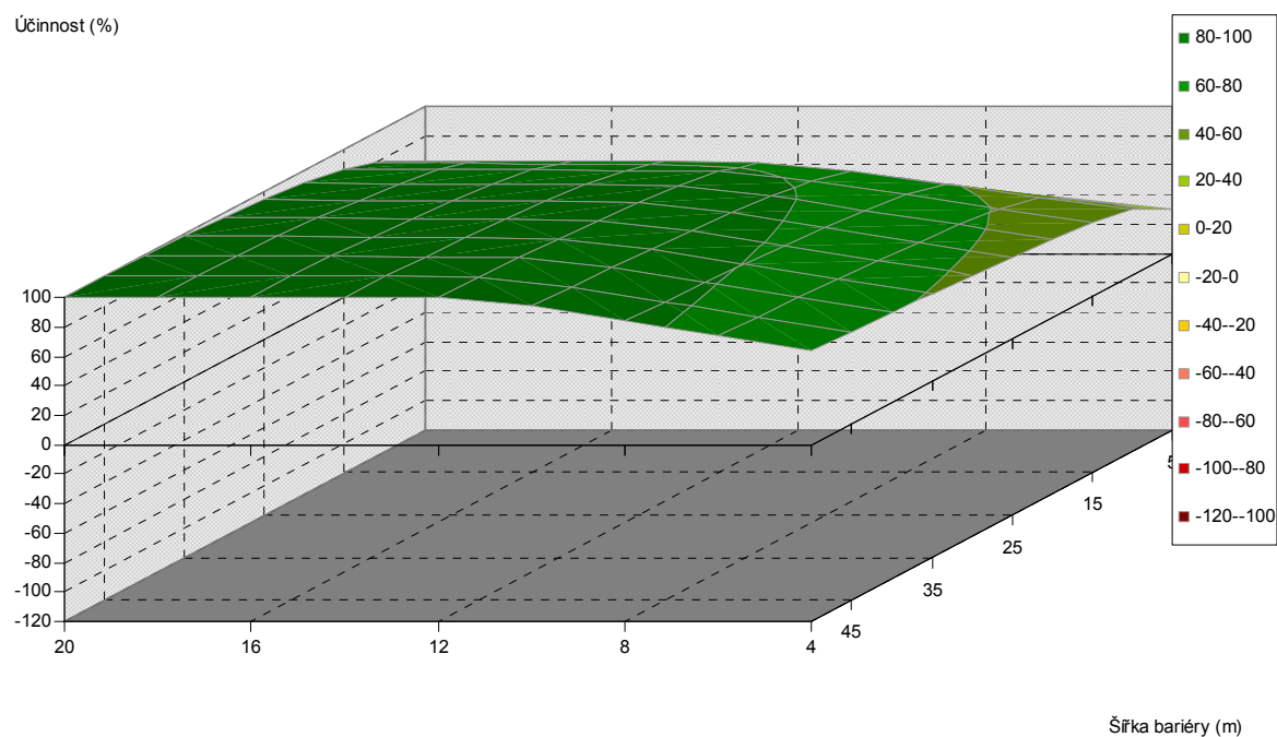
Obr. 5.399. Závislost účinnosti vegetační bariéry na výšce a šířce bariéry, pro vzdálenost od komunikace 60 m, jehličnaté dřeviny, PM75, 6 m nad povrchem
