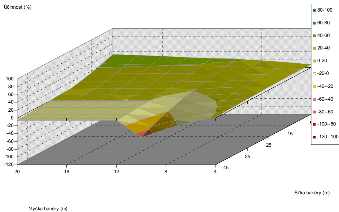
Obr. 5.256. Závislost účinnosti vegetační bariéry na výšce a šířce bariéry, pro vzdálenost od komunikace 60 m, listnaté dřeviny, PM10, 1,5 m nad povrchem
