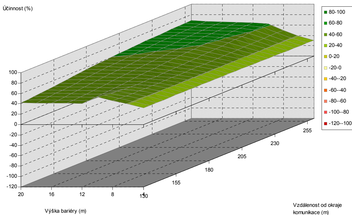
Obr. 5.44. Závislost účinnosti vegetační bariéry na výšce bariéry a vzdálenosti od komunikace, pro šířku bariéry 120 m, jehličnaté dřeviny, PM10, 3 m nad povrchem
