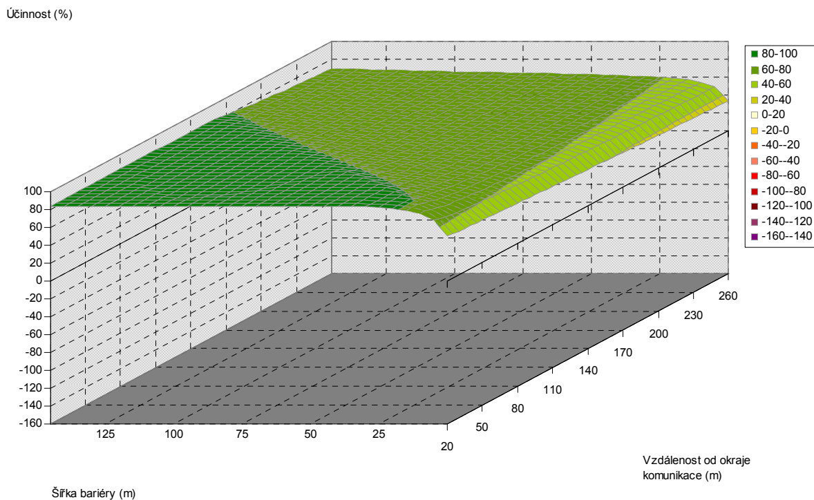
Obr. 5.206. Závislost účinnosti vegetační bariéry na šířce bariéry a vzdálenosti od komunikace, pro výšku bariéry 6 m, jehličnaté dřeviny, PM75, 1,5 m nad povrchem
