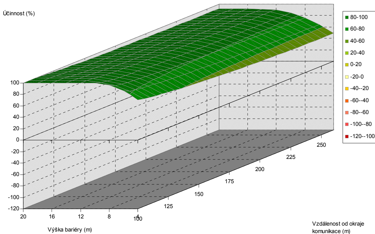
Obr. 5.110. Závislost účinnosti vegetační bariéry na výšce bariéry a vzdálenosti od komunikace, pro šířku bariéry 120 m, jehličnaté dřeviny, PM75, 3 m nad povrchem
