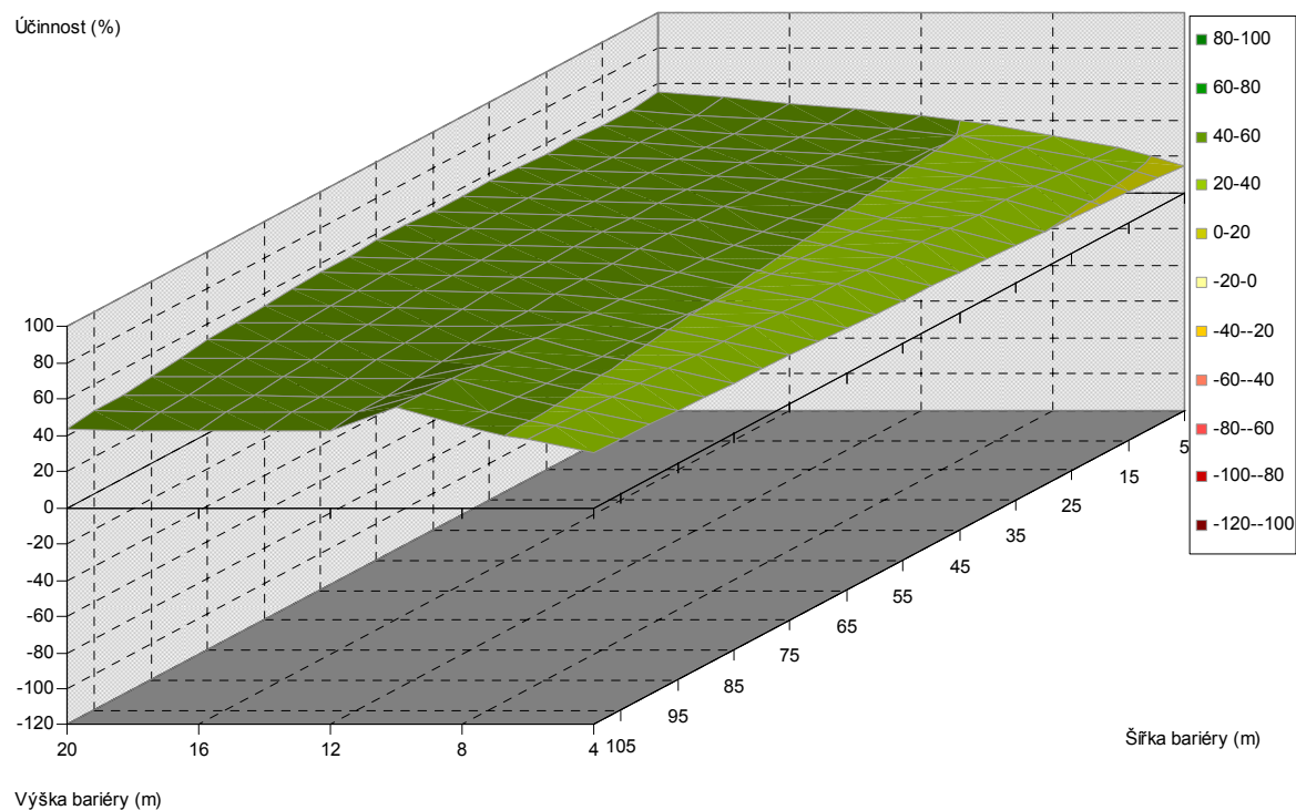
Obr. 5.298. Závislost účinnosti vegetační bariéry na výšce a šířce bariéry, pro vzdálenost od komunikace 120 m, jehličnaté dřeviny, PM10, 3 m nad povrchem
