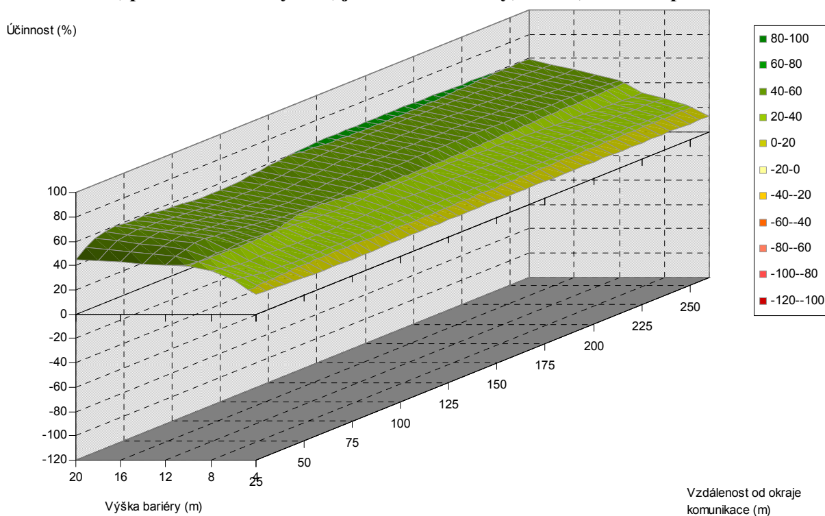
Obr. 5.34. Závislost účinnosti vegetační bariéry na výšce bariéry a vzdálenosti od komunikace, pro šířku bariéry 4 m, jehličnaté dřeviny, PM10, 3 m nad povrchem
