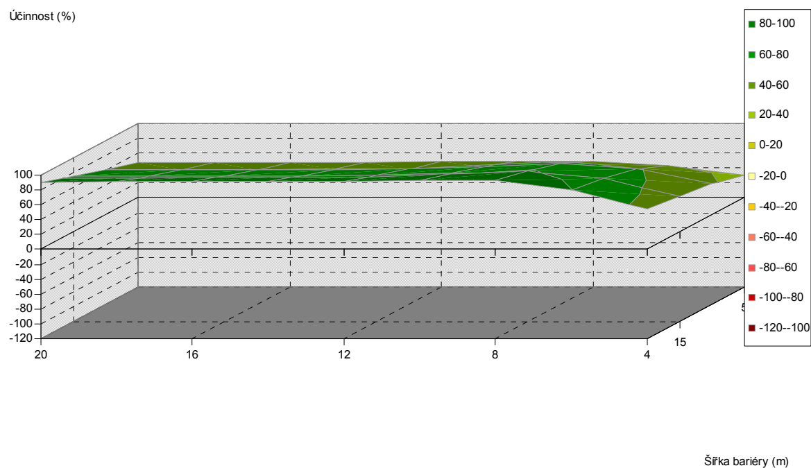
Obr. 5.371. Závislost účinnosti vegetační bariéry na výšce a šířce bariéry, pro vzdálenost od komunikace 30 m, jehličnaté dřeviny, PM75, 3 m nad povrchem
