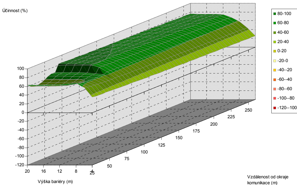
Obr. 5.92. Závislost účinnosti vegetační bariéry na výšce bariéry a vzdálenosti od komunikace, pro šířku bariéry 18 m, listnaté dřeviny, PM75, 3 m nad povrchem
