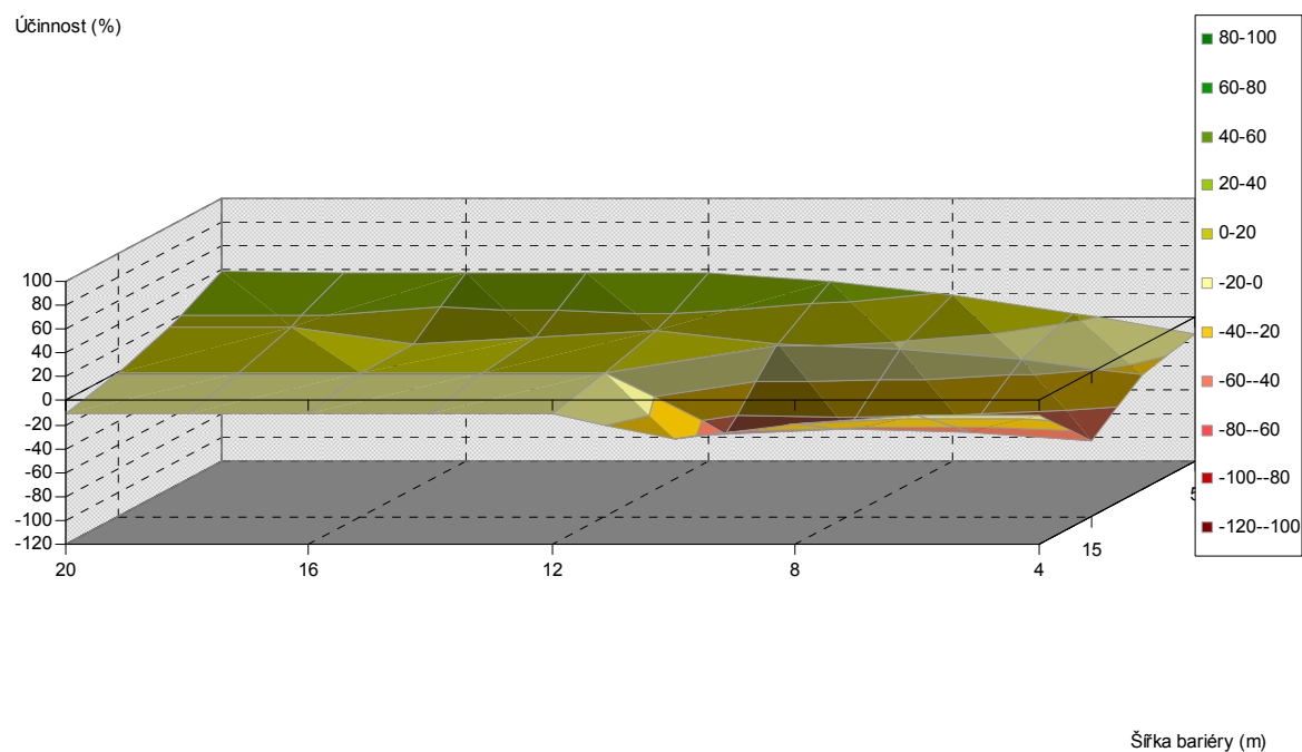
Obr. 5.319. Závislost účinnosti vegetační bariéry na výšce a šířce bariéry, pro vzdálenost od komunikace 30 m, jehličnaté dřeviny, PM10, 6 m nad povrchem
