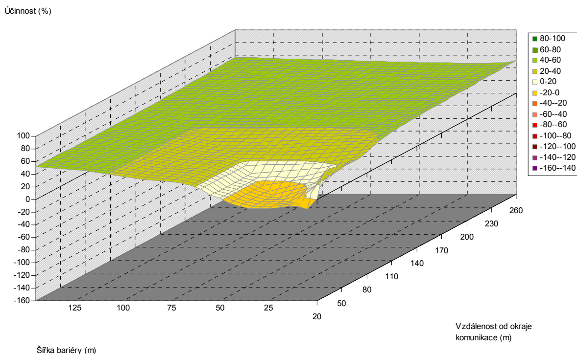
Obr. 5.192. Závislost účinnosti vegetační bariéry na šířce bariéry a vzdálenosti od komunikace, pro výšku bariéry 20 m, jehličnaté dřeviny, PM10, 6 m nad povrchem
