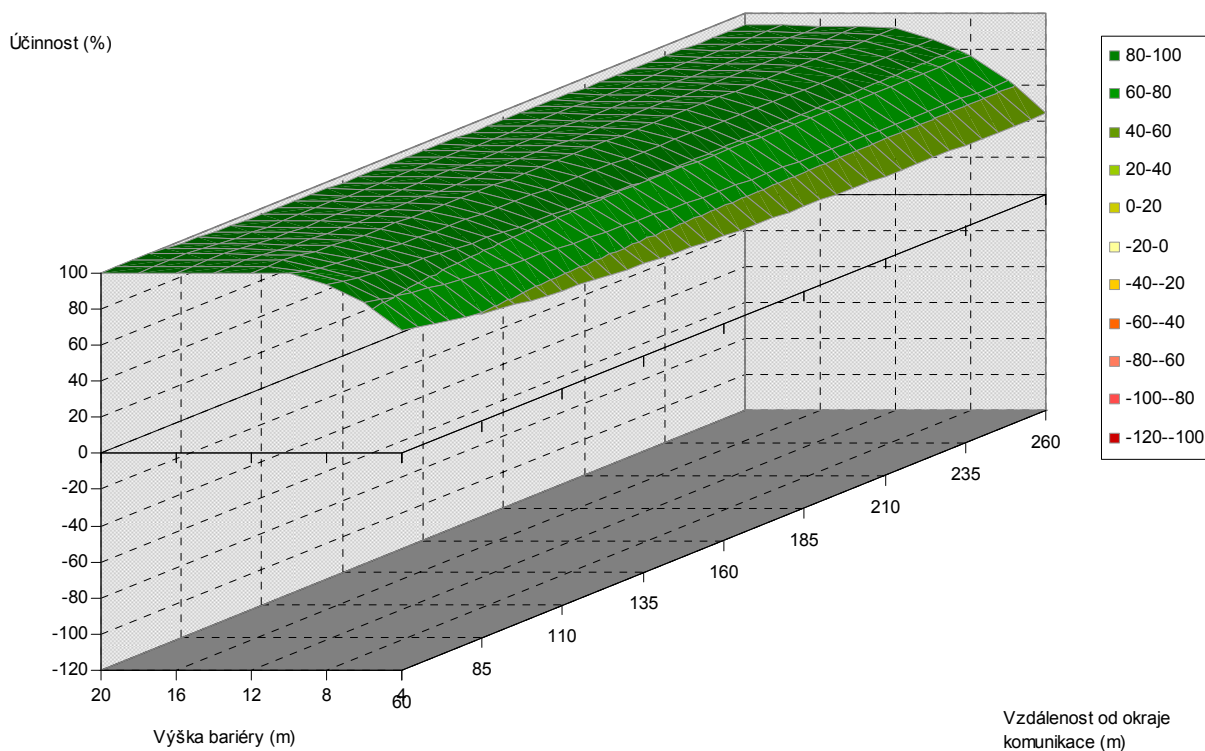
Obr. 5.86. Závislost účinnosti vegetační bariéry na výšce bariéry a vzdálenosti od komunikace, pro šířku bariéry 70 m, jehličnaté dřeviny, PM75, 1,5 m nad povrchem
