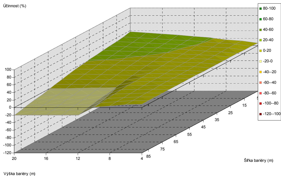
Obr. 5.284. Závislost účinnosti vegetační bariéry na výšce a šířce bariéry, pro vzdálenost od komunikace 100 m, listnaté dřeviny, PM10, 3 m nad povrchem
