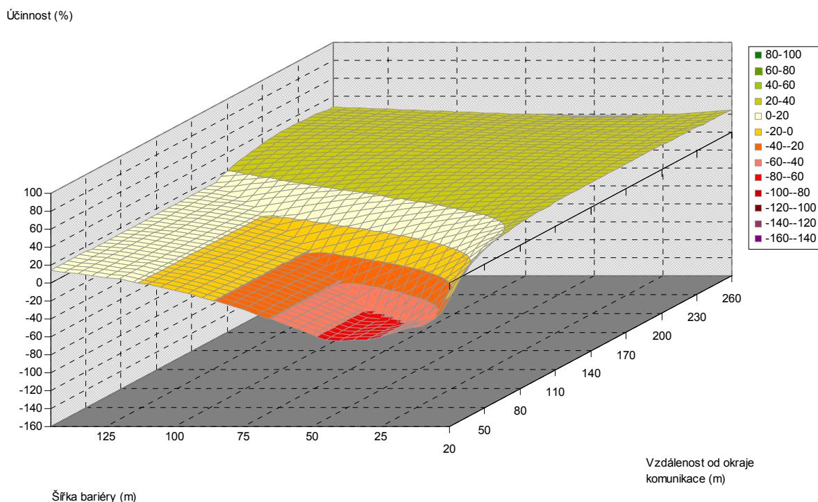
Obr. 5.160. Závislost účinnosti vegetační bariéry na šířce bariéry a vzdálenosti od komunikace, pro výšku bariéry 15 m, listnaté dřeviny, PM10, 3 m nad povrchem
