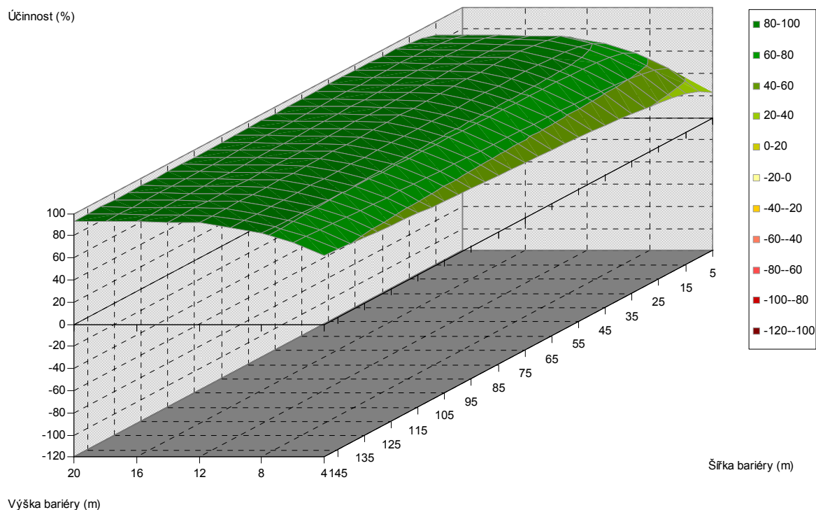
Obr. 5.356. Závislost účinnosti vegetační bariéry na výšce a šířce bariéry, pro vzdálenost od komunikace 240 m, jehličnaté dřeviny, PM75, 1,5 m nad povrchem
