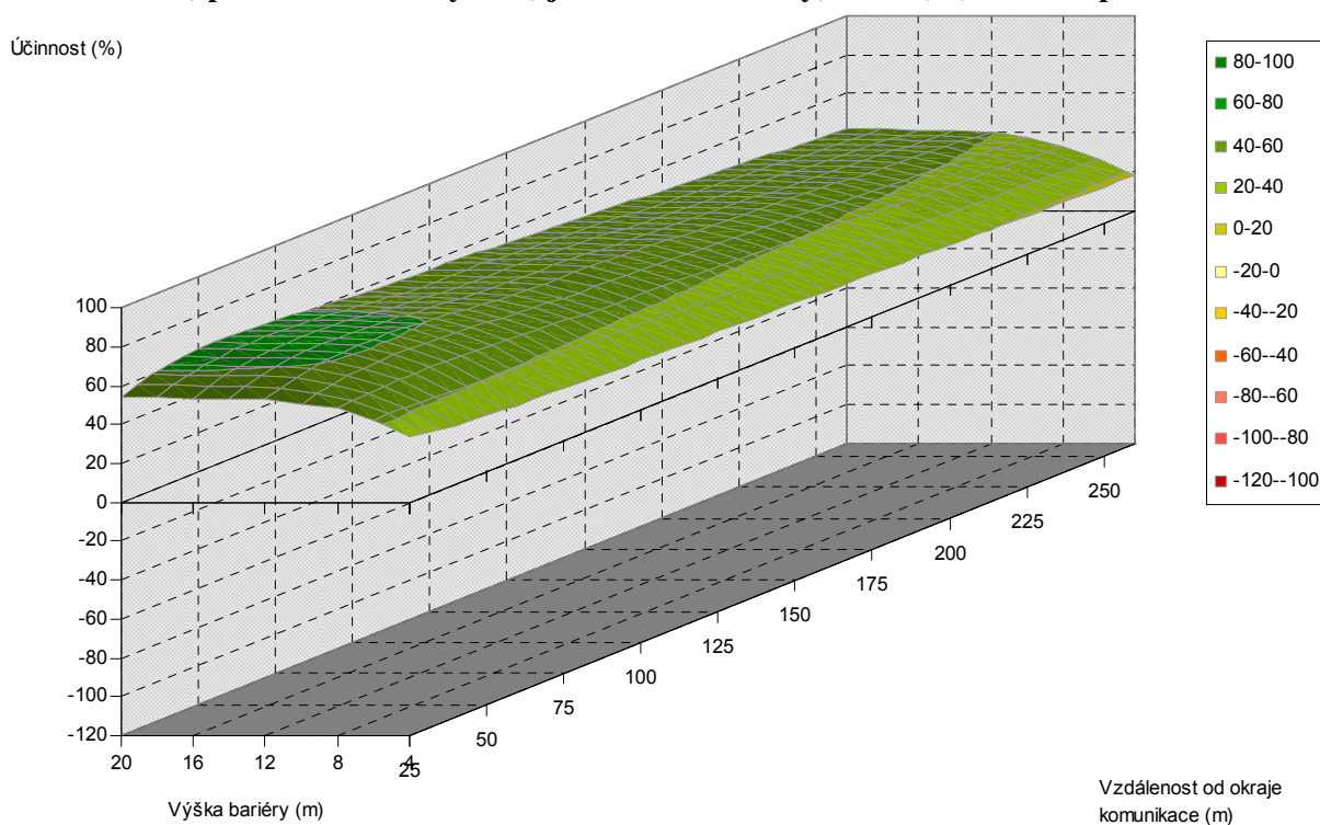
Obr. 5.78. Závislost účinnosti vegetační bariéry na výšce bariéry a vzdálenosti od komunikace, pro šířku bariéry 4 m, jehličnaté dřeviny, PM75, 1,5 m nad povrchem
