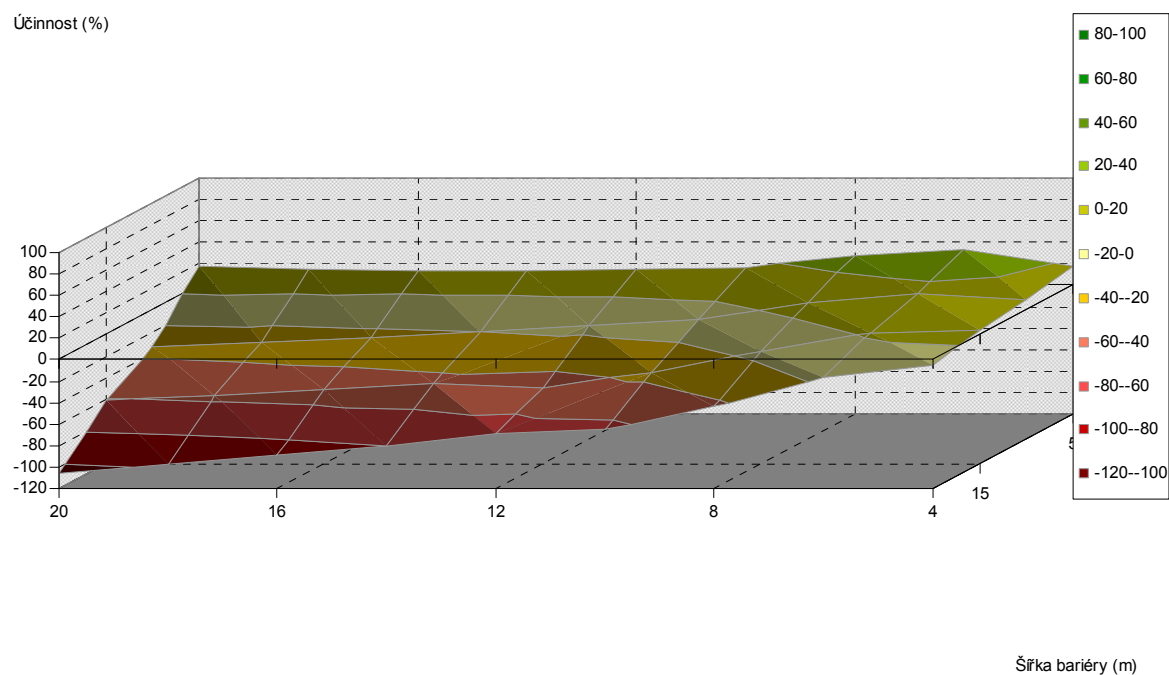
Obr. 5.267. Závislost účinnosti vegetační bariéry na výšce a šířce bariéry, pro vzdálenost od komunikace 30 m, jehličnaté dřeviny, PM10, 1,5 m nad povrchem
