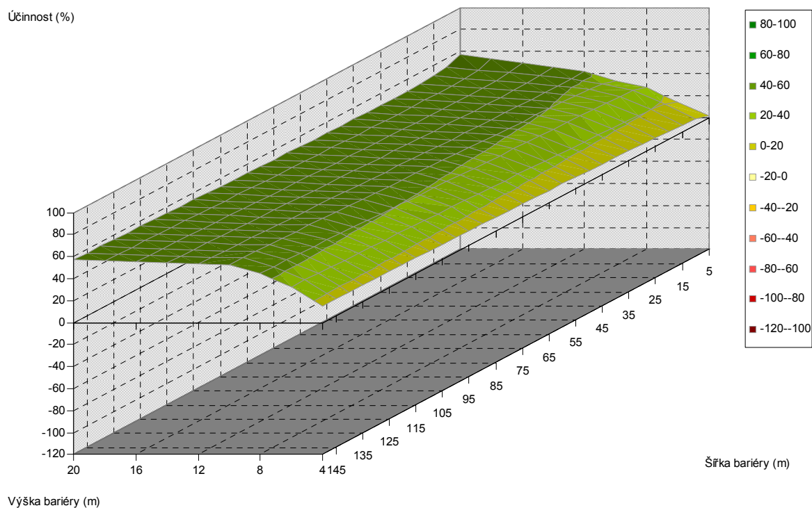
Obr. 5.330. Závislost účinnosti vegetační bariéry na výšce a šířce bariéry, pro vzdálenost od komunikace 240 m, jehličnaté dřeviny, PM10, 6 m nad povrchem
