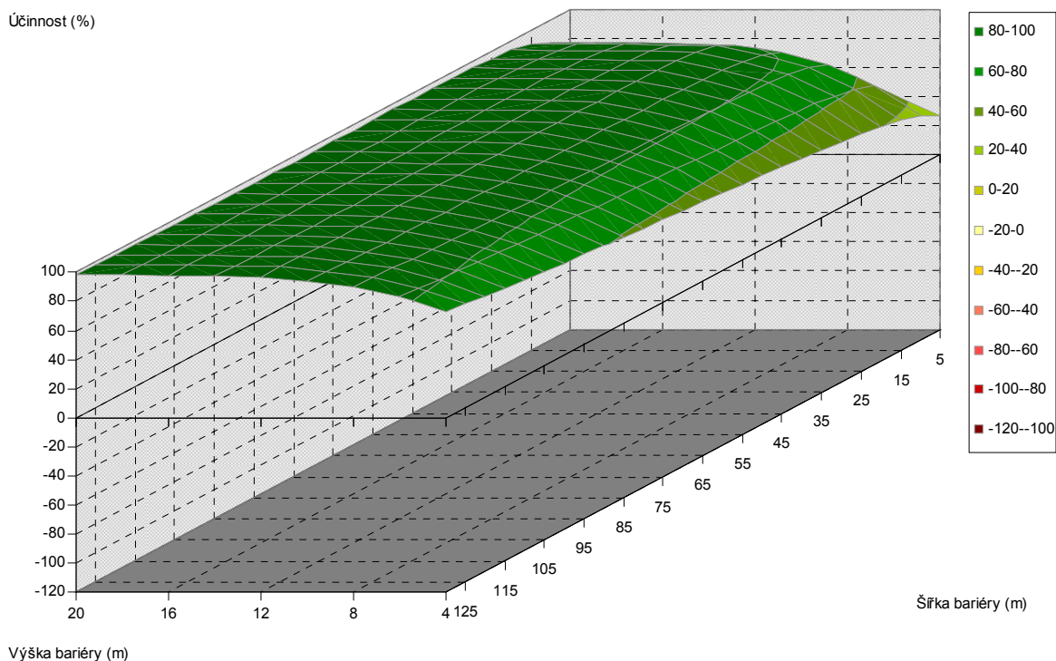
Obr. 5.352. Závislost účinnosti vegetační bariéry na výšce a šířce bariéry, pro vzdálenost od komunikace 160 m, jehličnaté dřeviny, PM75, 1,5 m nad povrchem
