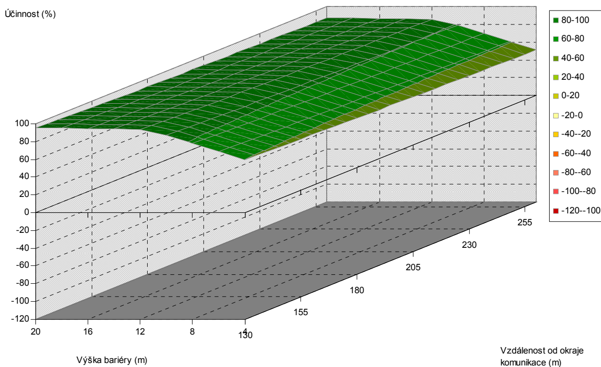
Obr. 5.122. Závislost účinnosti vegetační bariéry na výšce bariéry a vzdálenosti od komunikace, pro šířku bariéry 4 m, jehličnaté dřeviny, PM75, 6 m nad povrchem
