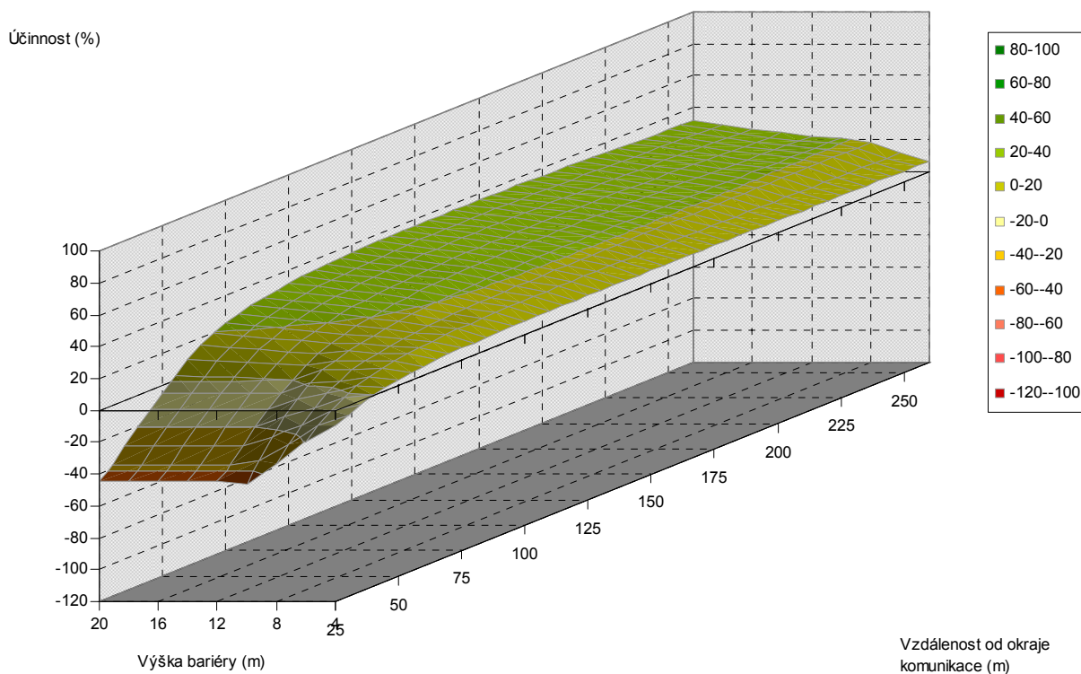
Obr. 5.26. Závislost účinnosti vegetační bariéry na výšce bariéry a vzdálenosti od komunikace, pro šířku bariéry 18 m, listnaté dřeviny, PM10, 3 m nad povrchem
