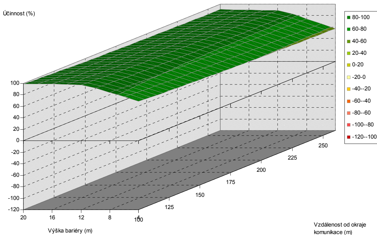
Obr. 5.132. Závislost účinnosti vegetační bariéry na výšce bariéry a vzdálenosti od komunikace, pro šířku bariéry 120 m, jehličnaté dřeviny, PM75, 6 m nad povrchem
