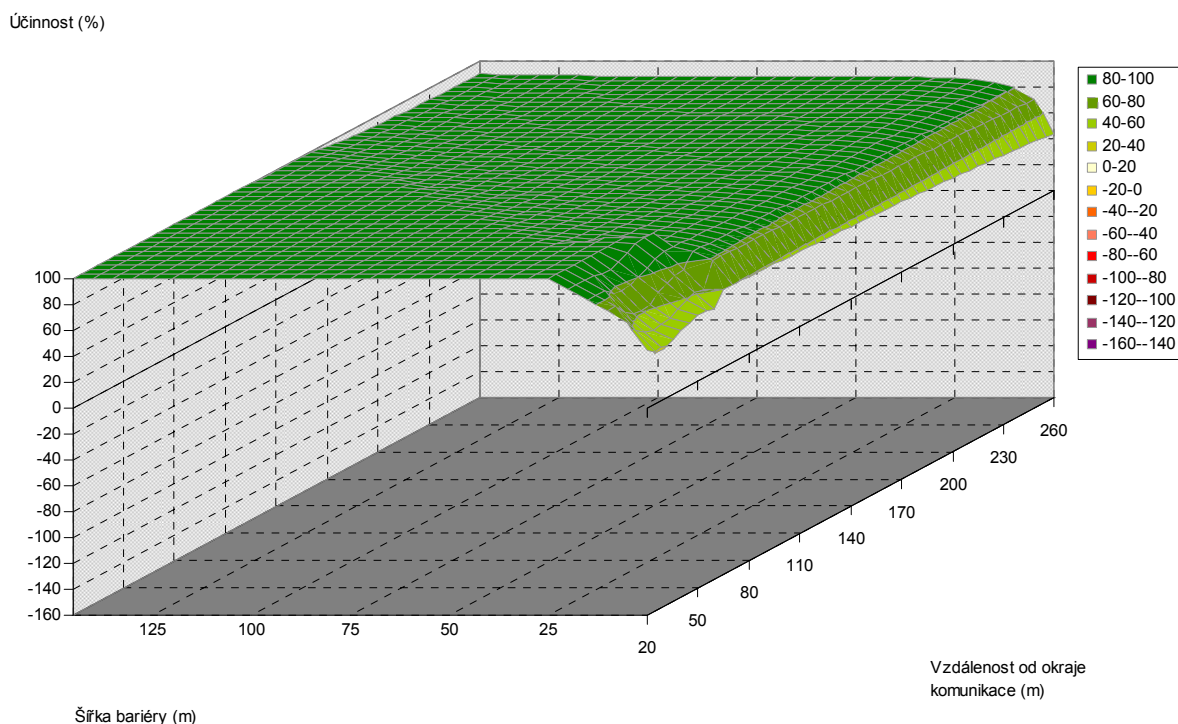
Obr. 5.222. Závislost účinnosti vegetační bariéry na šířce bariéry a vzdálenosti od komunikace, pro výšku bariéry 20 m, listnaté dřeviny, PM75, 3 m nad povrchem
