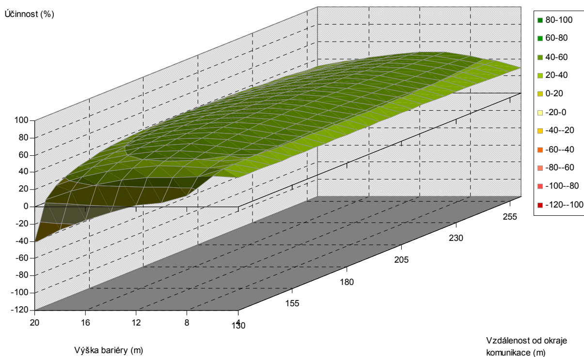
Obr. 5.22. Závislost účinnosti vegetační bariéry na výšce bariéry a vzdálenosti od komunikace, pro šířku bariéry 120 m, jehličnaté dřeviny, PM10, 1,5 m nad povrchem
