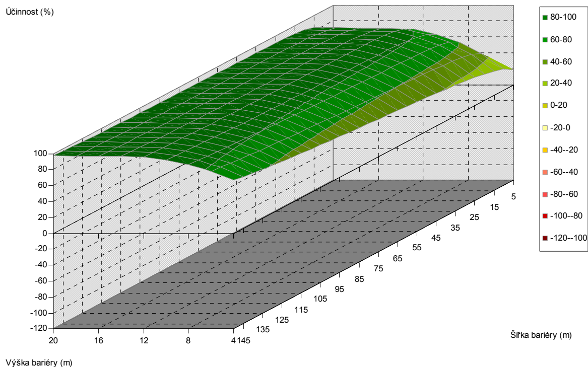
Obr. 5.340. Závislost účinnosti vegetační bariéry na výšce a šířce bariéry, pro vzdálenost od komunikace 180 m, listnaté dřeviny, PM75, 1,5 m nad povrchem
