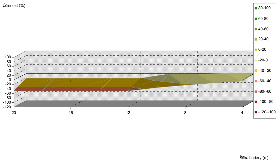
Obr. 5.253. Závislost účinnosti vegetační bariéry na výšce a šířce bariéry, pro vzdálenost od komunikace 20 m, listnaté dřeviny, PM10, 1,5 m nad povrchem
