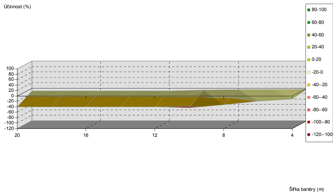
Obr. 5.279. Závislost účinnosti vegetační bariéry na výšce a šířce bariéry, pro vzdálenost od komunikace 20 m, listnaté dřeviny, PM10, 3 m nad povrchem
