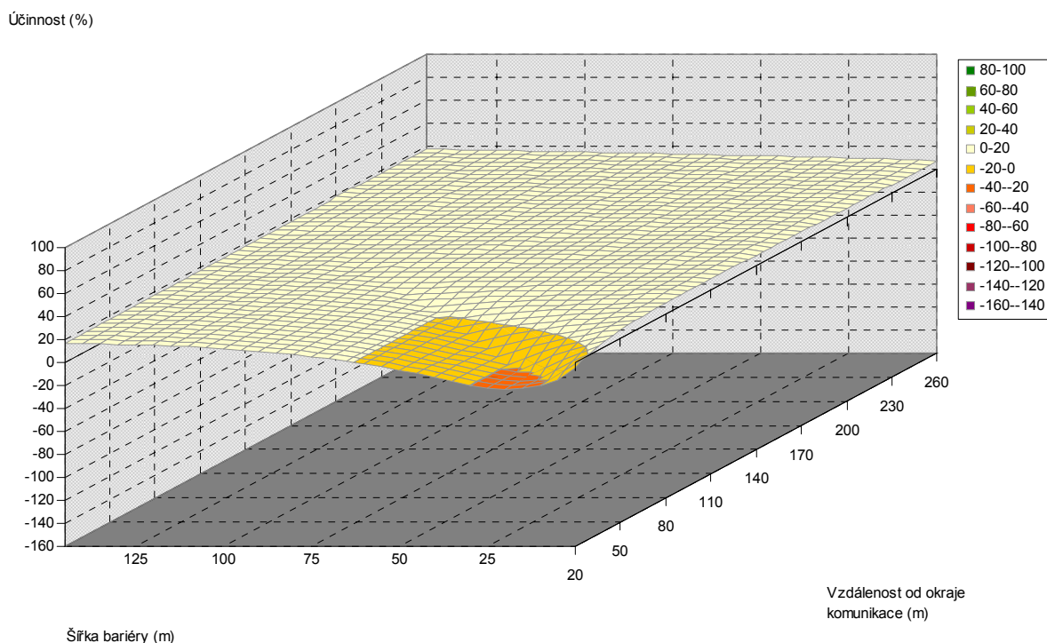
Obr. 5.156. Závislost účinnosti vegetační bariéry na šířce bariéry a vzdálenosti od komunikace, pro výšku bariéry 6 m, listnaté dřeviny, PM10, 3 m nad povrchem
