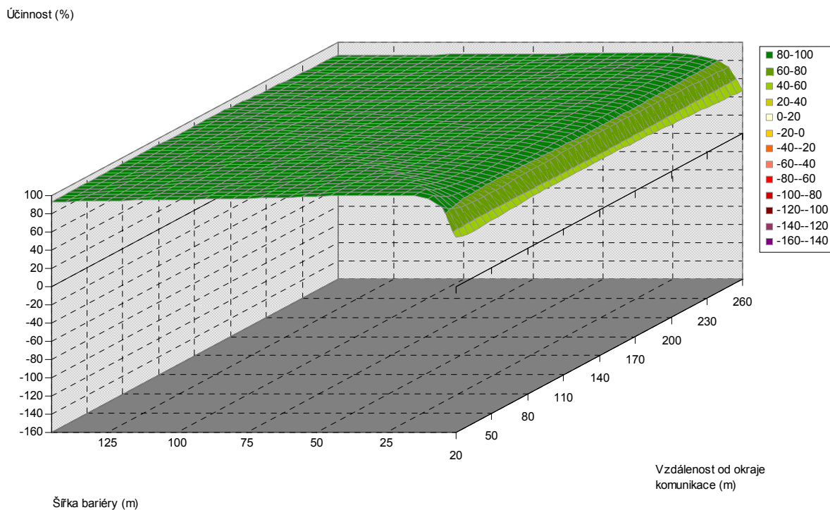
Obr. 5.248. Závislost účinnosti vegetační bariéry na šířce bariéry a vzdálenosti od komunikace, pro výšku bariéry 11 m, jehličnaté dřeviny, PM75, 6 m nad povrchem
