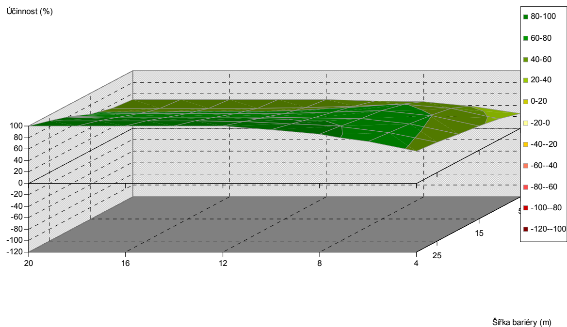
Obr. 5.333. Závislost účinnosti vegetační bariéry na výšce a šířce bariéry, pro vzdálenost od komunikace 40 m, listnaté dřeviny, PM75, 1,5 m nad povrchem
