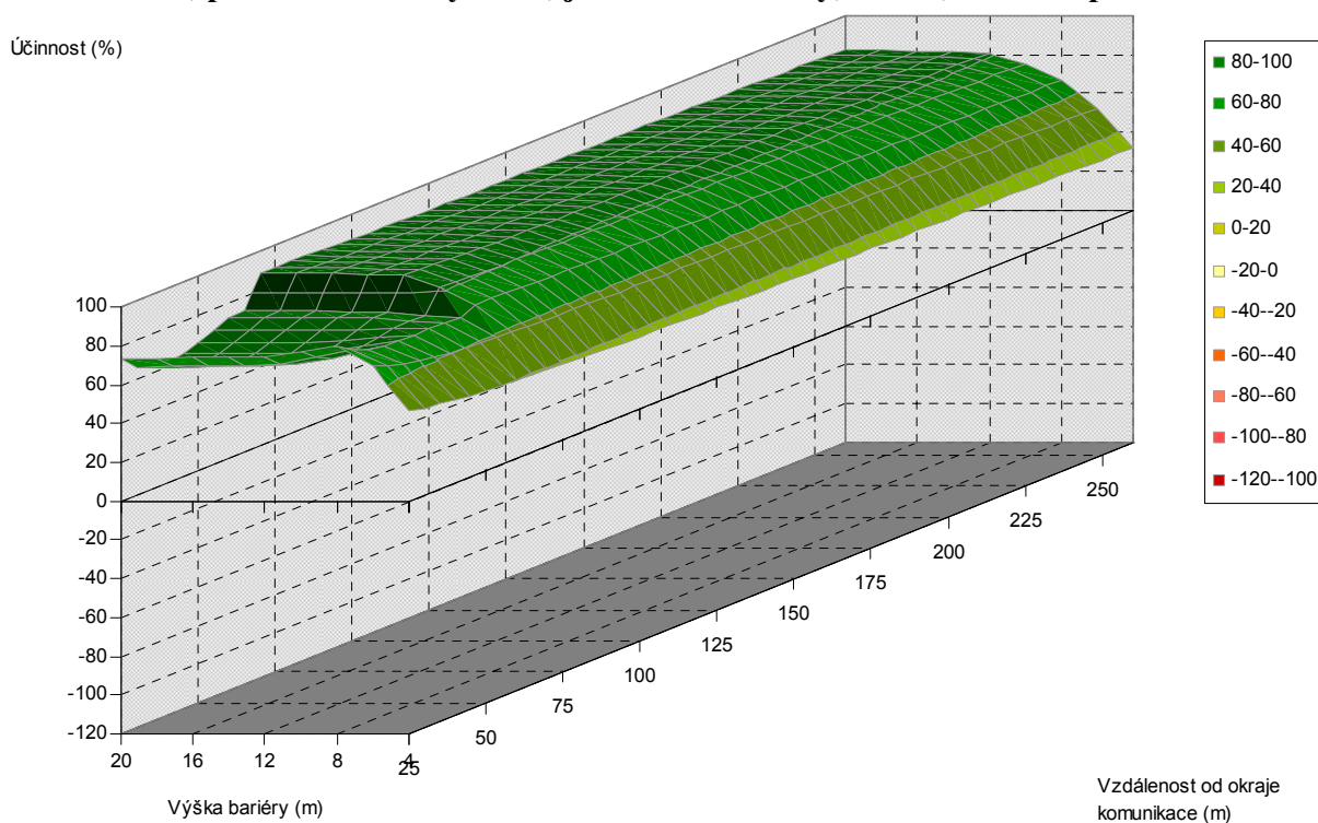
Obr. 5.102. Závislost účinnosti vegetační bariéry na výšce bariéry a vzdálenosti od komunikace, pro šířku bariéry 12 m, jehličnaté dřeviny, PM75, 3 m nad povrchem
