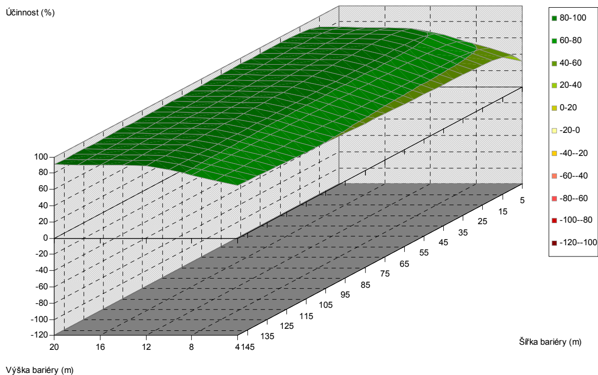
Obr. 5.408. Závislost účinnosti vegetační bariéry na výšce a šířce bariéry, pro vzdálenost od komunikace 240 m, jehličnaté dřeviny, PM75, 6 m nad povrchem
