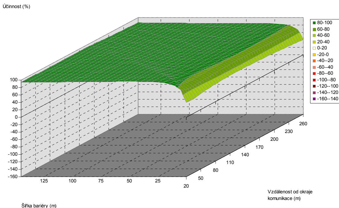
Obr. 5.240. Závislost účinnosti vegetační bariéry na šířce bariéry a vzdálenosti od komunikace, pro výšku bariéry 15 m, listnaté dřeviny, PM75, 6 m nad povrchem
