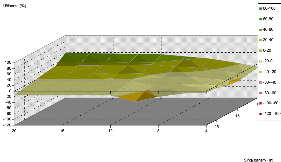
Obr. 5.320. Závislost účinnosti vegetační bariéry na výšce a šířce bariéry, pro vzdálenost od komunikace 40 m, jehličnaté dřeviny, PM10, 6 m nad povrchem
