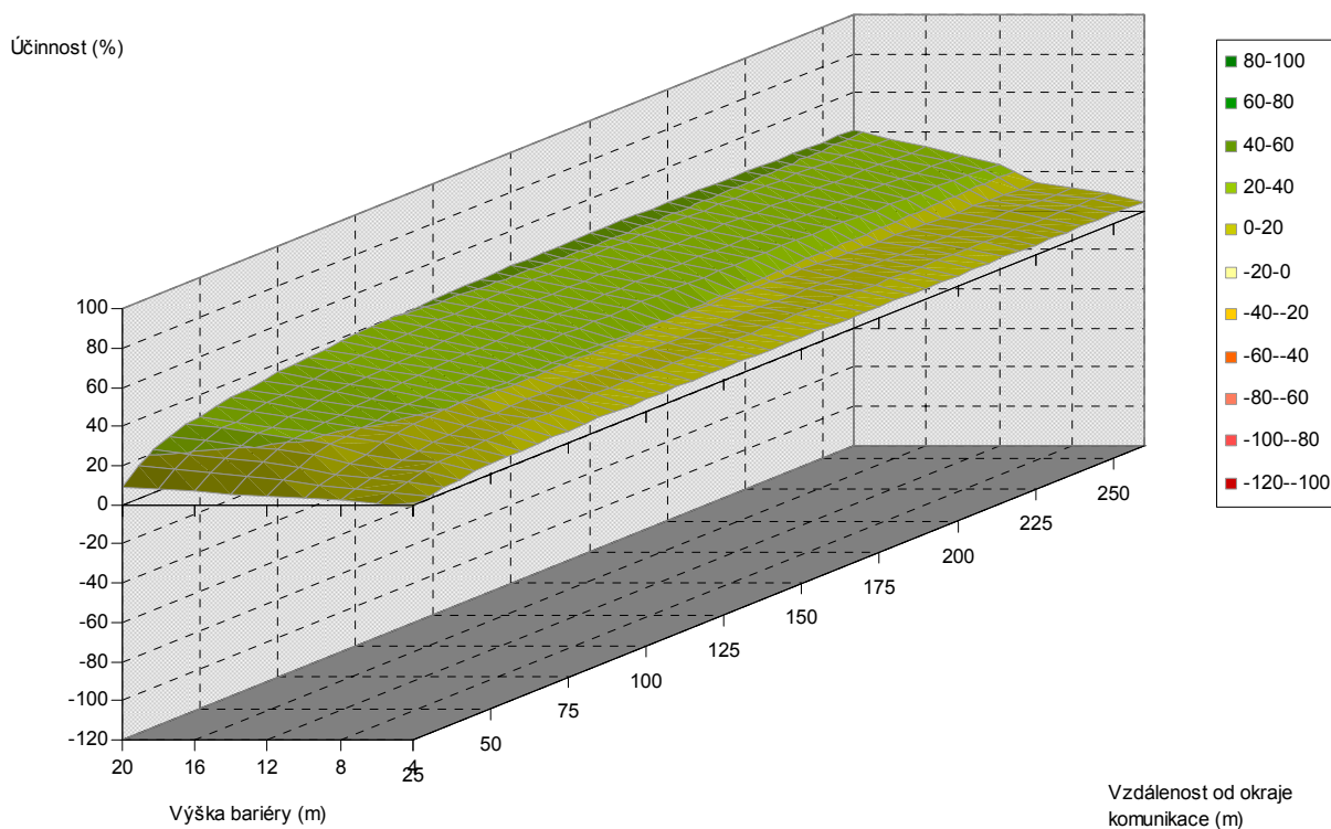
Obr. 5.24. Závislost účinnosti vegetační bariéry na výšce bariéry a vzdálenosti od komunikace, pro šířku bariéry 8 m, listnaté dřeviny, PM10, 3 m nad povrchem
