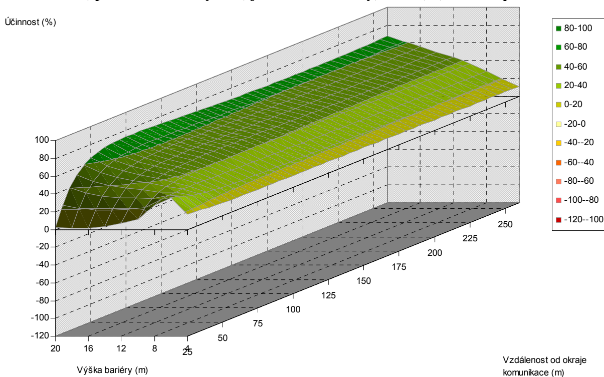
Obr. 5.12. Závislost účinnosti vegetační bariéry na výšce bariéry a vzdálenosti od komunikace, pro šířku bariéry 4 m, jehličnaté dřeviny, PM10, 1,5 m nad povrchem
