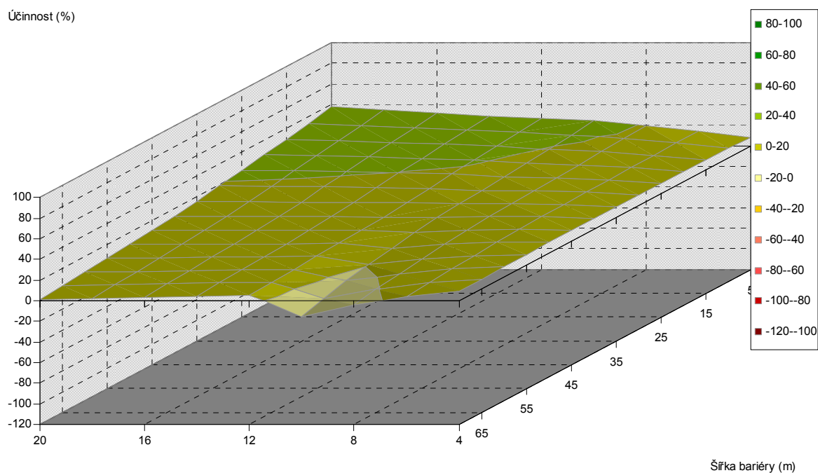
Obr. 5.257. Závislost účinnosti vegetační bariéry na výšce a šířce bariéry, pro vzdálenost od komunikace 80 m, listnaté dřeviny, PM10, 1,5 m nad povrchem
