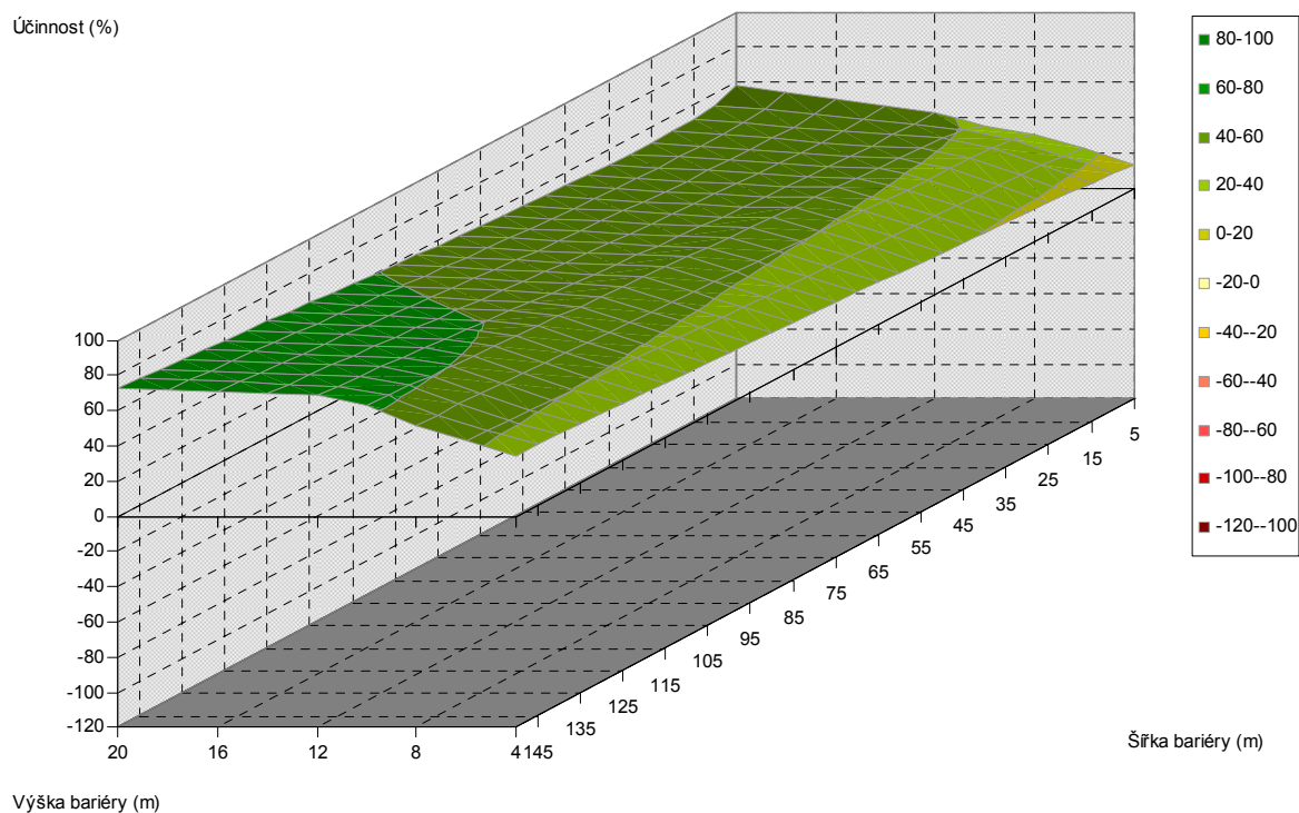
Obr. 5.304. Závislost účinnosti vegetační bariéry na výšce a šířce bariéry, pro vzdálenost od komunikace 240 m, jehličnaté dřeviny, PM10, 3 m nad povrchem
