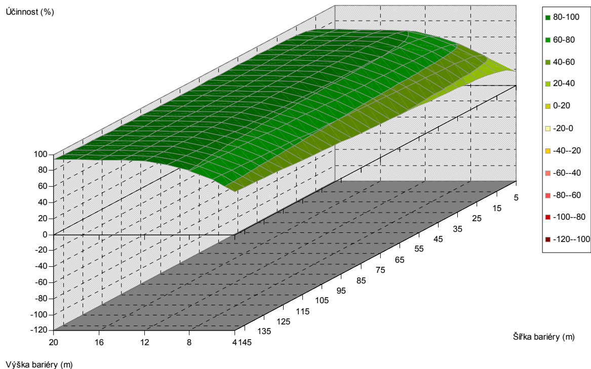
Obr. 5.368. Závislost účinnosti vegetační bariéry na výšce a šířce bariéry, pro vzdálenost od komunikace 220 m, listnaté dřeviny, PM75, 3 m nad povrchem
