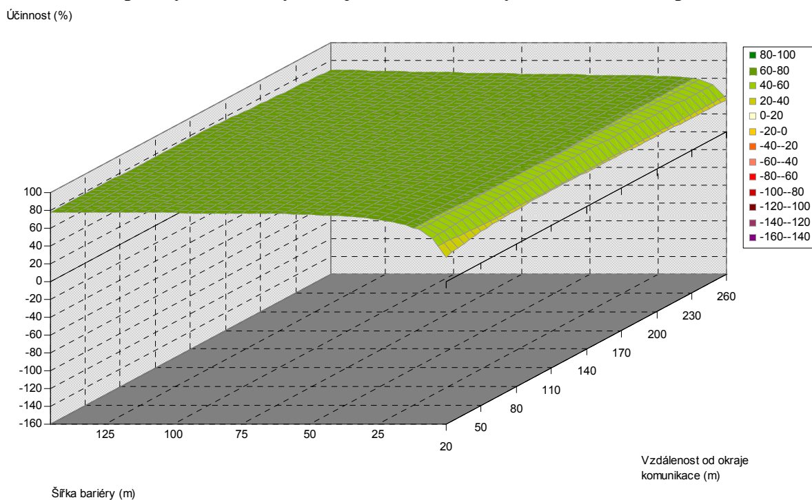
Obr. 5.246. Závislost účinnosti vegetační bariéry na šířce bariéry a vzdálenosti od komunikace, pro výšku bariéry 6 m, jehličnaté dřeviny, PM75, 6 m nad povrchem
