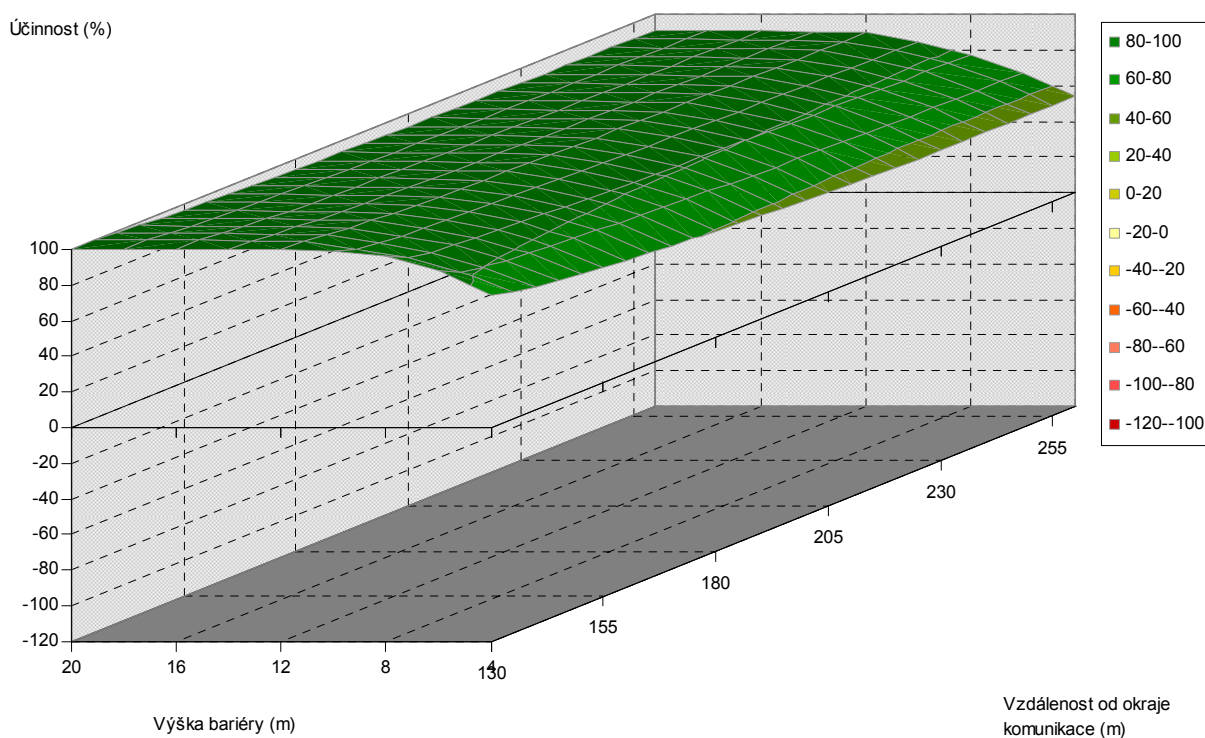
Obr. 5.110. Závislost účinnosti vegetační bariéry na výšce bariéry a vzdálenosti od komunikace, pro šířku bariéry 120 m, jehličnaté dřeviny, PM75, 3 m nad povrchem
