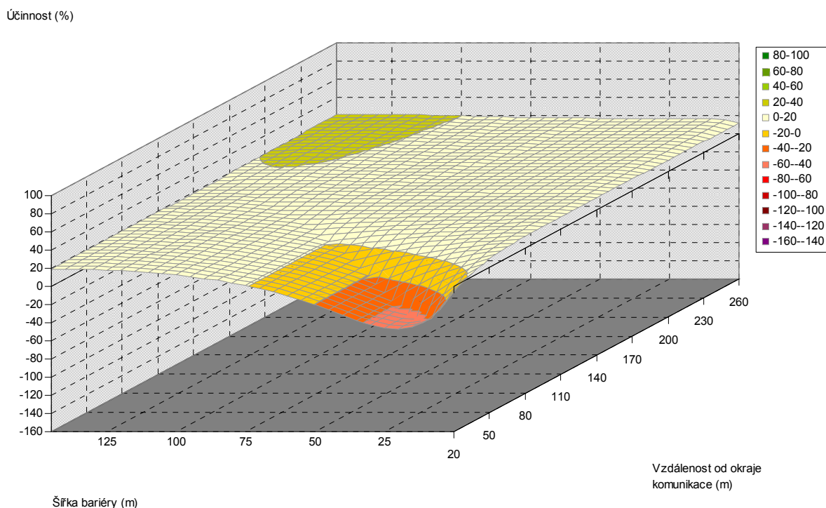
Obr. 5.158. Závislost účinnosti vegetační bariéry na šířce bariéry a vzdálenosti od komunikace, pro výšku bariéry 11 m, listnaté dřeviny, PM10, 3 m nad povrchem
