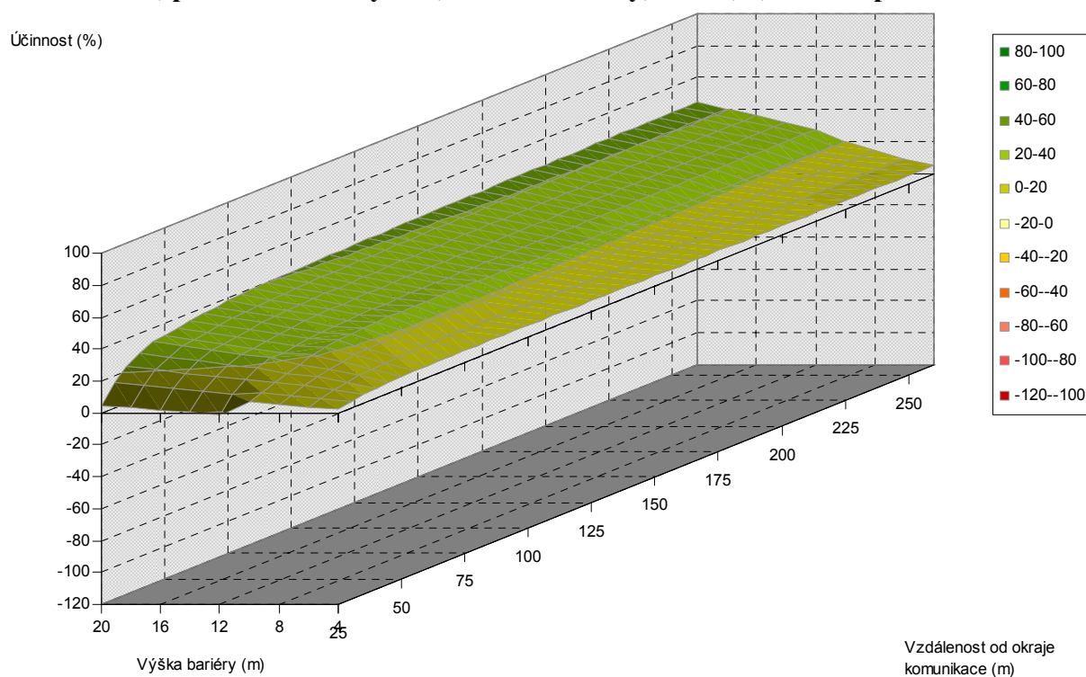
Obr. 5.2. Závislost účinnosti vegetační bariéry na výšce bariéry a vzdálenosti od komunikace, pro šířku bariéry 8 m, listnaté dřeviny, PM10, 1,5 m nad povrchem
