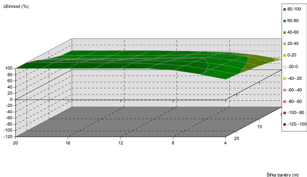
Obr. 5.346. Závislost účinnosti vegetační bariéry na výšce a šířce bariéry, pro vzdálenost od komunikace 40 m, jehličnaté dřeviny, PM75, 1,5 m nad povrchem
