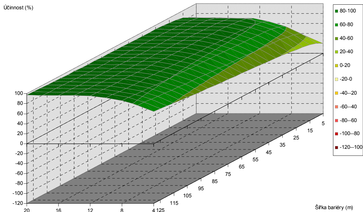
Obr. 5.338. Závislost účinnosti vegetační bariéry na výšce a šířce bariéry, pro vzdálenost od komunikace 140 m, listnaté dřeviny, PM75, 1,5 m nad povrchem
