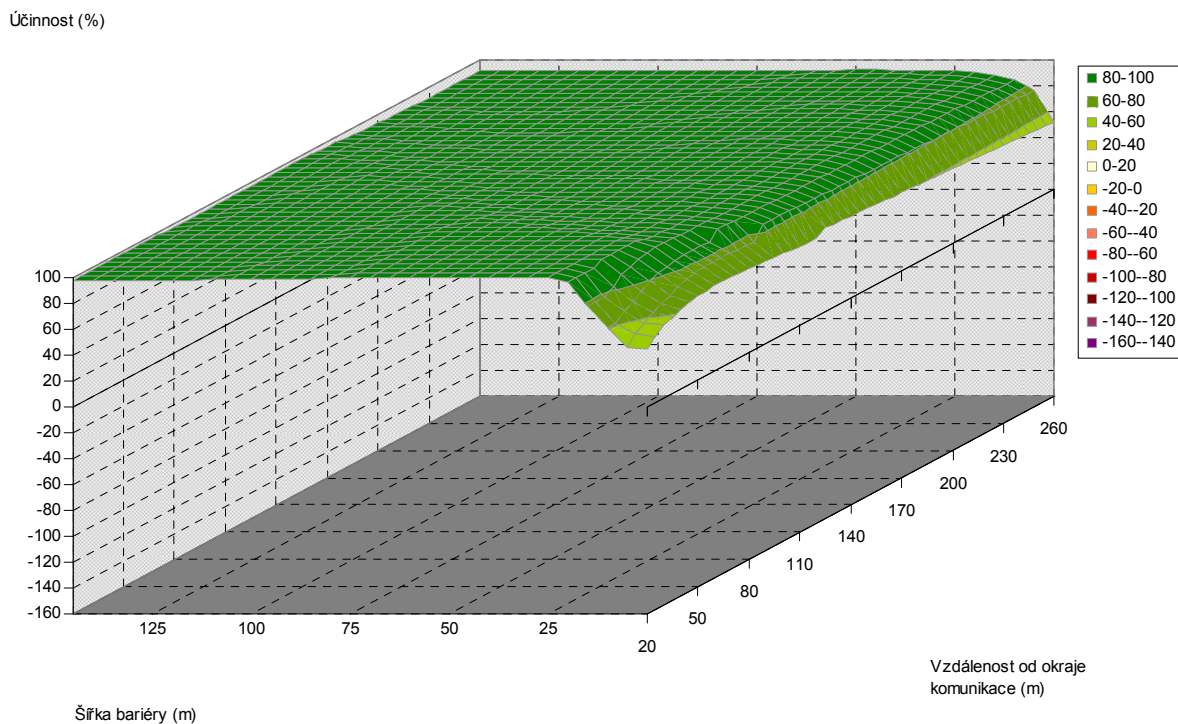
Obr. 5.210. Závislost účinnosti vegetační bariéry na šířce bariéry a vzdálenosti od komunikace, pro výšku bariéry 15 m, jehličnaté dřeviny, PM75, 1,5 m nad povrchem
