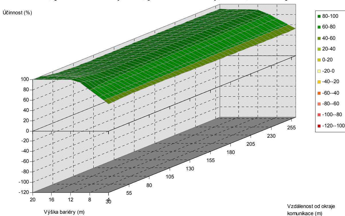
Obr. 5.126. Závislost účinnosti vegetační bariéry na výšce bariéry a vzdálenosti od komunikace, pro šířku bariéry 24 m, jehličnaté dřeviny, PM75, 6 m nad povrchem
