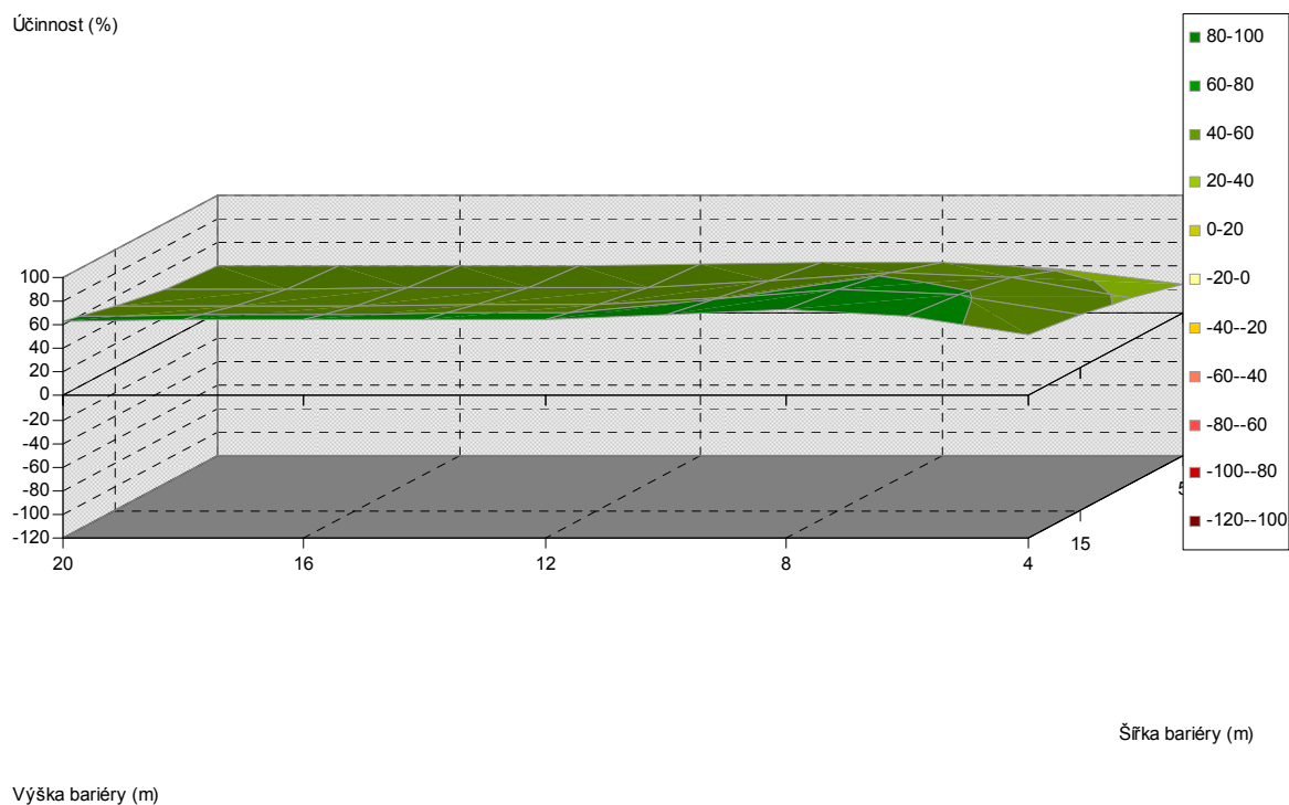
Obr. 5.332. Závislost účinnosti vegetační bariéry na výšce a šířce bariéry, pro vzdálenost od komunikace 30 m, listnaté dřeviny, PM75, 1,5 m nad povrchem
