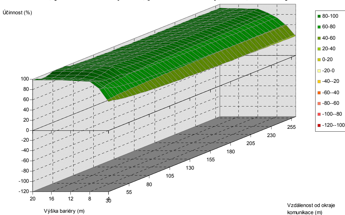
Obr. 5.104. Závislost účinnosti vegetační bariéry na výšce bariéry a vzdálenosti od komunikace, pro šířku bariéry 24 m, jehličnaté dřeviny, PM75, 3 m nad povrchem
