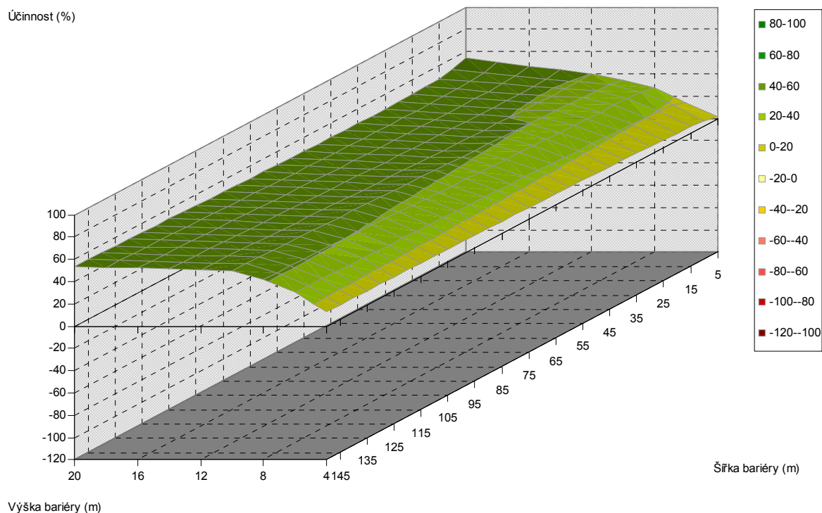
Obr. 5.328. Závislost účinnosti vegetační bariéry na výšce a šířce bariéry, pro vzdálenost od komunikace 200 m, jehličnaté dřeviny, PM10, 6 m nad povrchem
