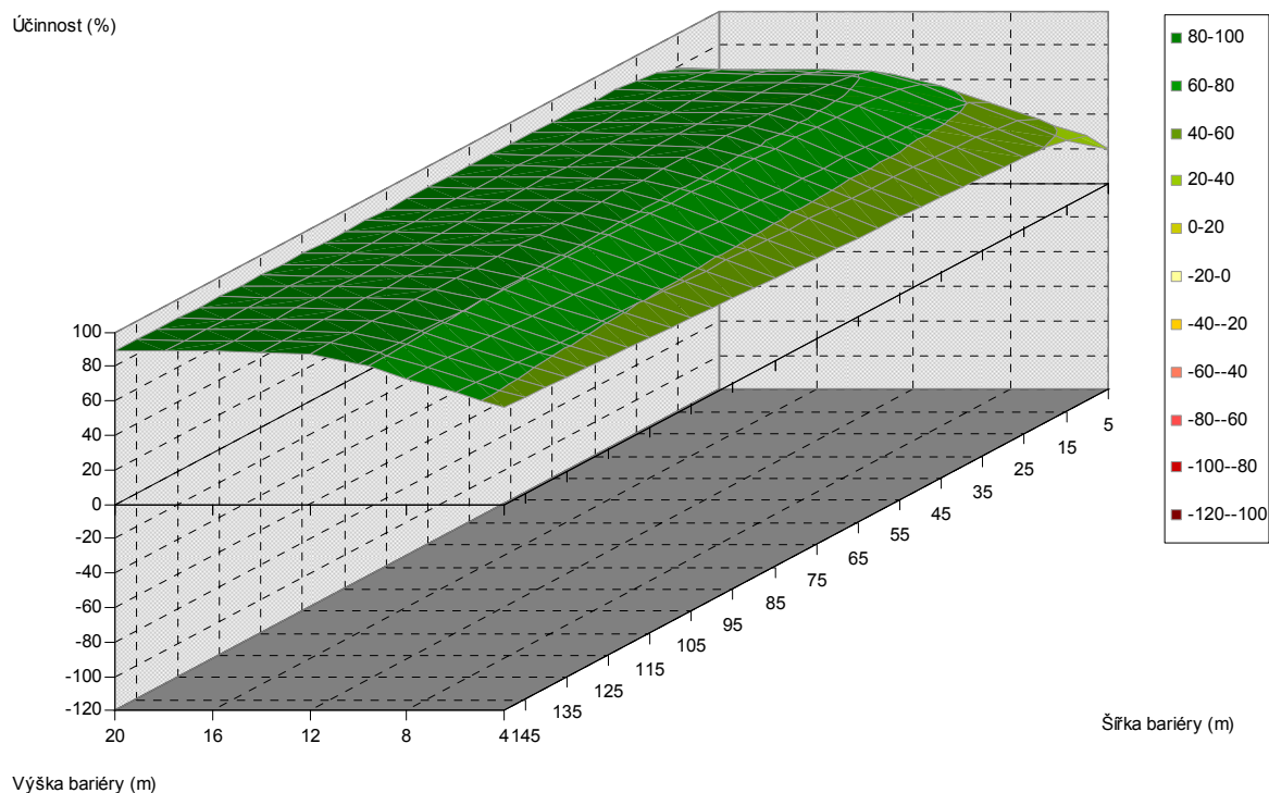
Obr. 5.396. Závislost účinnosti vegetační bariéry na výšce a šířce bariéry, pro vzdálenost od komunikace 20 m, jehličnaté dřeviny, PM75, 6 m nad povrchem
