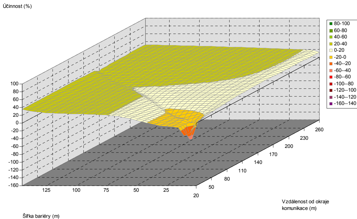
Obr. 5.186. Závislost účinnosti vegetační bariéry na šířce bariéry a vzdálenosti od komunikace, pro výšku bariéry 6 m, jehličnaté dřeviny, PM10, 6 m nad povrchem
