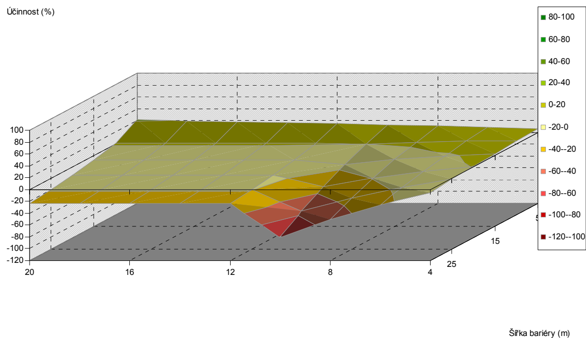
Obr. 5.255. Závislost účinnosti vegetační bariéry na výšce a šířce bariéry, pro vzdálenost od komunikace 40 m, listnaté dřeviny, PM10, 1,5 m nad povrchem
