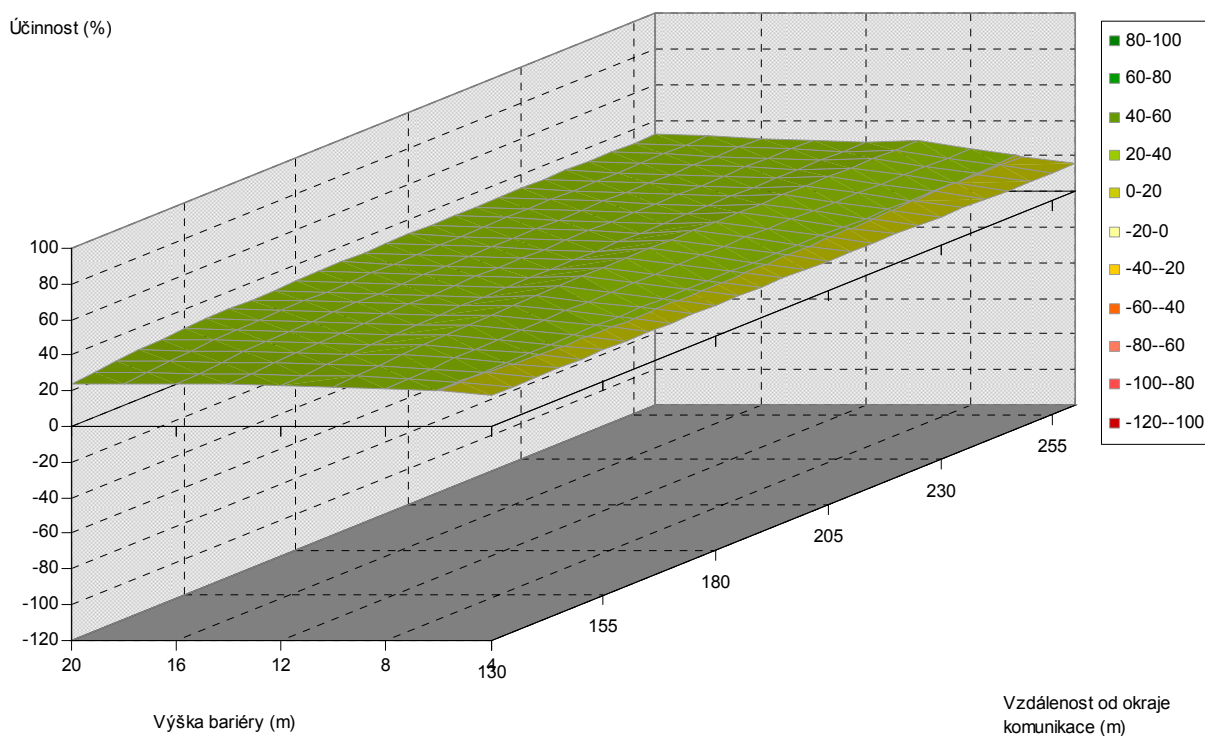
Obr. 5.12. Závislost účinnosti vegetační bariéry na výšce bariéry a vzdálenosti od komunikace, pro šířku bariéry 4 m, jehličnaté dřeviny, PM10, 1,5 m nad povrchem
