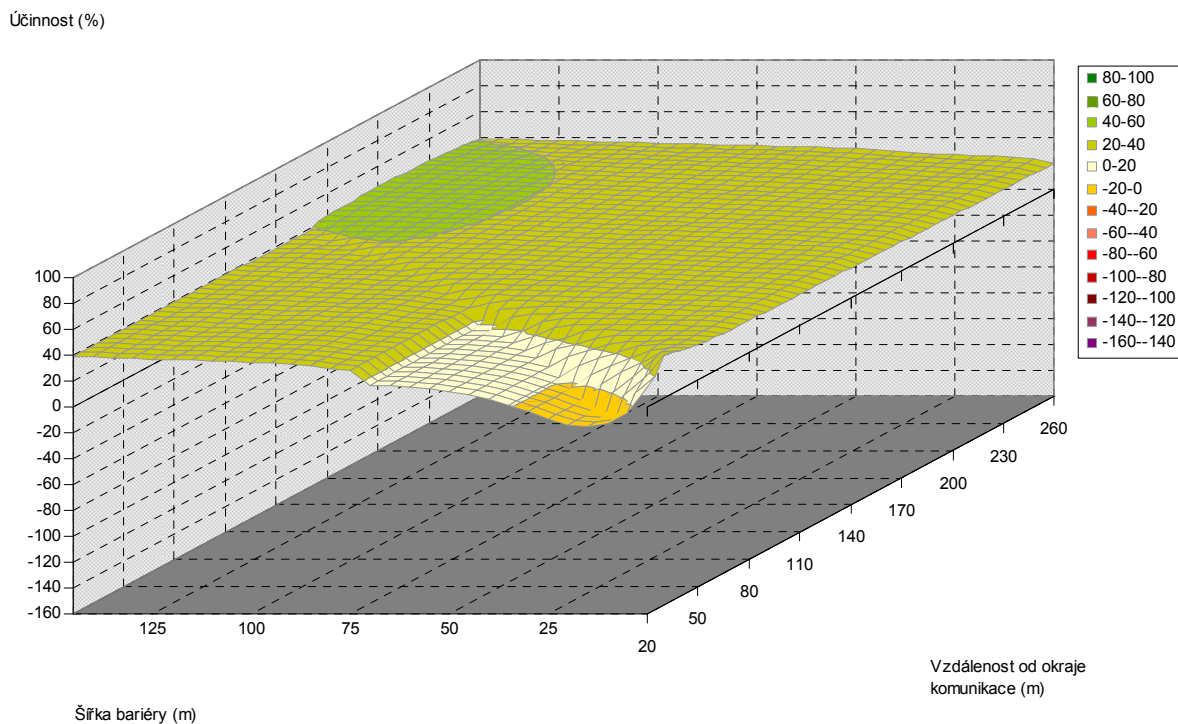
Obr. 5.146. Závislost účinnosti vegetační bariéry na šířce bariéry a vzdálenosti od komunikace, pro výšku bariéry 6 m, jehličnaté dřeviny, PM10, 1,5 m nad povrchem
