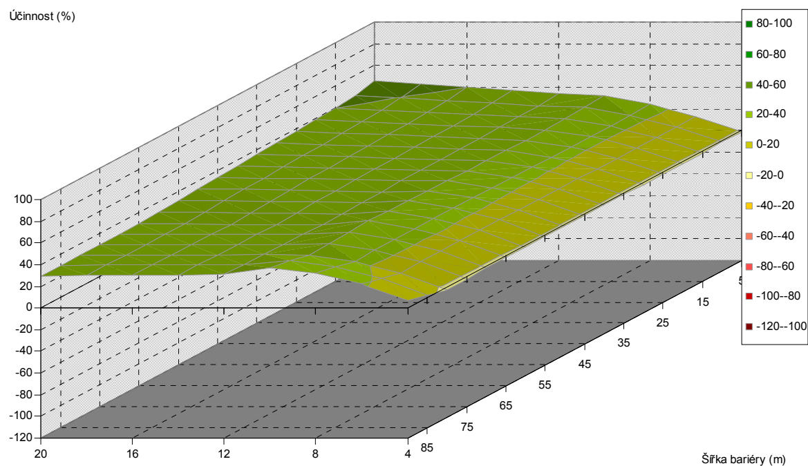
Obr. 5.323. Závislost účinnosti vegetační bariéry na výšce a šířce bariéry, pro vzdálenost od komunikace 100 m, jehličnaté dřeviny, PM10, 6 m nad povrchem
