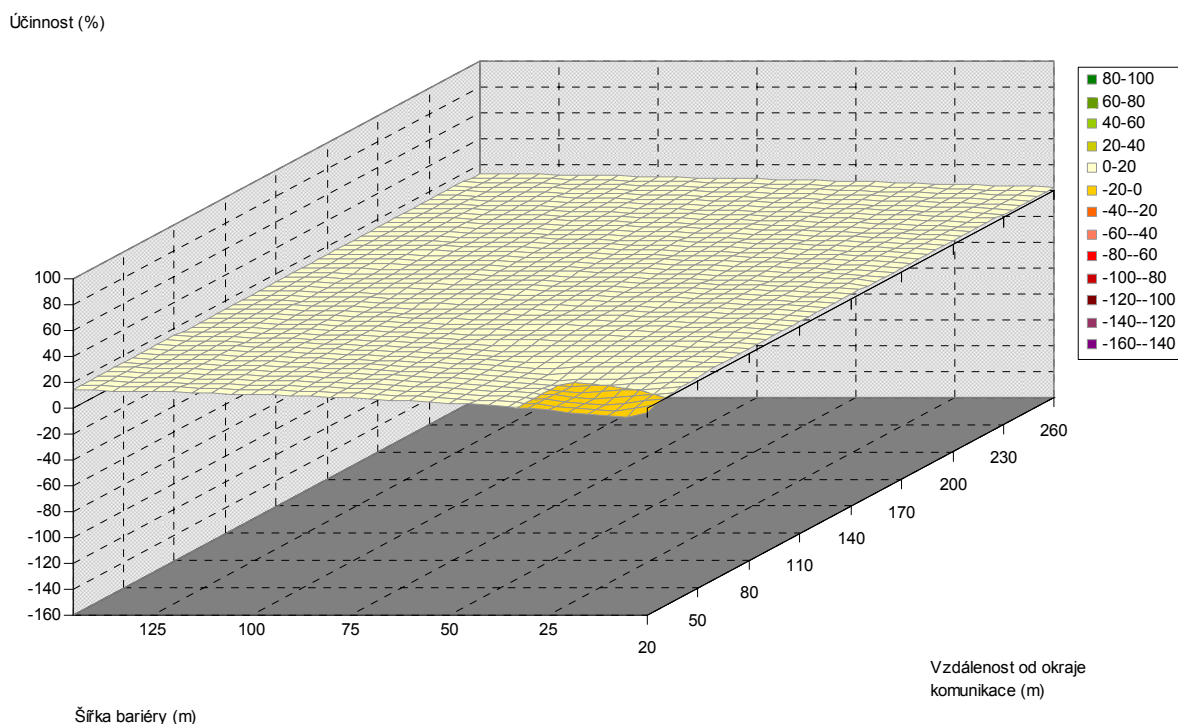
Obr. 5.154. Závislost účinnosti vegetační bariéry na šířce bariéry a vzdálenosti od komunikace, pro výšku bariéry 4 m, listnaté dřeviny, PM10, 3 m nad povrchem
