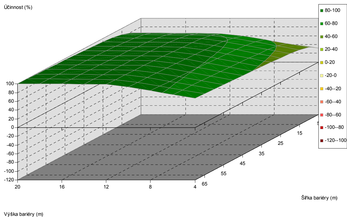
Obr. 5.400. Závislost účinnosti vegetační bariéry na výšce a šířce bariéry, pro vzdálenost od komunikace 80 m, jehličnaté dřeviny, PM75, 6 m nad povrchem
