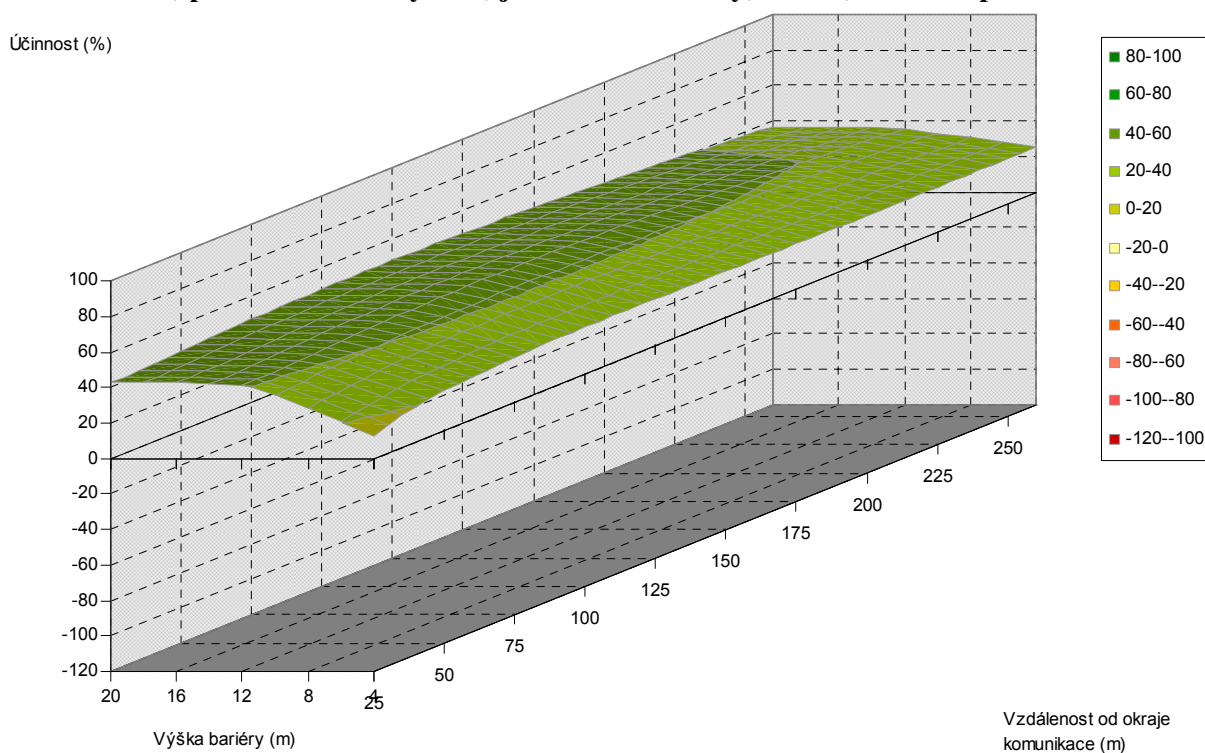
Obr. 5.122. Závislost účinnosti vegetační bariéry na výšce bariéry a vzdálenosti od komunikace, pro šířku bariéry 4 m, jehličnaté dřeviny, PM75, 6 m nad povrchem
