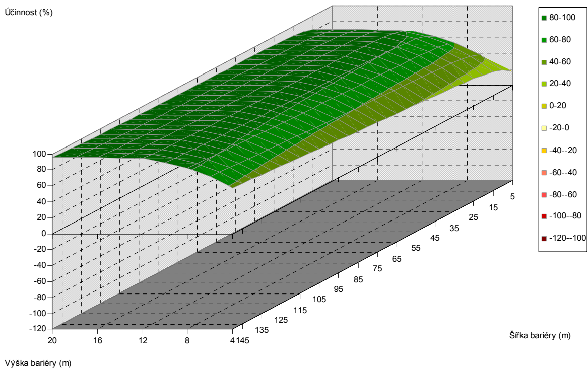
Obr. 5.366. Závislost účinnosti vegetační bariéry na výšce a šířce bariéry, pro vzdálenost od komunikace 180 m, listnaté dřeviny, PM75, 3 m nad povrchem
