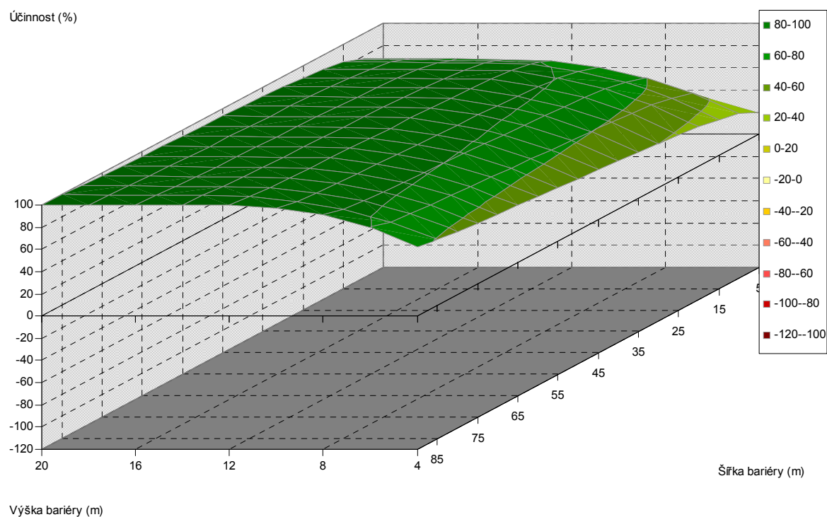
Obr. 5.362. Závislost účinnosti vegetační bariéry na výšce a šířce bariéry, pro vzdálenost od komunikace 100 m, listnaté dřeviny, PM75, 3 m nad povrchem
