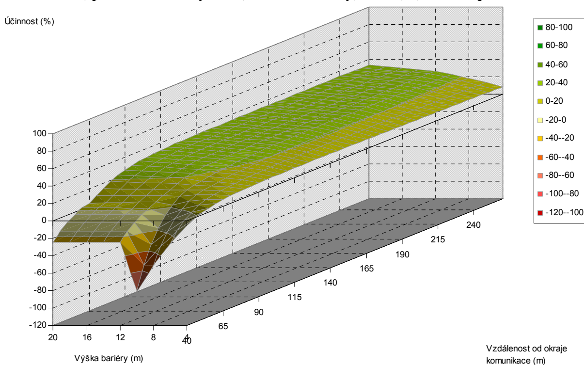
Obr. 5.6. Závislost účinnosti vegetační bariéry na výšce bariéry a vzdálenosti od komunikace, pro šířku bariéry 30 m, listnaté dřeviny, PM10, 1,5 m nad povrchem
