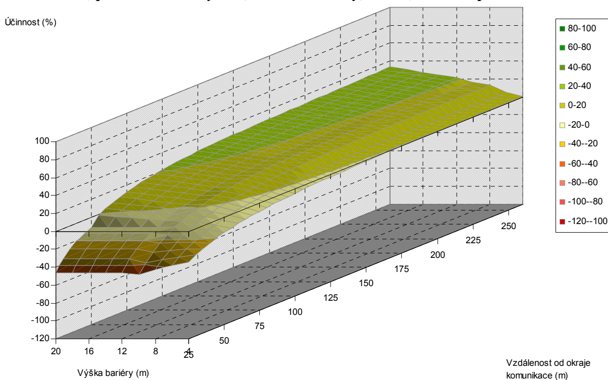
Obr. 5.46. Závislost účinnosti vegetační bariéry na výšce bariéry a vzdálenosti od komunikace, pro šířku bariéry 8 m, listnaté dřeviny, PM10, 6 m nad povrchem
