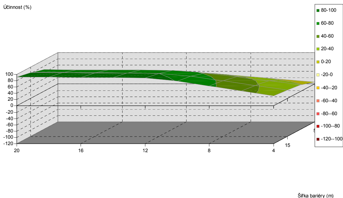
Obr. 5.384. Závislost účinnosti vegetační bariéry na výšce a šířce bariéry, pro vzdálenost od komunikace 30 m, listnaté dřeviny, PM75, 6 m nad povrchem
