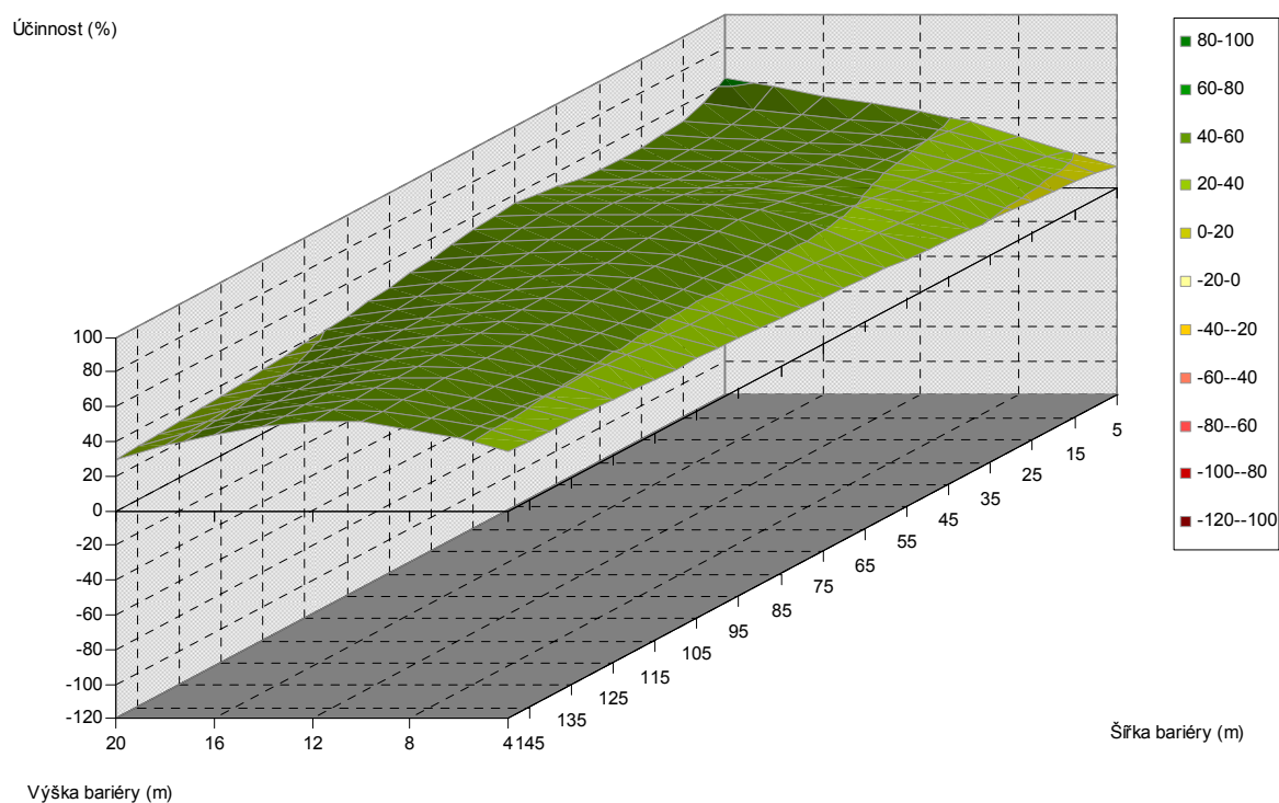
Obr. 5.278. Závislost účinnosti vegetační bariéry na výšce a šířce bariéry, pro vzdálenost od komunikace 240 m, jehličnaté dřeviny, PM10, 1,5 m nad povrchem
