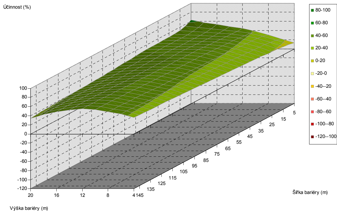
Obr. 5.276. Závislost účinnosti vegetační bariéry na výšce a šířce bariéry, pro vzdálenost od komunikace 200 m, jehličnaté dřeviny, PM10, 1,5 m nad povrchem
