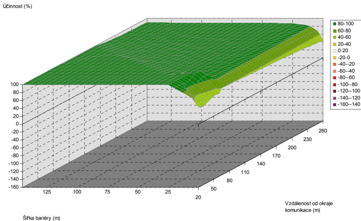
Obr. 5.220. Závislost účinnosti vegetační bariéry na šířce bariéry a vzdálenosti od komunikace, pro výšku bariéry 15 m, listnaté dřeviny, PM75, 3 m nad povrchem
