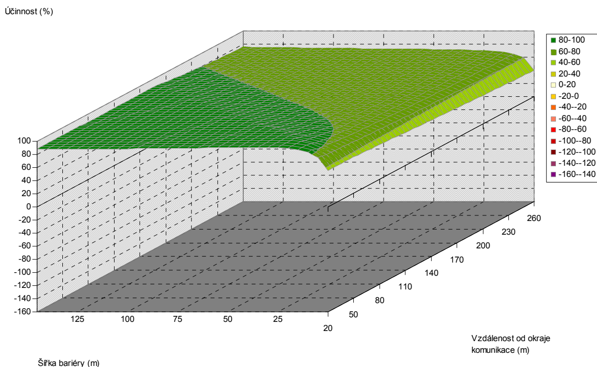
Obr. 5.208. Závislost účinnosti vegetační bariéry na šířce bariéry a vzdálenosti od komunikace, pro výšku bariéry 11 m, jehličnaté dřeviny, PM75, 1,5 m nad povrchem
