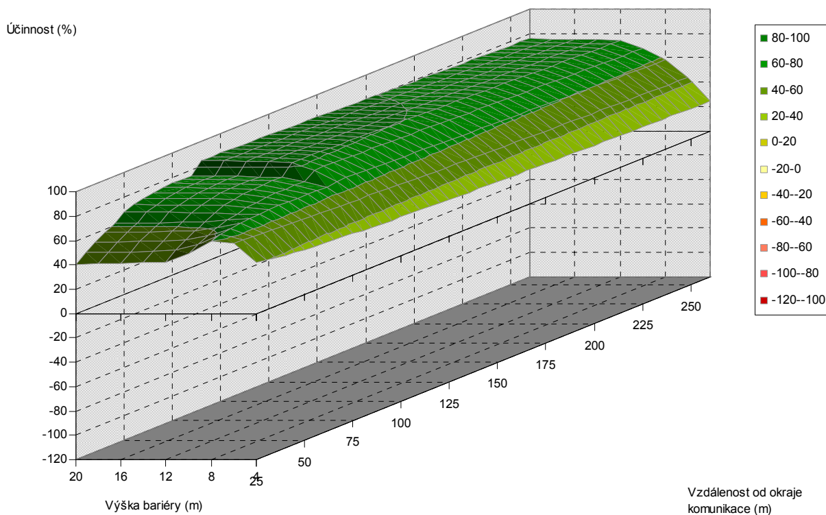
Obr. 5.70. Závislost účinnosti vegetační bariéry na výšce bariéry a vzdálenosti od komunikace, pro šířku bariéry 18 m, listnaté dřeviny, PM75, 1,5 m nad povrchem
