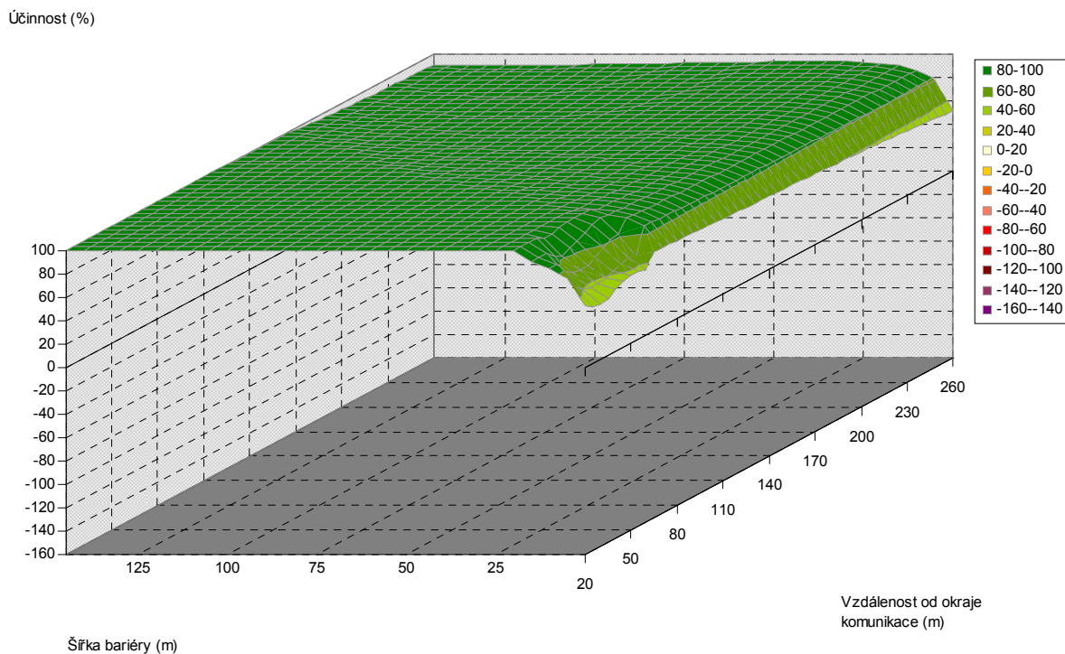
Obr. 5.232. Závislost účinnosti vegetační bariéry na šířce bariéry a vzdálenosti od komunikace, pro výšku bariéry 20 m, jehličnaté dřeviny, PM75, 3 m nad povrchem
