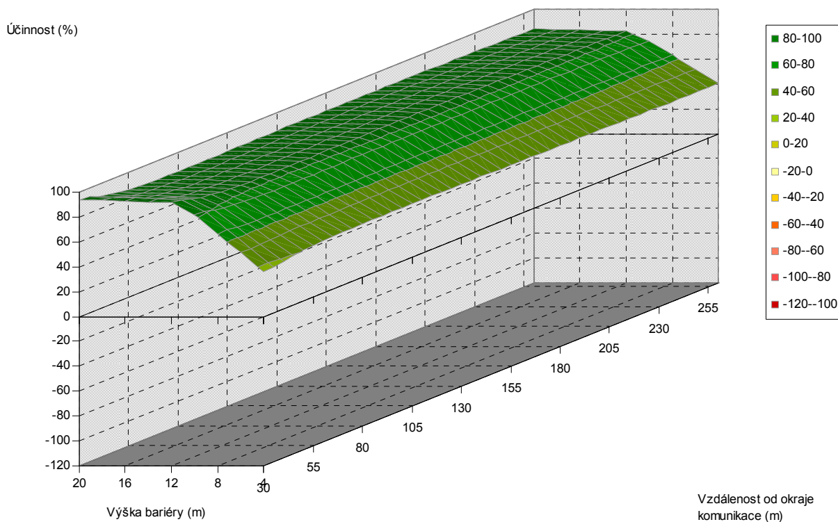
Obr. 5.116. Závislost účinnosti vegetační bariéry na výšce bariéry a vzdálenosti od komunikace, pro šířku bariéry 30 m, listnaté dřeviny, PM75, 6 m nad povrchem
