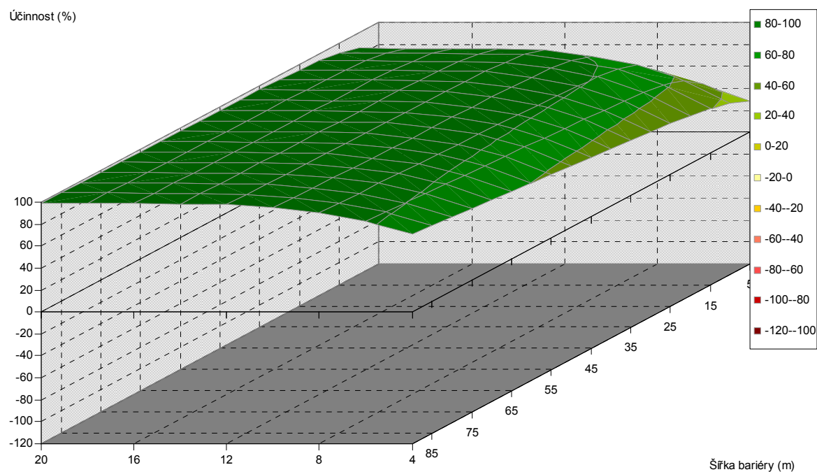
Obr. 5.349. Závislost účinnosti vegetační bariéry na výšce a šířce bariéry, pro vzdálenost od komunikace 100 m, jehličnaté dřeviny, PM75, 1,5 m nad povrchem
