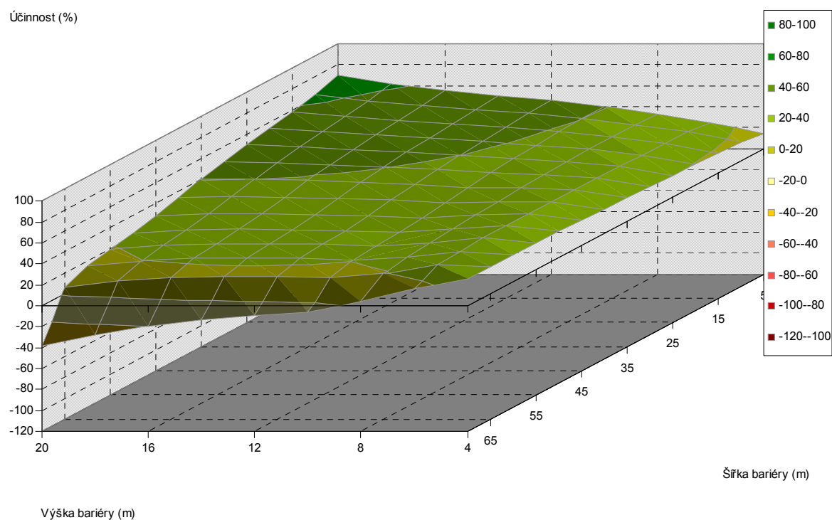
Obr. 5.270. Závislost účinnosti vegetační bariéry na výšce a šířce bariéry, pro vzdálenost od komunikace 80 m, jehličnaté dřeviny, PM10, 1,5 m nad povrchem
