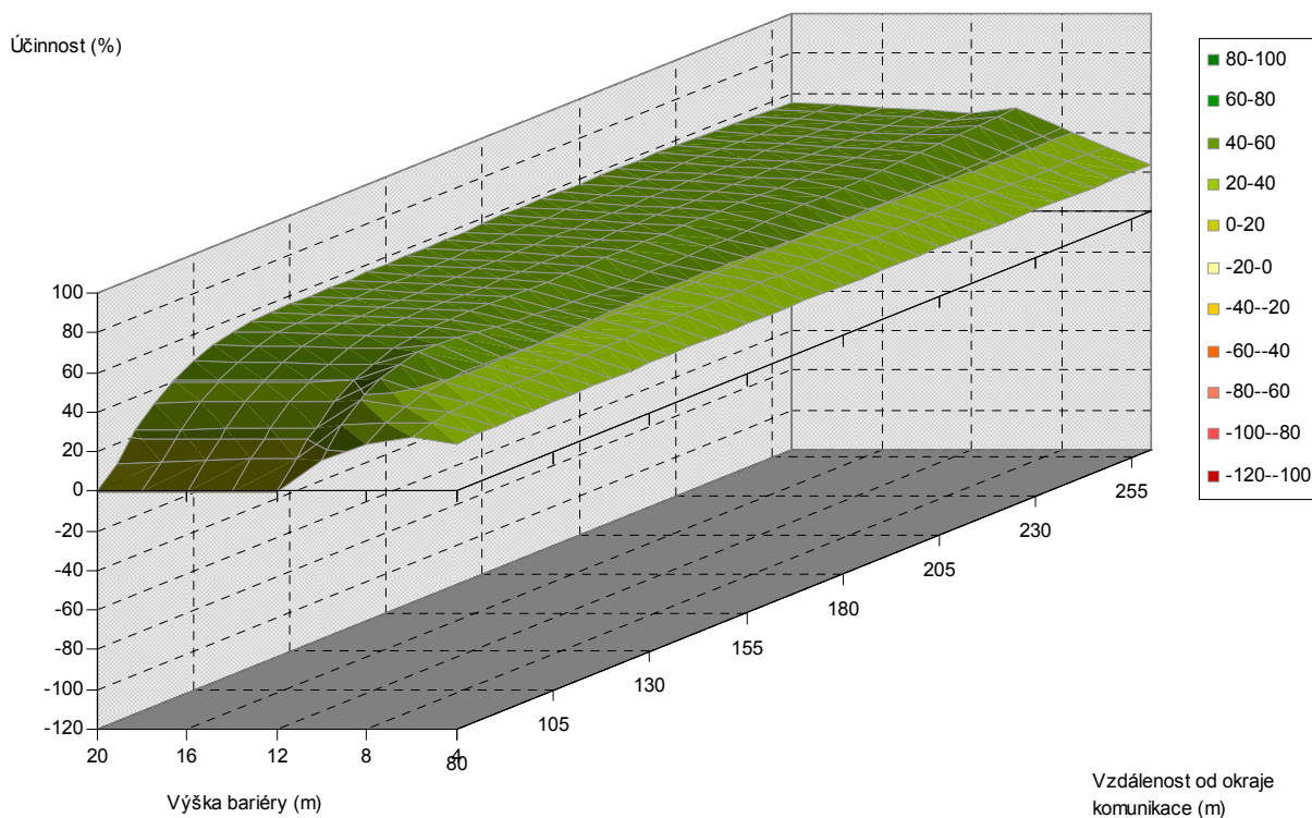
Obr. 5.42. Závislost účinnosti vegetační bariéry na výšce bariéry a vzdálenosti od komunikace, pro šířku bariéry 70 m, jehličnaté dřeviny, PM10, 3 m nad povrchem
