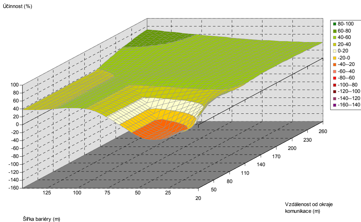
Obr. 5.168. Závislost účinnosti vegetační bariéry na šířce bariéry a vzdálenosti od komunikace, pro výšku bariéry 11 m, jehličnaté dřeviny, PM10, 3 m nad povrchem
