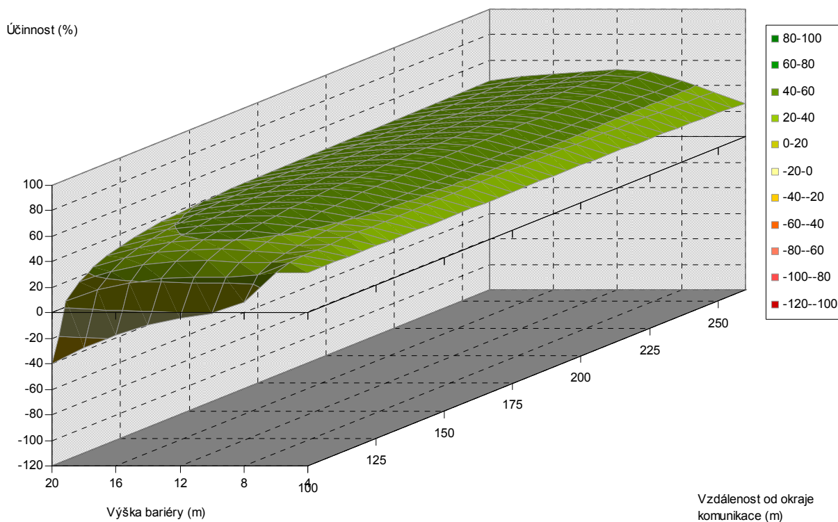
Obr. 5.22. Závislost účinnosti vegetační bariéry na výšce bariéry a vzdálenosti od komunikace, pro šířku bariéry 120 m, jehličnaté dřeviny, PM10, 1,5 m nad povrchem
