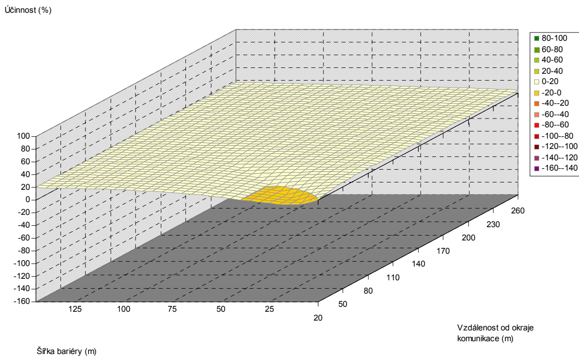
Obr. 5.134. Závislost účinnosti vegetační bariéry na šířce bariéry a vzdálenosti od komunikace, pro výšku bariéry 4 m, listnaté dřeviny, PM10, 1,5 m nad povrchem
