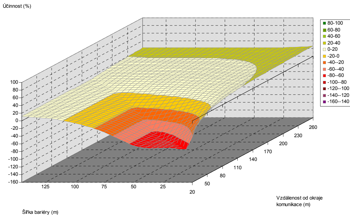
Obr. 5.180. Závislost účinnosti vegetační bariéry na šířce bariéry a vzdálenosti od komunikace, pro výšku bariéry 15 m, listnaté dřeviny, PM10, 6 m nad povrchem
