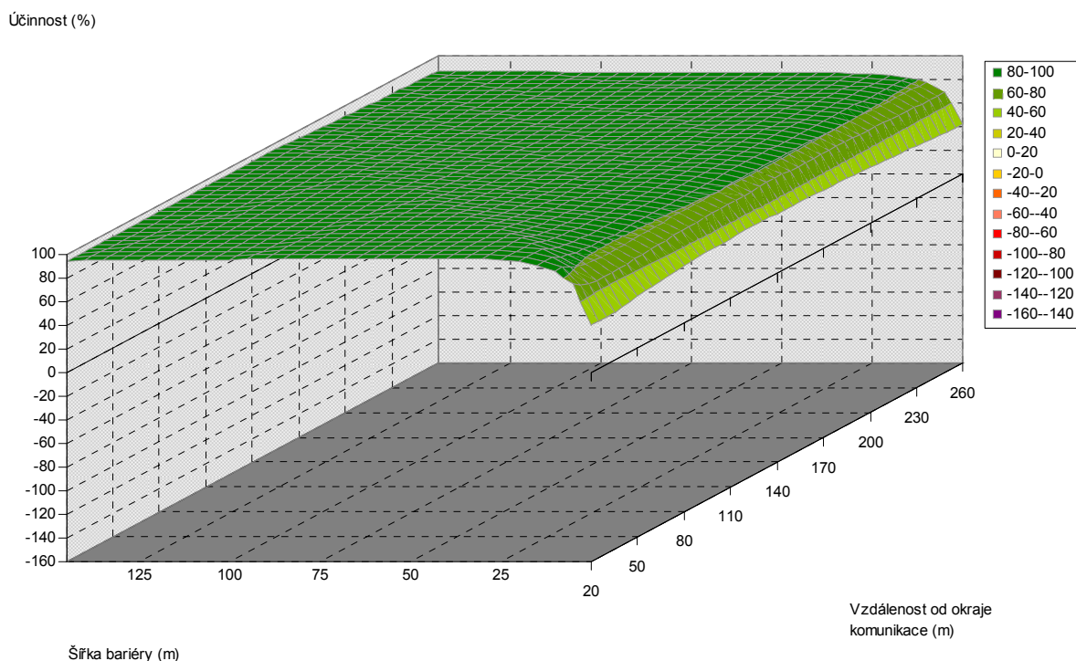
Obr. 5.242. Závislost účinnosti vegetační bariéry na šířce bariéry a vzdálenosti od komunikace, pro výšku bariéry 20 m, listnaté dřeviny, PM75, 6 m nad povrchem
