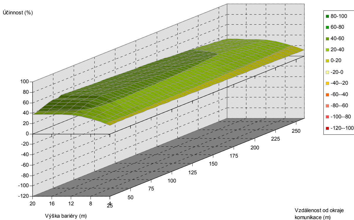
Obr. 5.90. Závislost účinnosti vegetační bariéry na výšce bariéry a vzdálenosti od komunikace, pro šířku bariéry 8 m, listnaté dřeviny, PM75, 3 m nad povrchem
