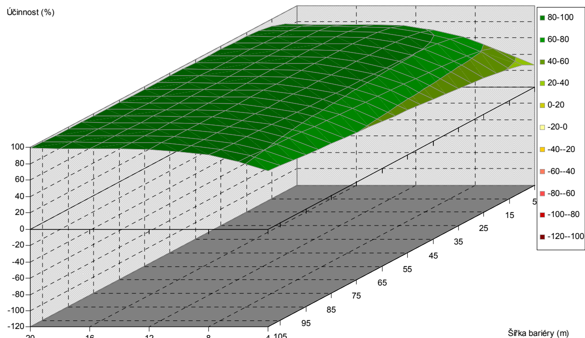
Obr. 5.350. Závislost účinnosti vegetační bariéry na výšce a šířce bariéry, pro vzdálenost od komunikace 120 m, jehličnaté dřeviny, PM75, 1,5 m nad povrchem
