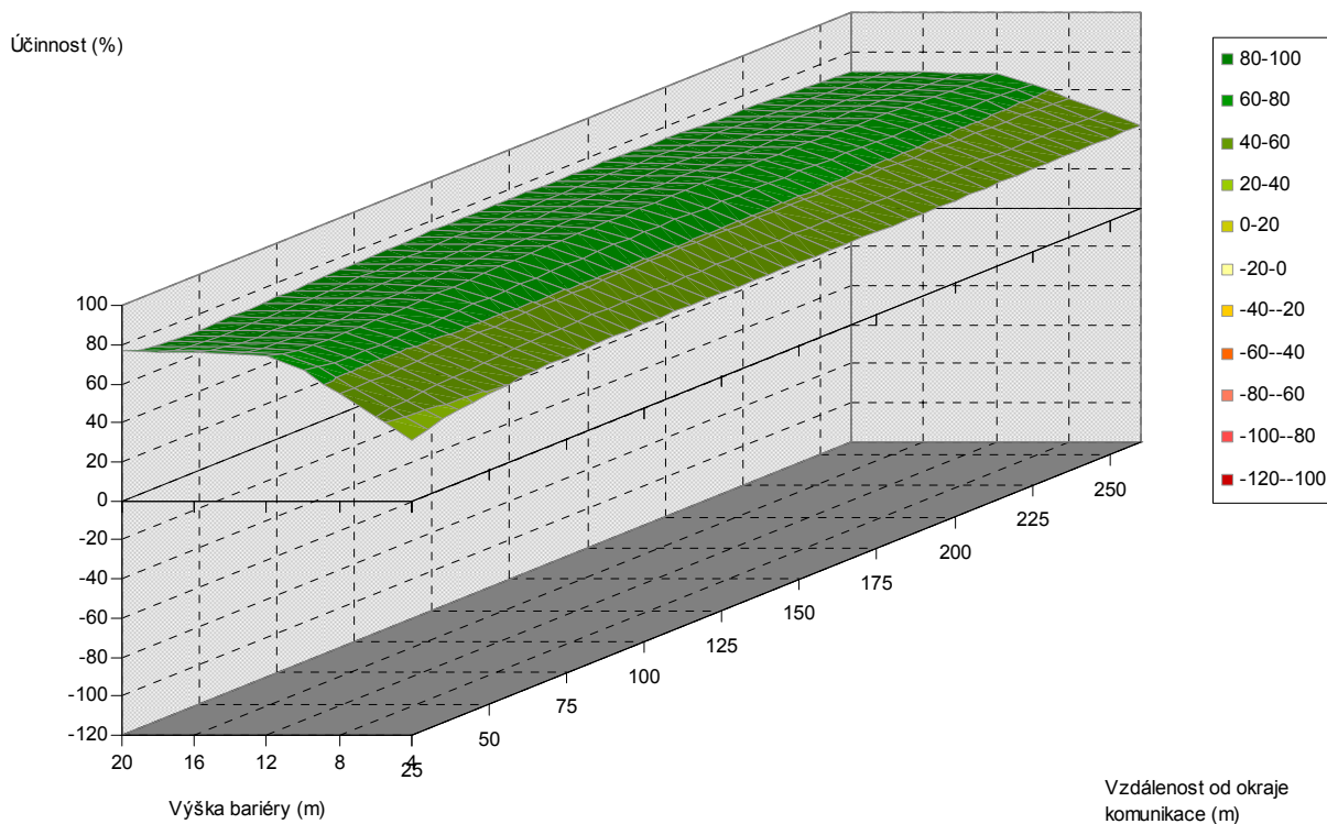
Obr. 5.124. Závislost účinnosti vegetační bariéry na výšce bariéry a vzdálenosti od komunikace, pro šířku bariéry 12 m, jehličnaté dřeviny, PM75, 6 m nad povrchem
