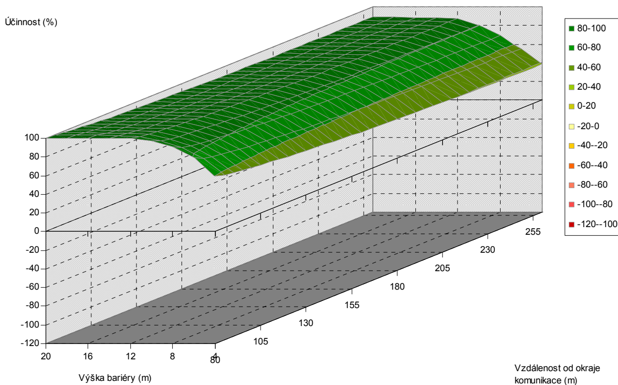
Obr. 5.98. Závislost účinnosti vegetační bariéry na výšce bariéry a vzdálenosti od komunikace, pro šířku bariéry 90 m, listnaté dřeviny, PM75, 3 m nad povrchem
