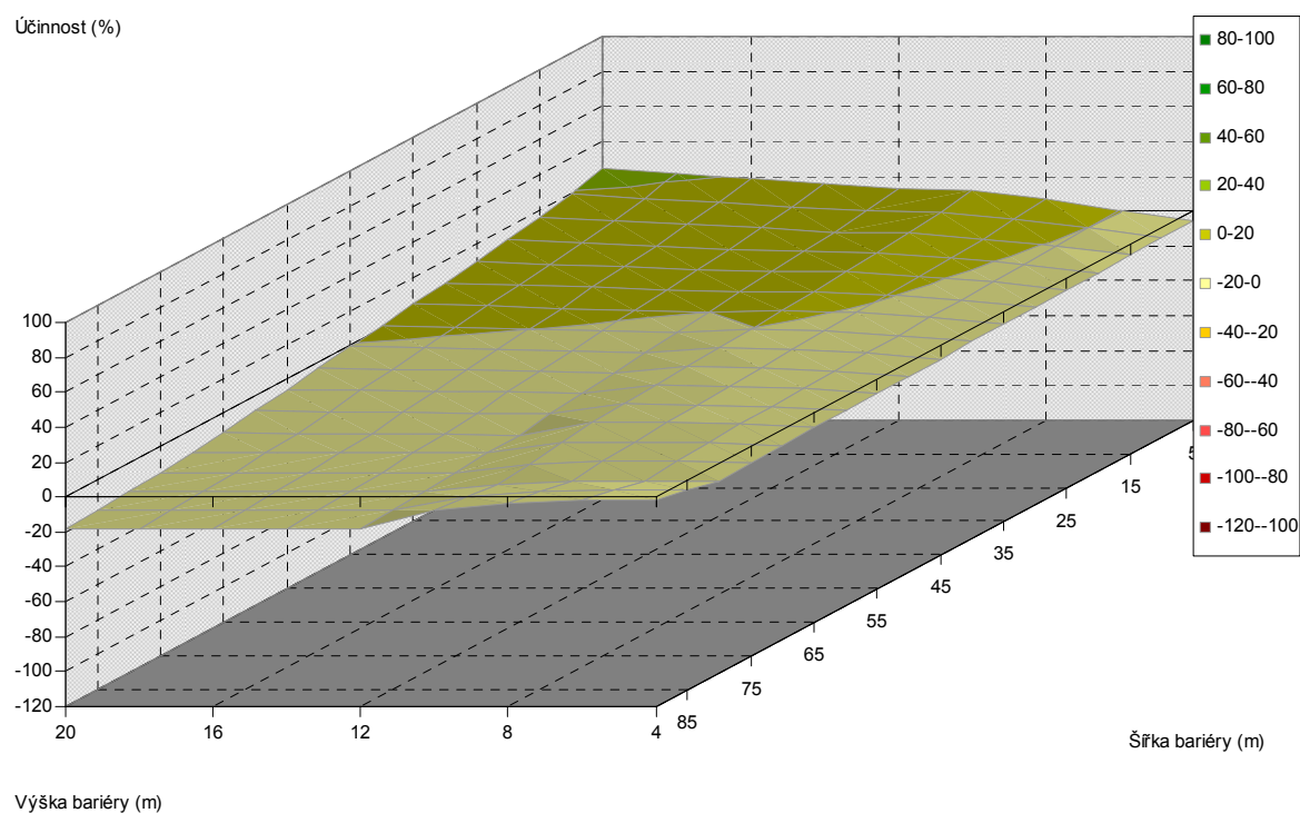
Obr. 5.310. Závislost účinnosti vegetační bariéry na výšce a šířce bariéry, pro vzdálenost od komunikace 100 m, listnaté dřeviny, PM10, 6 m nad povrchem
