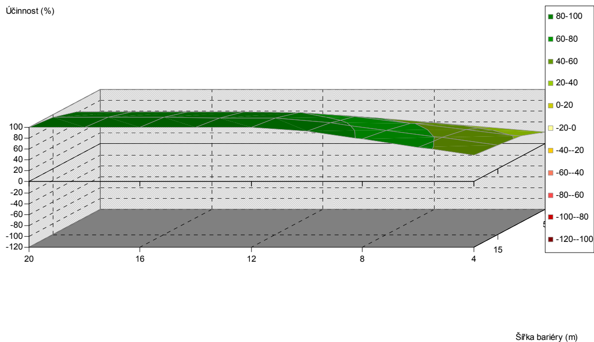
Obr. 5.397. Závislost účinnosti vegetační bariéry na výšce a šířce bariéry, pro vzdálenost od komunikace 30 m, jehličnaté dřeviny, PM75, 6 m nad povrchem
