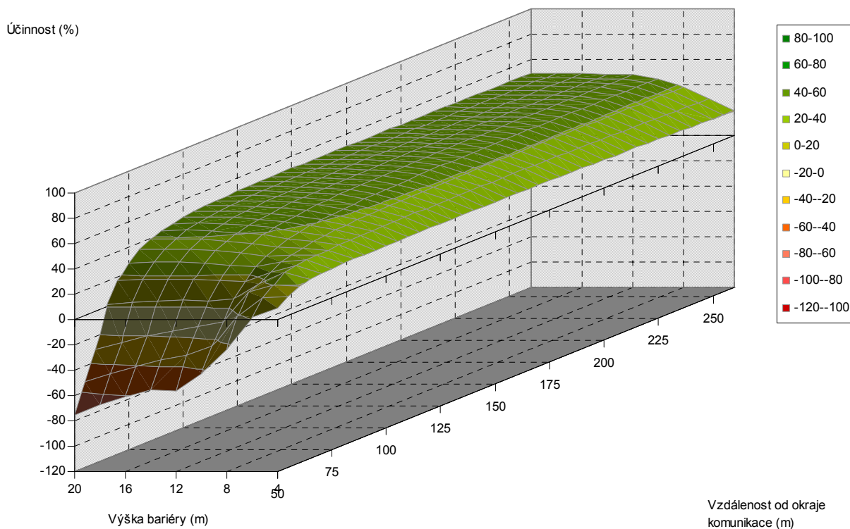
Obr. 5.18. Závislost účinnosti vegetační bariéry na výšce bariéry a vzdálenosti od komunikace, pro šířku bariéry 40 m, jehličnaté dřeviny, PM10, 1,5 m nad povrchem
