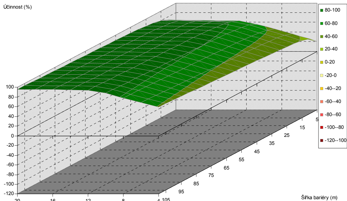
Obr. 5.389. Závislost účinnosti vegetační bariéry na výšce a šířce bariéry, pro vzdálenost od komunikace 120 m, listnaté dřeviny, PM75, 6 m nad povrchem
