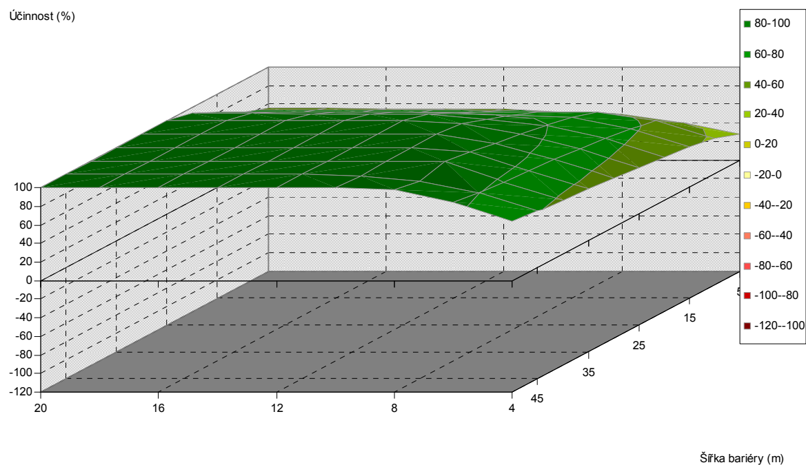
Obr. 5.373. Závislost účinnosti vegetační bariéry na výšce a šířce bariéry, pro vzdálenost od komunikace 60 m, jehličnaté dřeviny, PM75, 3 m nad povrchem
