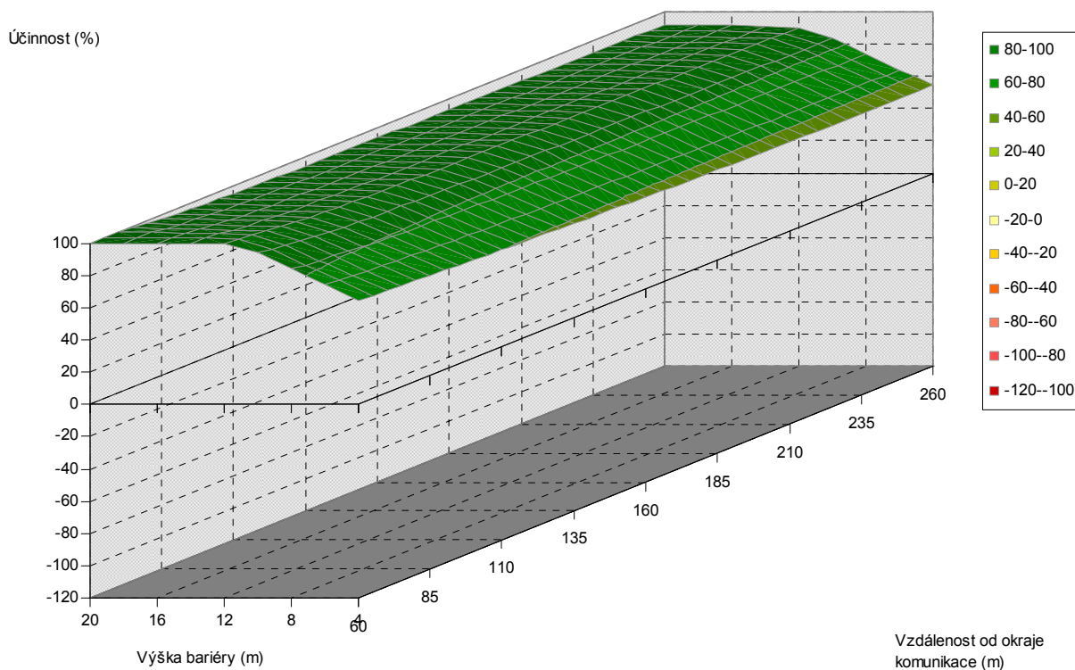
Obr. 5.130. Závislost účinnosti vegetační bariéry na výšce bariéry a vzdálenosti od komunikace, pro šířku bariéry 70 m, jehličnaté dřeviny, PM75, 6 m nad povrchem
