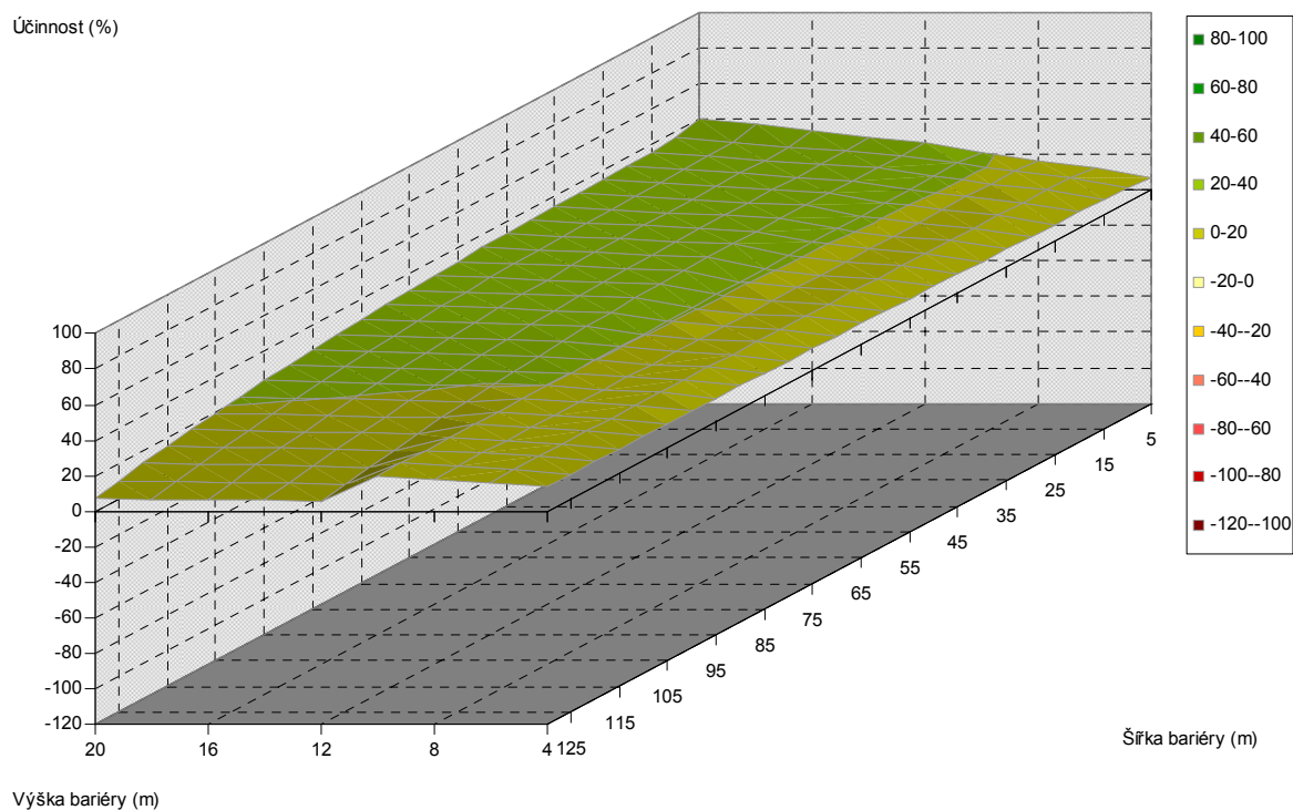
Obr. 5.286. Závislost účinnosti vegetační bariéry na výšce a šířce bariéry, pro vzdálenost od komunikace 140 m, listnaté dřeviny, PM10, 3 m nad povrchem
