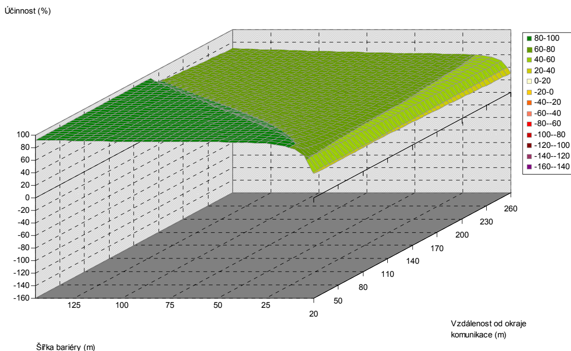
Obr. 5.218. Závislost účinnosti vegetační bariéry na šířce bariéry a vzdálenosti od komunikace, pro výšku bariéry 11 m, listnaté dřeviny, PM75, 3 m nad povrchem
