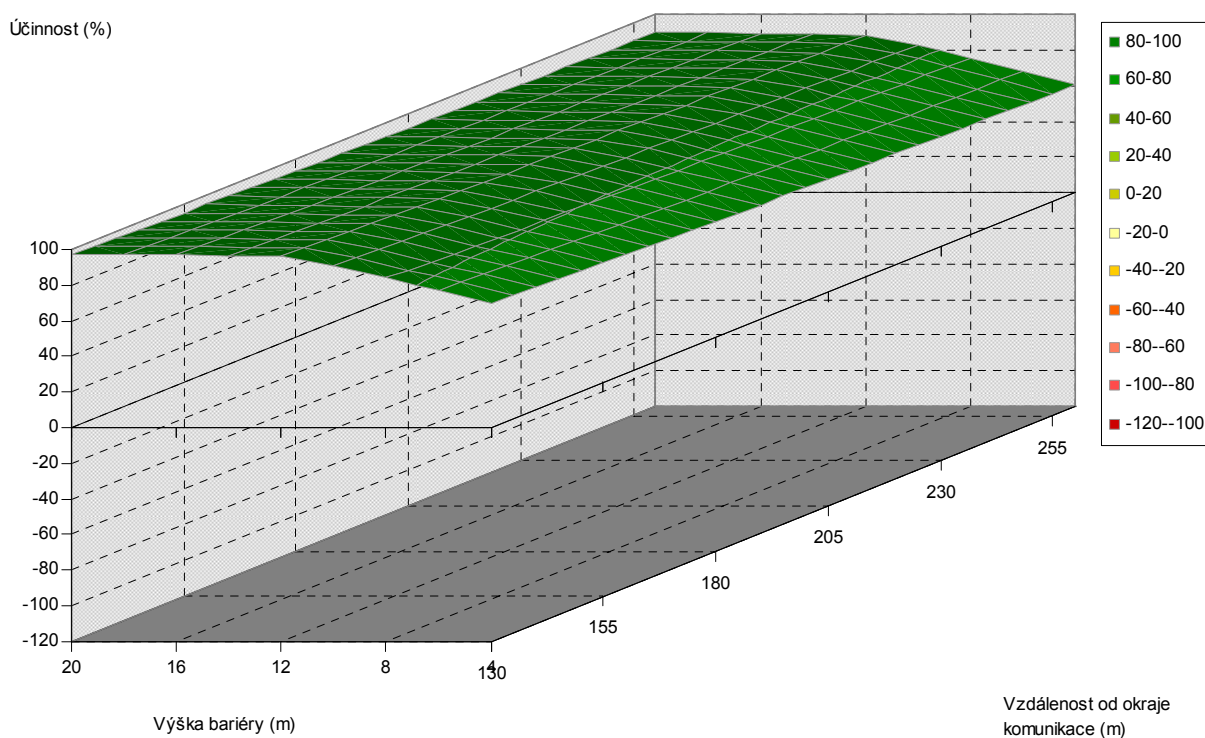
Obr. 5.132. Závislost účinnosti vegetační bariéry na výšce bariéry a vzdálenosti od komunikace, pro šířku bariéry 120 m, jehličnaté dřeviny, PM75, 6 m nad povrchem
