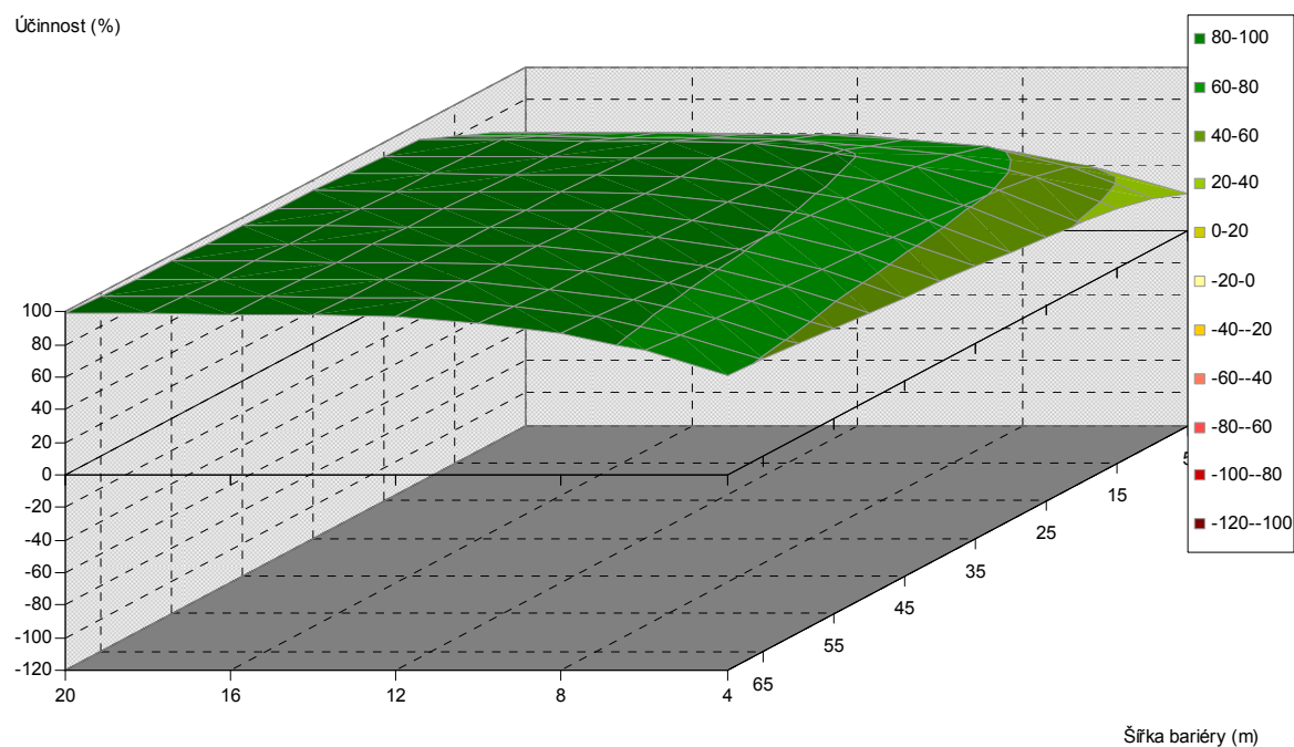
Obr. 5.335. Závislost účinnosti vegetační bariéry na výšce a šířce bariéry, pro vzdálenost od komunikace 80 m, listnaté dřeviny, PM75, 1,5 m nad povrchem
