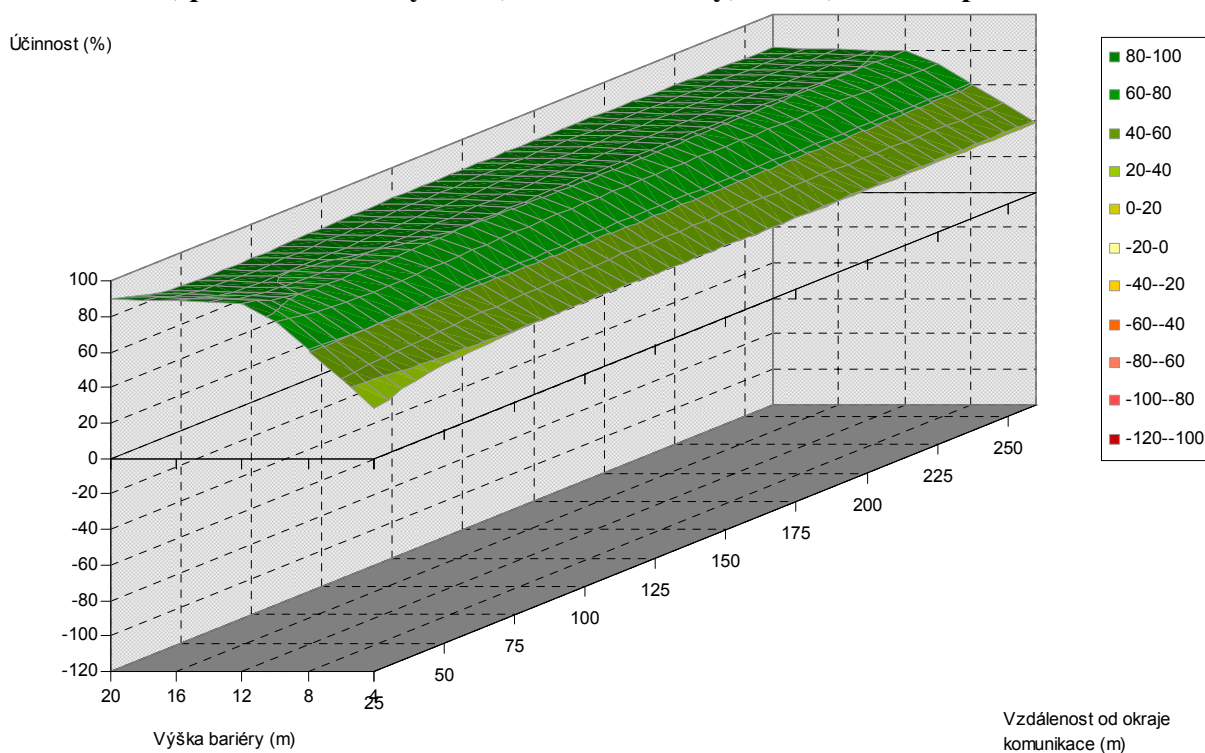
Obr. 5.114. Závislost účinnosti vegetační bariéry na výšce bariéry a vzdálenosti od komunikace, pro šířku bariéry 18 m, listnaté dřeviny, PM75, 6 m nad povrchem
