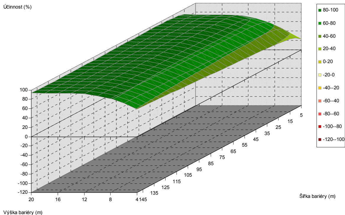
Obr. 5.382. Závislost účinnosti vegetační bariéry na výšce a šířce bariéry, pro vzdálenost od komunikace 240 m, jehličnaté dřeviny, PM75, 3 m nad povrchem
