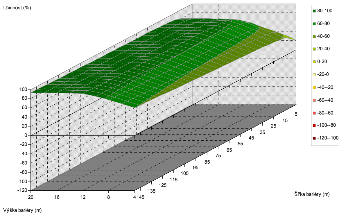
Obr. 5.392. Závislost účinnosti vegetační bariéry na výšce a šířce bariéry, pro vzdálenost od komunikace 180 m, listnaté dřeviny, PM75, 6 m nad povrchem
