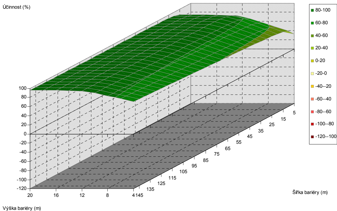
Obr. 5.404. Závislost účinnosti vegetační bariéry na výšce a šířce bariéry, pro vzdálenost od komunikace 160 m, jehličnaté dřeviny, PM75, 6 m nad povrchem
