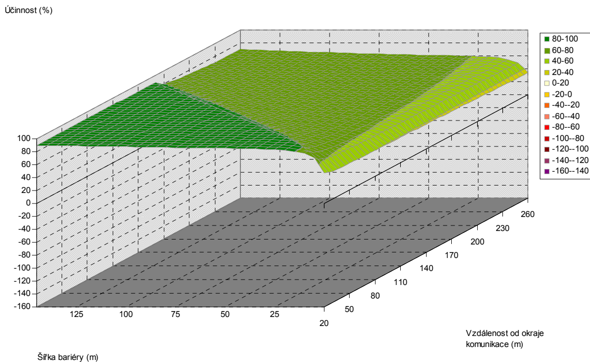
Obr. 5.226. Závislost účinnosti vegetační bariéry na šířce bariéry a vzdálenosti od komunikace, pro výšku bariéry 6 m, jehličnaté dřeviny, PM75, 3 m nad povrchem
