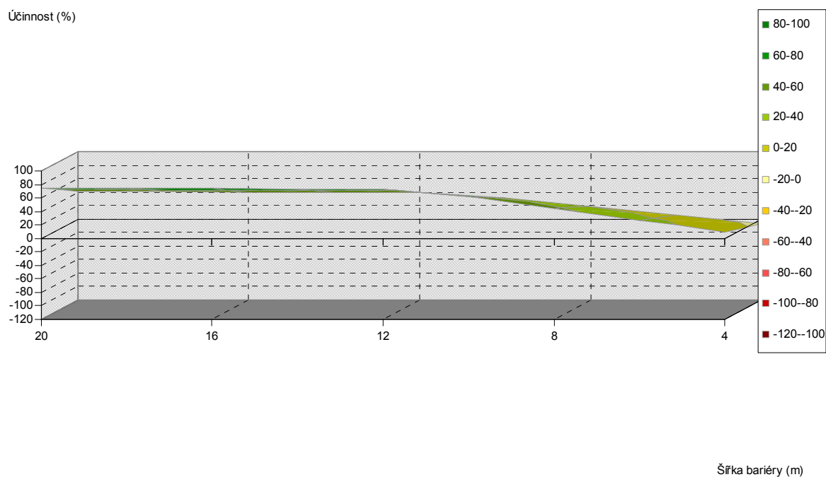
Obr. 5.383. Závislost účinnosti vegetační bariéry na výšce a šířce bariéry, pro vzdálenost od komunikace 20 m, listnaté dřeviny, PM75, 6 m nad povrchem
