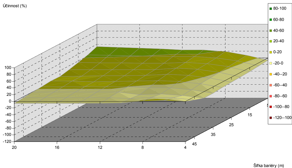
Obr. 5.321. Závislost účinnosti vegetační bariéry na výšce a šířce bariéry, pro vzdálenost od komunikace 60 m, jehličnaté dřeviny, PM10, 6 m nad povrchem
