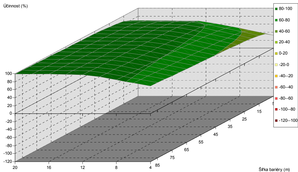
Obr. 5.401. Závislost účinnosti vegetační bariéry na výšce a šířce bariéry, pro vzdálenost od komunikace 100 m, jehličnaté dřeviny, PM75, 6 m nad povrchem
