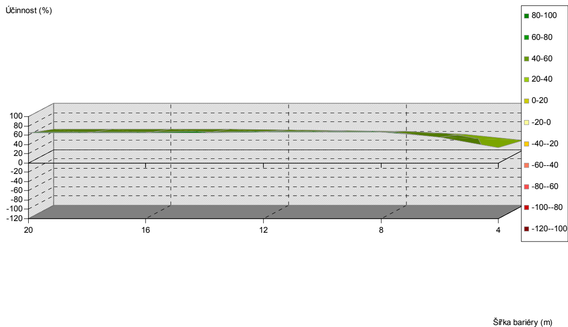
Obr. 5.357. Závislost účinnosti vegetační bariéry na výšce a šířce bariéry, pro vzdálenost od komunikace 20 m, listnaté dřeviny, PM75, 3 m nad povrchem
