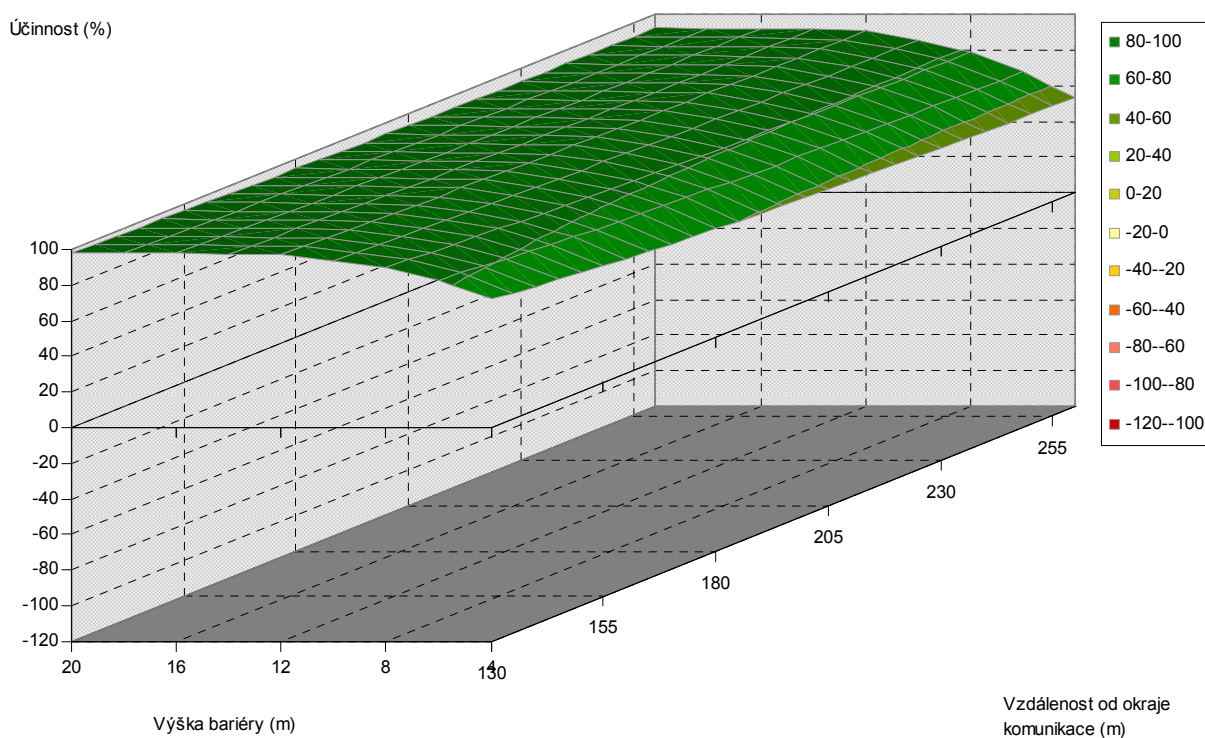
Obr. 5.88. Závislost účinnosti vegetační bariéry na výšce bariéry a vzdálenosti od komunikace, pro šířku bariéry 120 m, jehličnaté dřeviny, PM75, 1,5 m nad povrchem
