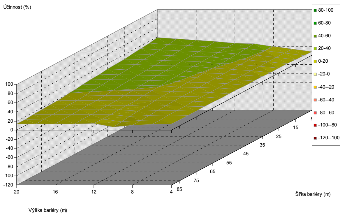
Obr. 5.258. Závislost účinnosti vegetační bariéry na výšce a šířce bariéry, pro vzdálenost od komunikace 100 m, listnaté dřeviny, PM10, 1,5 m nad povrchem
